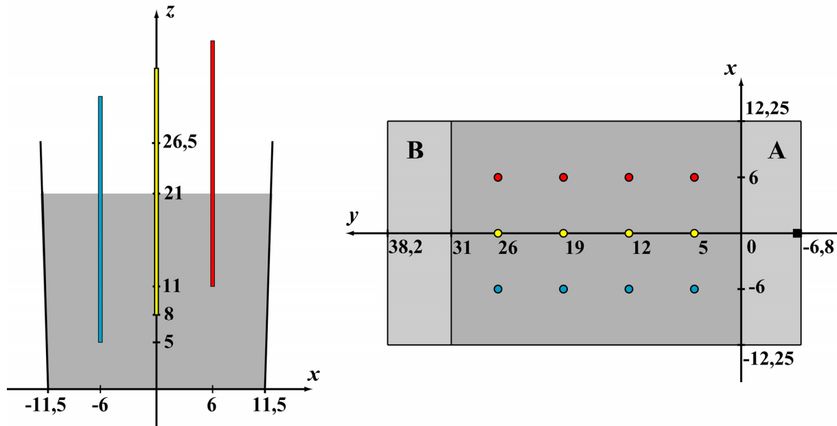
Figure 3.4. Position des électrodes et des réservoirs pour les expériences d'écoulement. Gauche : vue transverse; droite : vue de dessus. Trois séries de quatre électrodes de mesure ( cercles ) sont disposées longitudinalement: la série à x = 6 cm ( rouge ) échantillonne la cote z = 11 cm; la série à x = 0 cm ( jaune ) la cote z = 8 cm; et la série à x = -6 cm ( bleu ) la cote z = 5 cm. L'électrode de référence ( carré ) est située dans le réservoir A (amont), à z = 8,4 cm. Distances en centimètres.
