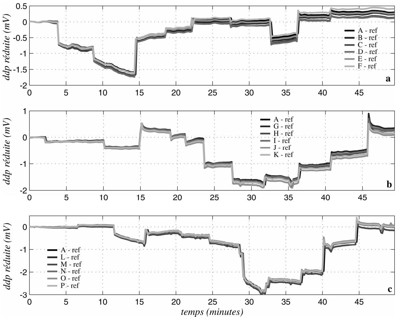
Figure 2.18. Vérification de la similarité des réponses des différentes électrodes. Les électrodes ont été disposées par groupes de six (A, B, C, D, E et F (a); A, G, H, I, J, K (b); A, L, M, N, O, P (c)) dans la cuve remplie de sable et mise en eau courante, sur la ligne y = 15 cm et z = 8 cm (voir figure 2.3), espacées chacune de 2 cm. Une électrode de référence est placée dans le réservoir A. Une tension variable est alors imposée entre les deux réservoirs A et B à l'aide d'un générateur de basse tension stabilisée, créant une différence de potentiel entre la ligne des électrodes, isopotentielle, et la référence. Les différences de potentiel ( ddp ) observées, globalement similaires, confirment la validité des électrodes, les dérivées temporelles linéaires observées, propres à chaque couple d'électrodes, s'expliquant par le fait que l'équilibre entre les électrodes et le milieu n'était pas encore atteint avant le début de chaque expérience.
