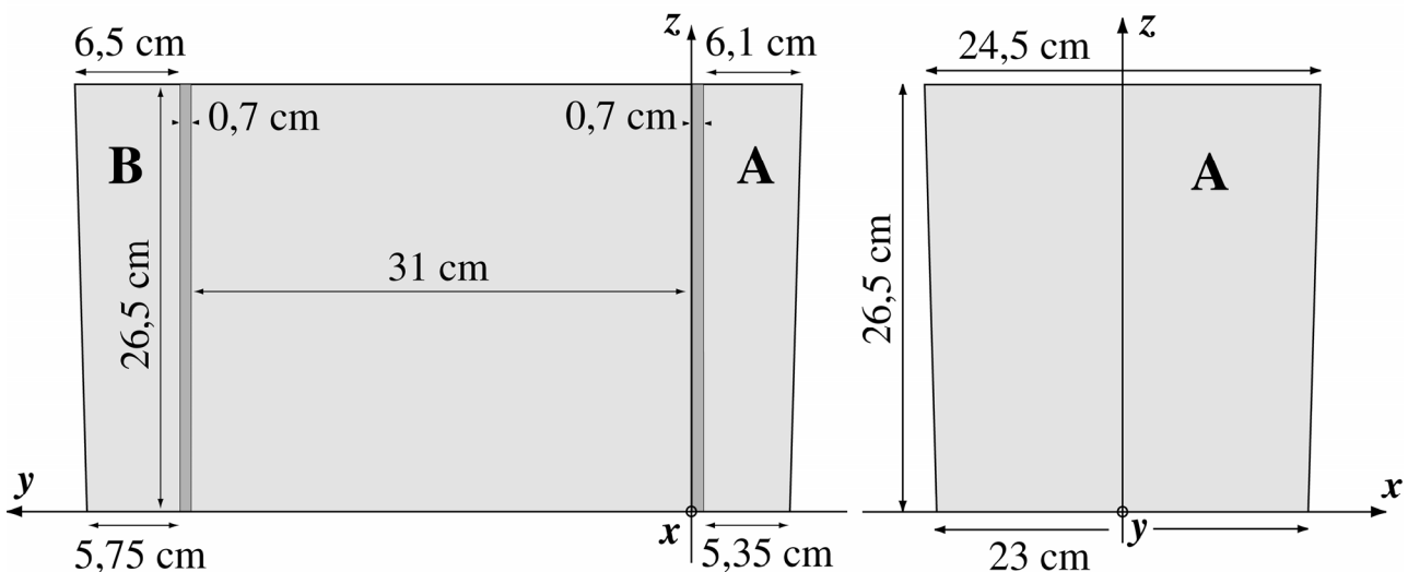
Figure 2.3. Dimensions de la cuve. Gauche : coupe dans la direction d'écoulement; droite : coupe dans la direction transverse. La cuve a été divisée dans le sens de la longueur en trois parties par des plaques de PVC percées. Le sable est placé dans la partie centrale, les deux autres parties A et B formant les réservoirs amont ou aval. Un repère cartésien direct (x,y,z) est associé à la cuve pour repérer les positions des électrodes. Notez que les bords extérieurs de la cuve sont faiblement ouverts vers l'extérieur (angle de 1,62^\circ ). Proportions respectées.
