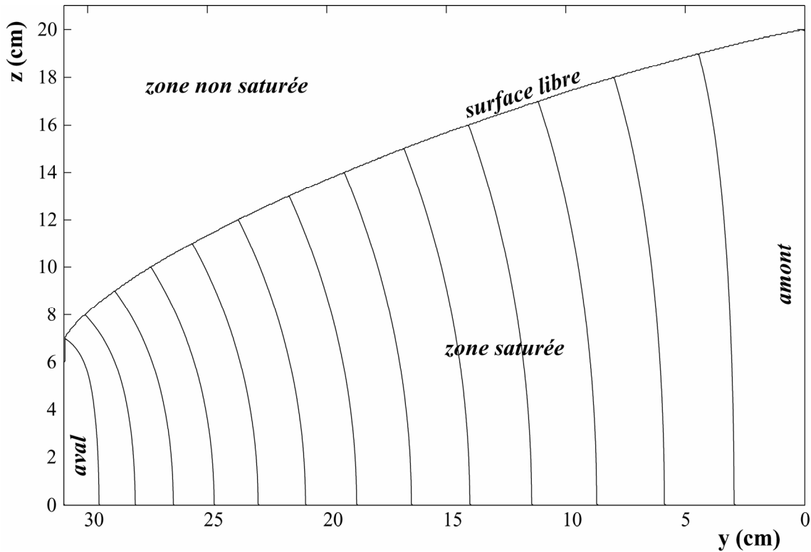
Figure 2.9. Surface libre et lignes isopotentielles pour un niveau amont de 20 cm et un niveau aval de 6 cm. La charge entre deux lignes de contour est de 1 cm. Noter la zone de fuite de 1 cm en y = Y = 31 cm.
