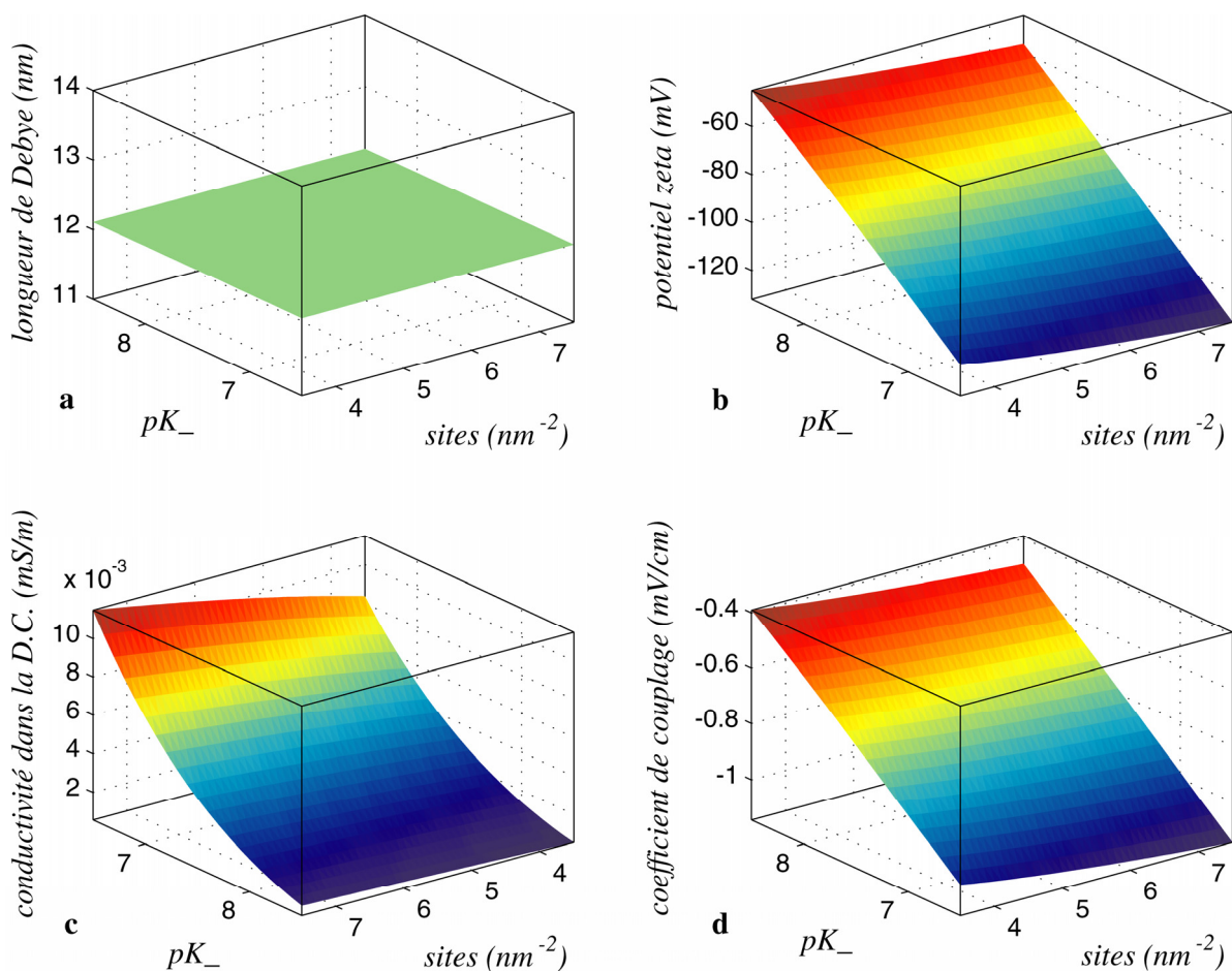
Figure 3.13. Modèle de Revil et Glover appliqué au système quartz 300 \mu\text{m} / solution de NaCl à 8 \text{mS}\cdot\text{m}^{-1} . Paramètres en fonction de la densité de sites et de pK_- pour un pK_{\text{Na}} de 7,1: a: longueur de Debye; b: potentiel \zeta ; c: conductivité de la double couche; d: coefficient de couplage électrocinétique.
