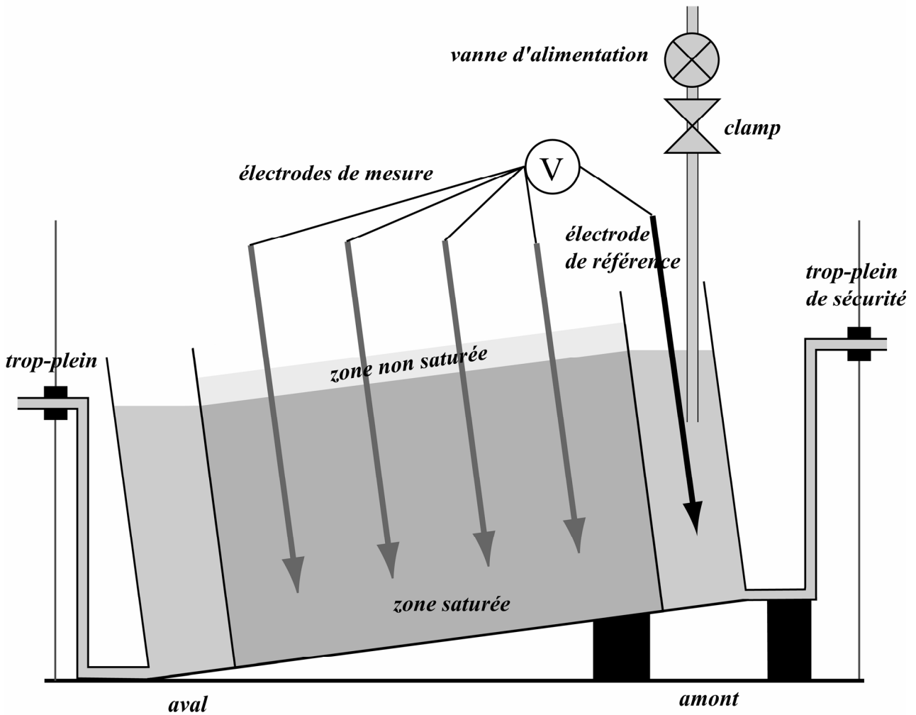
Figure 2.5. Schéma de la cuve en configuration 1D. La cuve est inclinée et les hauteurs d'eau par rapport au fond de la cuve, au niveau des deux limites sable-réservoir, sont maintenues égales, générant ainsi un écoulement unidimensionnel (parallèle à l'axe d'inclinaison). Le débit nécessaire pour maintenir la hauteur amont est obtenu en ajustant le clamp, de façon à ce que le trop-plein de sécurité (amont) ne rejette pas de fluide. Le niveau aval est maintenu en réglant la hauteur du trop-plein. L'électrode de référence est placée, selon les expériences, dans le réservoir amont ou dans le réservoir aval. Notez l'existence d'une zone partiellement saturée entre la surface du sable et la surface libre.
