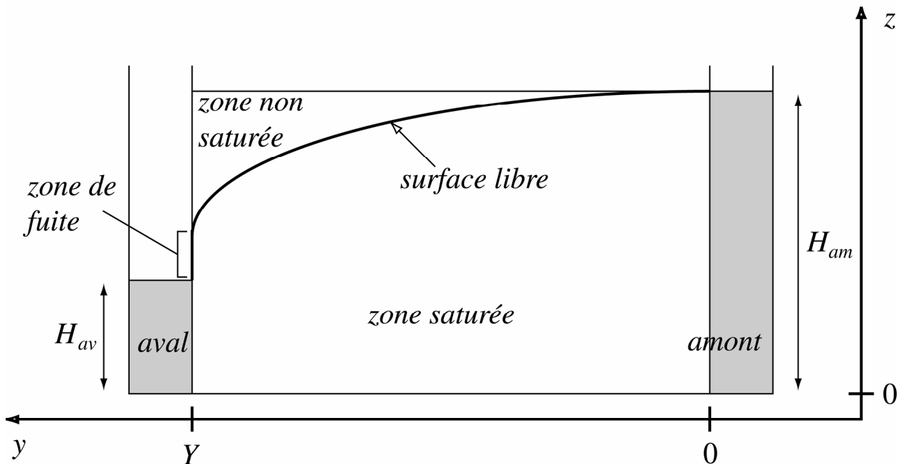
Figure 2.8. Géométrie du problème de l'écoulement 2D. Les trois paramètres du problème sont les niveaux amont et aval, respectivement notés H_{am} et H_{av} , et la longueur de sable Y . La méthode de Baiocchi étend le domaine de résolution de la zone saturée à l'ensemble zone saturée - zone non saturée (en négligeant cependant le stockage dans cette dernière), soit le domaine H_{am} \times Y . Notez l'existence d'une "zone de fuite", d'autant plus importante que le différentiel entre niveaux amont et aval est grand.
