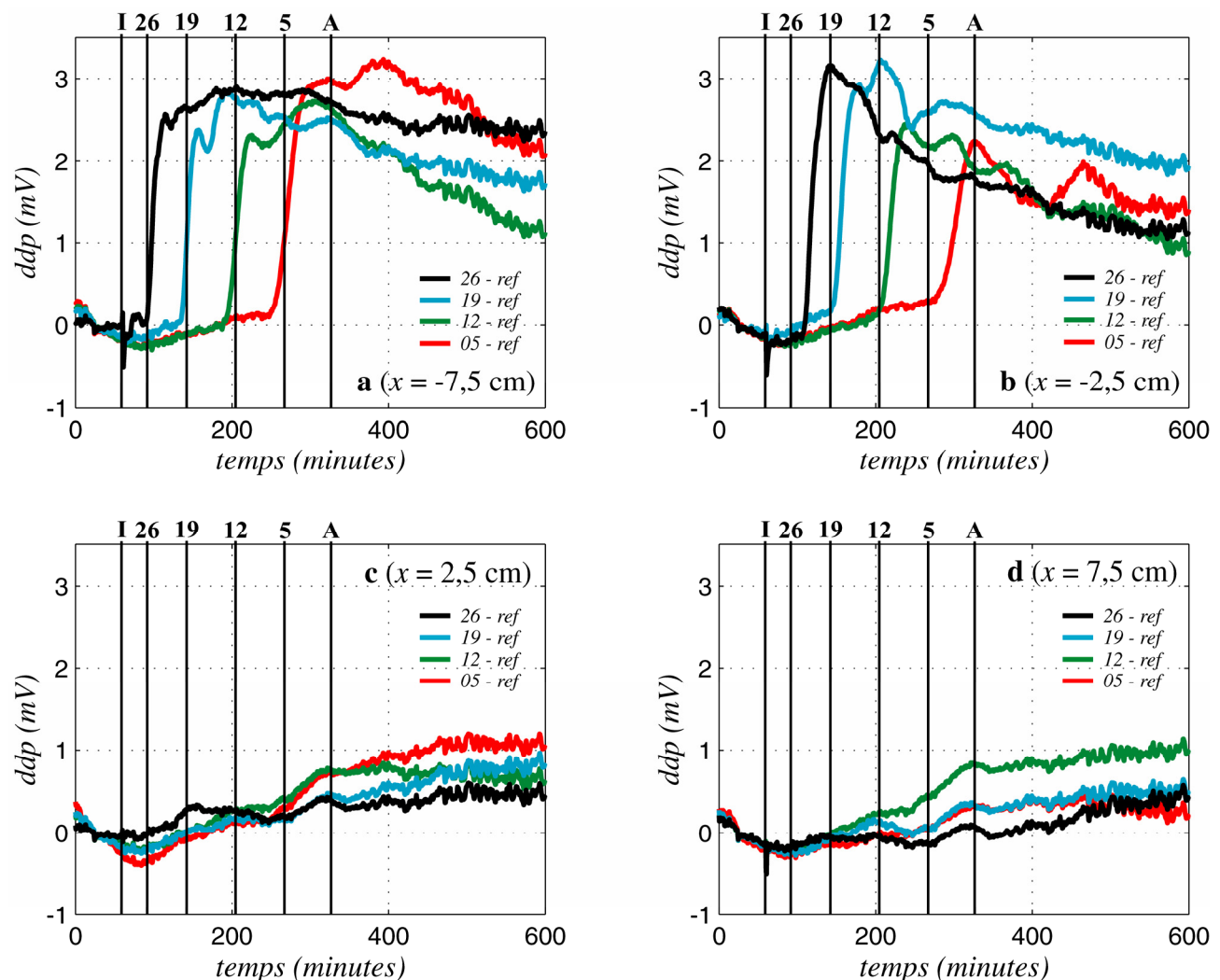
Figure 5.6. Différences de potentiel par rapport à la référence pour la réaction HCl-NaOH, réduites de leur valeur moyenne sur le temps pré-injection. a et b : séries longitudinales dans la zone liée à l'injection d'acide chlorhydrique (liée au réservoir B., x = -7,5 \text{ cm} et x = -2,5 \text{ cm} ); c et d : séries longitudinales dans la zone liée à l'injection de soude (liée au réservoir B., x = 2,5 \text{ cm} et x = 7,5 \text{ cm} ) (voir figure 5.1). Courbes noires: électrodes de mesure à y = 26 \text{ cm} ; bleues: à y = 19 \text{ cm} ; vertes: à y = 12 \text{ cm} ; rouges: à y = 5 \text{ cm} . Barre verticale I: temps d'injection; barres 26, 19, 12, 5: temps de passage théorique du front salin aux électrodes dans l'hypothèse unidimensionnelle à y = 26, 19, 12 et 5 \text{ cm} respectivement; barre A: temps d'arrivée théorique dans le réservoir aval. La forme des courbes permet de conclure à une modification du couplage électrocinétique local en fonction du pH.
