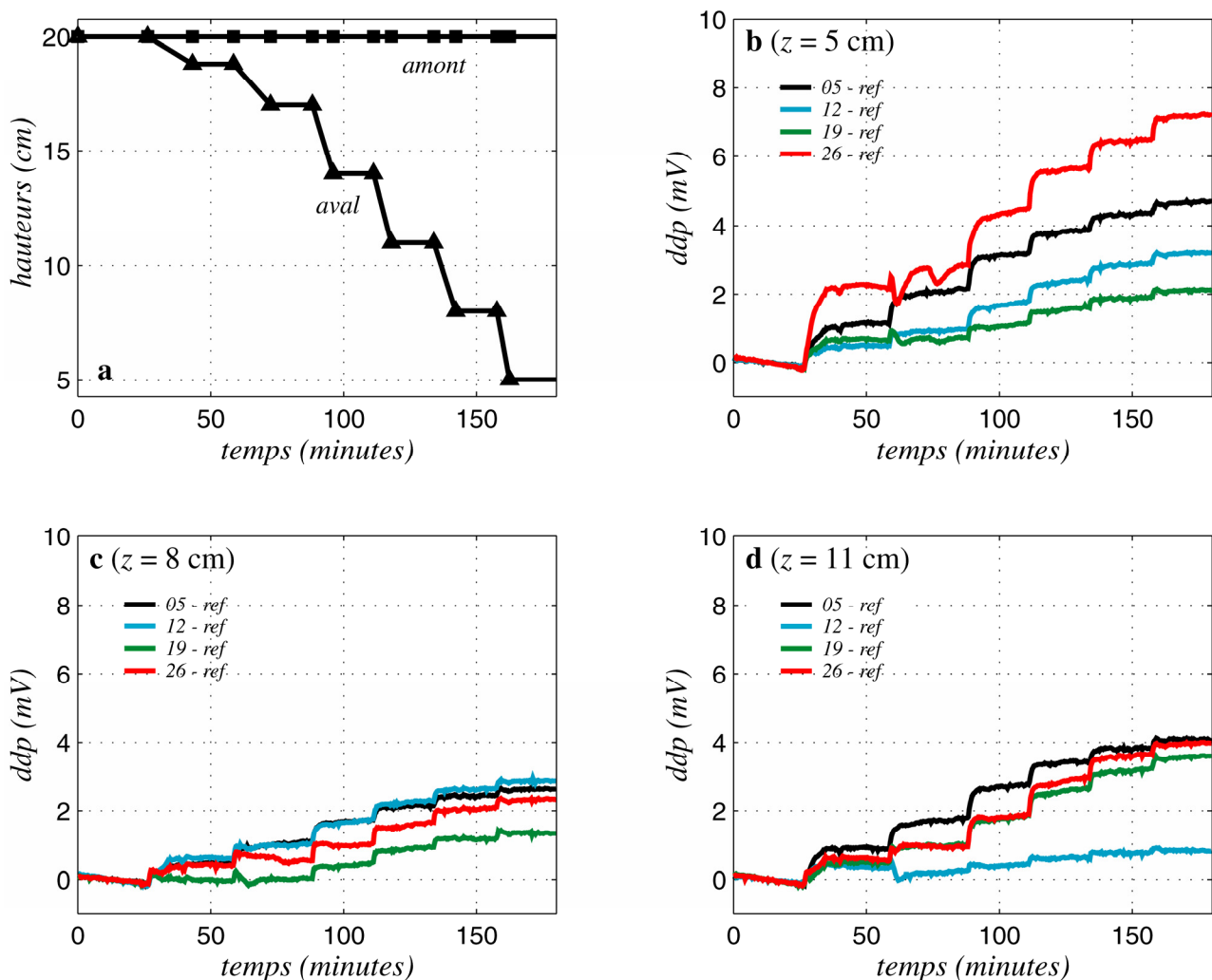
Figure 3.12. Différences de potentiel par rapport à la référence pour une descente aval, eau déionisée. a: évolution des niveaux de fluide dans les réservoirs (les transitions entre paliers intègrent les effets transitoires). b: différences de potentiel (ddp) par rapport à la référence à la cote z = 5 \text{ cm} ; c: ddp à la cote z = 8 \text{ cm} ; d: ddp à la cote z = 11 \text{ cm} . Courbes noires: électrodes à y = 5 \text{ cm} ; bleues: à y = 12 \text{ cm} ; vertes: à y = 19 \text{ cm} ; rouges: à y = 26 \text{ cm} (voir figure 3.4). Le temps de stabilisation des ddp sur les paliers est beaucoup plus long que lors de la montée aval (figure 3.6), conséquence des effets de désaturation.
