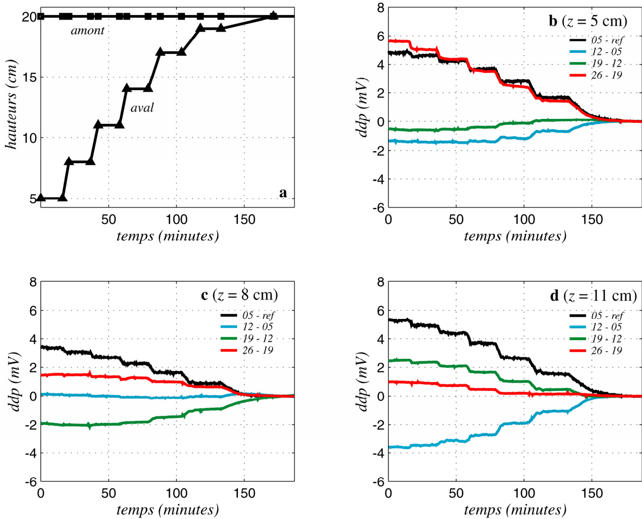
Figure 3.7. Différences de potentiel locales pour une montée aval, eau déionisée. a: évolution des niveaux de fluide dans les réservoirs (les transitions entre paliers intègrent les effets transitoires). b: différences de potentiel (ddp) locales à la cote z = 5 cm; c: ddp à la cote z = 8 cm; d: ddp à la cote z = 11 cm. Courbes noires: différence entre l'électrode à y = 5 cm et la référence; bleues: entre y = 12 cm et y = 5 cm; vertes: entre y = 19 cm et y = 12 cm; rouges: entre y = 26 cm et y = 19 cm (voir figure 3.4). Remarquez l'existence de couplages positifs et l'absence de cohérence entre les trois séries.
