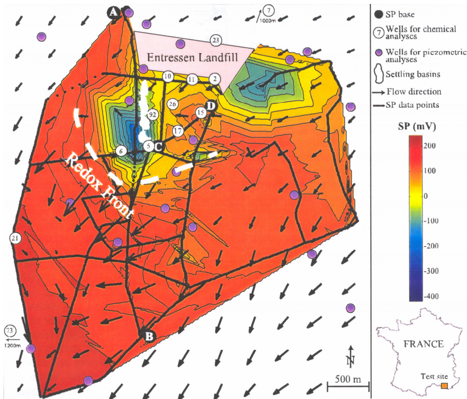
Figure 1.8. Carte de potentiel spontané du site d'Entressen. La zone réduite en aval du dépôt génère une anomalie de PS de -400 mV par rapport à une référence éloignée (en zone oxydée), permettant de déterminer la position du front d'oxydoréduction. Notez la composante électrocinétique (gradient de 200 mV dans le sens opposé à la direction d'écoulement). Carte effectuée sur 2800 points de mesure. Naudet et al., 2003.
