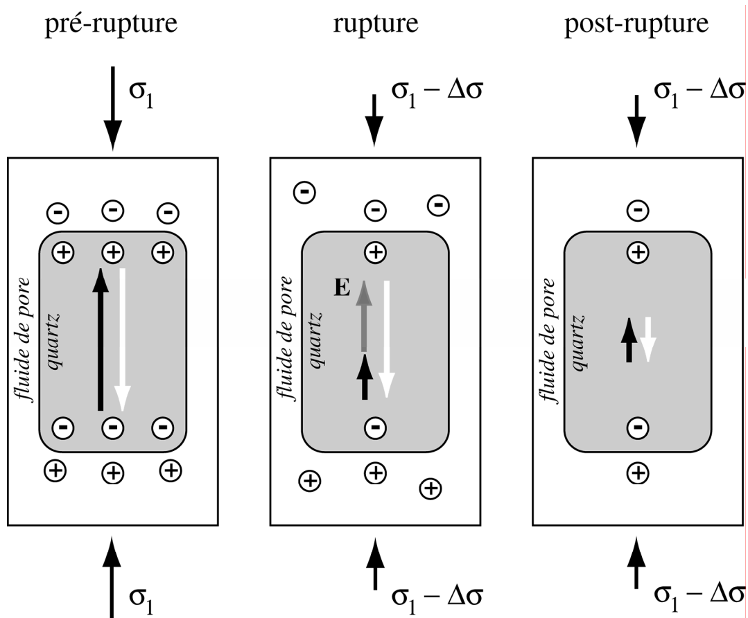
Figure 1.5. Effet piézoélectrique appliqué aux séismes. Avant la rupture, la polarisation des grains de quartz (flèche noire) induite par la contrainte maximale \sigma_1 est compensée par des charges fluides extérieures (flèche blanche). La chute de contrainte associée à la rupture entraîne une dépoliarisation très rapide des grains: la roche reste polarisée tant que la migration des charges extérieures pour assurer la neutralité n'est pas terminée (flèche grise). L'émission d'onde électromagnétique associée à la polarisation de la roche cesse dès que l'état de neutralité électrique est rétabli. D'après Darnet, 2003.
