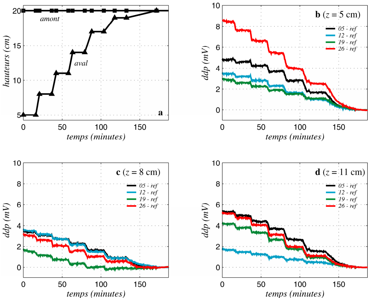
Figure 3.6. Différences de potentiel par rapport à la référence pour une montée aval, eau déionisée. a: évolution des niveaux de fluide dans les réservoirs (les transitions entre paliers intègrent les effets transitoires). b: différences de potentiel (ddp) par rapport à la référence à la cote z = 5 cm; c: ddp à la cote z = 8 cm; d: ddp à la cote z = 11 cm. Courbes noires: électrodes à y = 5 cm; bleues: à y = 12 cm; vertes: à y = 19 cm; rouges: à y = 26 cm (voir figure 3.4). Si les ddp sont positives, remarquez le comportement inattendu selon lequel la ddp n'augmente pas forcément avec la distance.
