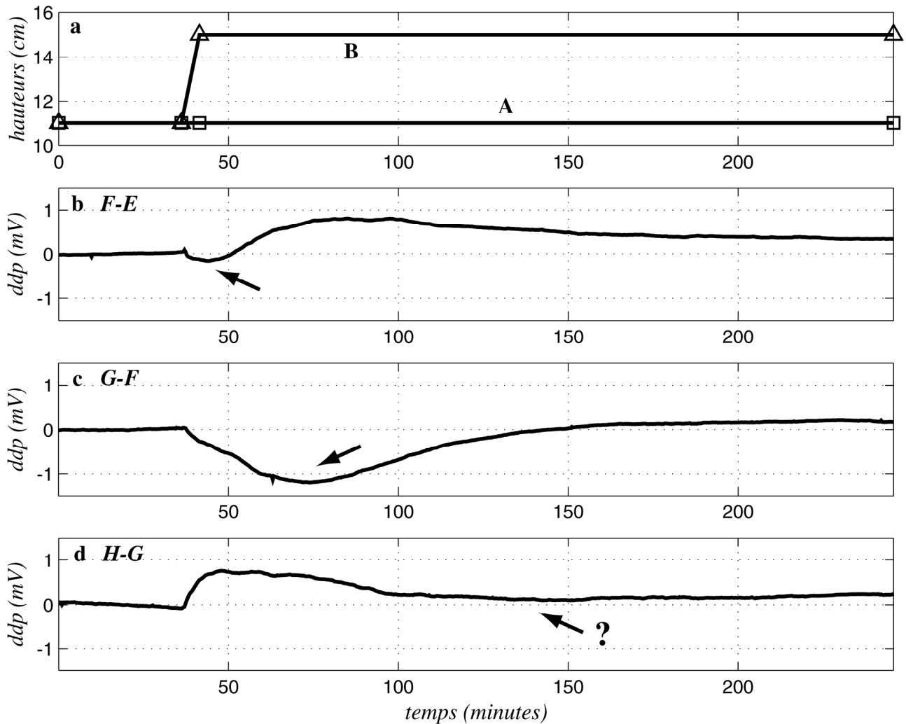
Figure 3.2. Test de vérification de la symétrie: montée du réservoir B. Les niveaux d'eau initiaux dans les réservoirs A et B sont à 11 cm; le niveau d'eau dans le réservoir B est augmenté brusquement à 15 cm (a). b, c, d: différences de potentiel (ddp) correspondantes, réduites de leur valeur initiale. Dès la génération de l'écoulement, les ddp sont modifiées, mais mettent plusieurs heures à atteindre une valeur stable, supérieure au zéro. Les flèches signalent l'éventuelle propagation d'un "front d'onde".
