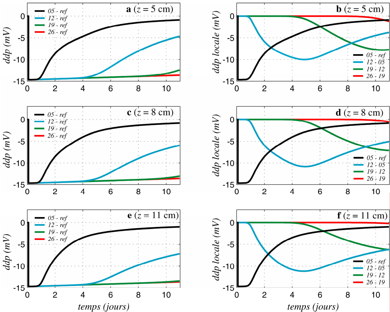
Figure 4.8. Modélisation 2D de la diffusion, D^* = D_m / \tau Différences de potentiel de jonction (ddp) par rapport à la référence, à la cote z = 5 cm (a), z = 8 cm (c) et z = 11 cm (e); courbes noires: électrodes de mesure à y = 5 cm; bleues: à y = 12 cm; vertes: à y = 19 cm; rouges: à y = 26 cm. Ddp locales, à la cote z = 5 cm (b), z = 8 cm (d) et z = 11 cm (f); courbes noires: ddp de jonction entre les électrodes à y = 5 cm et la référence; bleues: à y = 12 cm et y = 5 cm; vertes: à y = 19 cm et y = 12 cm; rouges: à y = 26 cm et y = 19 cm (voir figure 3.4).
