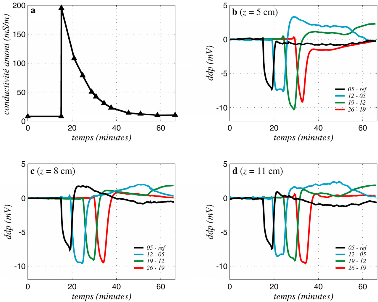
Figure 4.15. Différences de potentiel locales pour l'advection 2D de NaCl, réduites de leur valeur moyenne sur le temps pré-injection. a: conductivité du réservoir amont. b: ddp à la cote z = 5 cm; c: à z = 8 cm; d: à z = 11 cm. Courbes noires: ddp entre les électrodes à y = 5 cm et la référence; bleues: à y = 12 cm et y = 5 cm; vertes: à y = 19 cm et y = 12 cm rouges: à y = 26 cm et y = 19 cm (voir figure 3.4). Le comportement des ddp est très semblable au comportement advectif 1D (figure 4.11).
