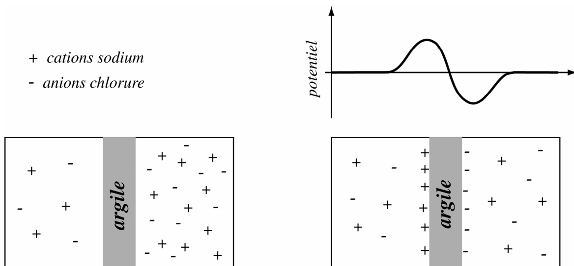
Figure 1.2. Potentiel d'exclusion membranaire dans le cas des argiles. Gauche : à l'instant initial, un différentiel de concentration existe de part et d'autre de la membrane argileuse. Droite : lors de la diffusion à travers l'argile, les ions négatifs (de même signe que la charge de surface des minéraux argileux) restent piégés, créant un déséquilibre de charge et donc une anomalie de potentiel.
