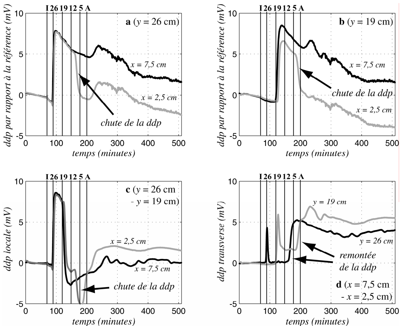
Figure 5.19. Réaction \text{KMnO}_4\text{-FeCl}_2 : différences de potentiel dans la zone x > 0 et y \geq 19 cm. Ddp entre électrodes et référence en y = 26 cm (a) et y = 19 cm (b) et ddp locales y = 26 cm – y = 19 cm (c), dans la solution de \text{FeCl}_2 ( x = 7,5 cm) et à la limite du front de réaction ( x = 2,5 cm). d: ddp transverses entre solution de \text{FeCl}_2 pur et zone limite (i.e., x = 7,5 cm – x = 2,5 cm) en y = 26 cm et y = 19 cm.
