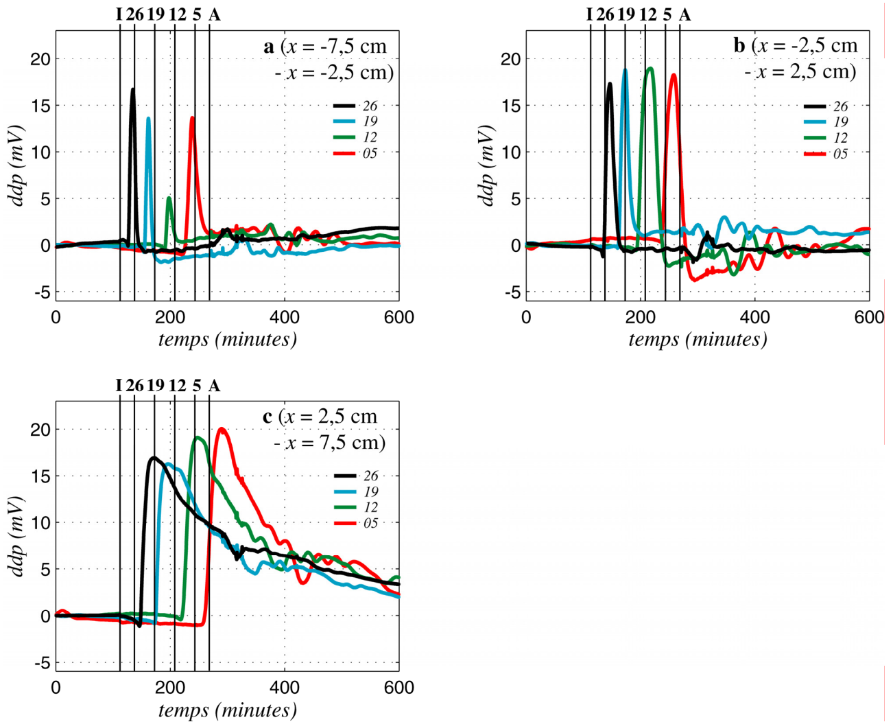
Figure 5.4. Différences de potentiel locales transverses pour l'expérience de contrôle , réduites de leur valeur moyenne sur le temps pré-injection. a : différences transverses dans la zone liée au réservoir B_- (injection de sel) ( x = -7,5 \text{ cm} - x = -2,5 \text{ cm} ); b : différences transverses au travers du plan médian entre les deux zones ( x = -2,5 \text{ cm} - x = 2,5 \text{ cm} ); c : différences transverses dans la zone liée au réservoir B_+ ( x = 2,5 \text{ cm} - x = 7,5 \text{ cm} ) (voir figure 5.1). Courbes noires: électrodes à y = 26 \text{ cm} ; bleues: à y = 19 \text{ cm} ; vertes: à y = 12 \text{ cm} ; rouges: à y = 5 \text{ cm} . Barre verticale I: temps d'injection; barres 26, 19, 12, 5: temps de passage théorique du front salin aux électrodes dans l'hypothèse unidimensionnelle à y = 26, 19, 12 et 5 \text{ cm} respectivement; barre A: temps d'arrivée théorique dans le réservoir aval. La largeur des pics augmente avec la distance à la zone liée au réservoir B_- , ce qui traduit la diminution de la vitesse de progression transverse avec la distance.
