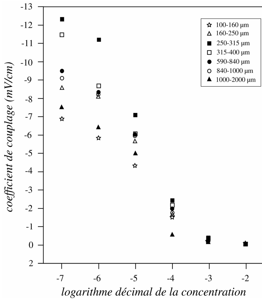
Figure 1.22. Coefficient de couplage électrocinétique du sable de Moskva, en fonction de la concentration en NaCl, pour différentes tailles de grain. Données de Ogilvy et al., 1969.
