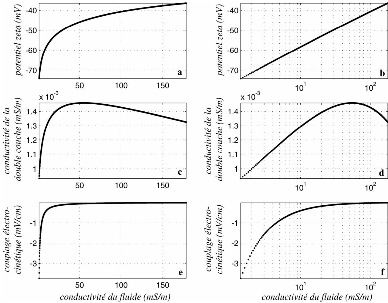
Figure 4.18. Paramètres électrocinétiques calculés pour l'advection 1D de NaCl , selon le modèle de Revil et Glover adapté (section 3.4.1). Evolution du potentiel \zeta (a, b), de la conductivité de la double couche (c, d) et du coefficient de couplage électrocinétique (e, f) en fonction de la conductivité du fluide. Les paramètres d'entrée utilisés sont \Gamma_S = 3 \text{ nm}^{-2} , pK_- = 7,1 et pK_{Na} = 8 .
