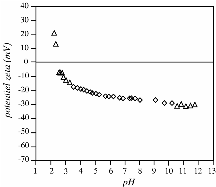
Figure 1.25. Potentiel \zeta du grès de Fontainebleau broyé à 150 \mu\text{m} , en fonction du pH (solution de NaCl à 10 mS.m -1 ). D'après Lorne et al., 1999a.
