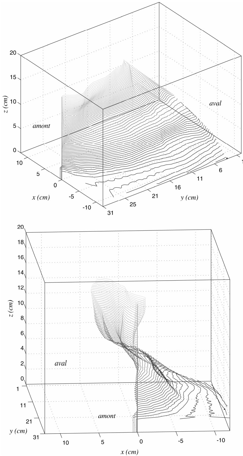
Figure 5.18. Reconstruction de la zone limite entre zone de réaction et \text{KMnO}_4 pour l'expérience préliminaire \text{KMnO}_4\text{-FeCl}_2 . L'incurvation des fronts résulte du contraste de densité entre le permanganate de potassium et le chlorure de fer II: plus dense, ce dernier a coulé vers le fond de la cuve.
