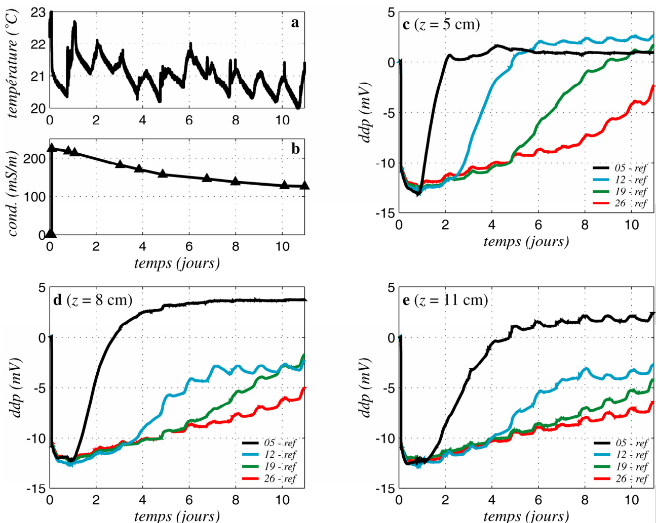
Figure 4.1. Différences de potentiel (ddp) par rapport à la référence pour l'expérience de diffusion de NaCl, réduites de leur valeur moyenne sur le temps pré-injection. a: température ambiante; b: conductivité électrique du réservoir amont; c: ddp à la cote z = 5 \text{ cm} ; d: à z = 8 \text{ cm} ; e: à z = 11 \text{ cm} . Courbes noires: électrodes de mesure à y = 5 \text{ cm} ; bleues: à y = 12 \text{ cm} ; vertes: à y = 19 \text{ cm} ; rouges: à y = 26 \text{ cm} (voir figure 3.4). Le front salin diffuse plus rapidement au fond du bac (c).
