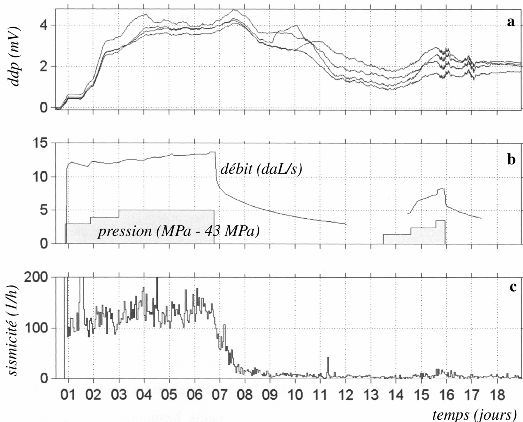
Figure 1.7. Expérience de Soultz-sous-Forêts, injection de juin 2000. a: différences de potentiel (ddp) enregistrées en surface à 500 m du puits d'injection (filtrées par basse-pass 24h); b: pression d'injection et débit d'injection en tête de puits; c: sismicité induite. La sismicité induite est directement corrélée avec le débit d'injection, traduisant la stimulation des fractures. Les ddp atteignent un plateau lorsque les écoulements sont stabilisés, puis retournent à zéro plus lentement que l'écoulement, ce qui implique l'action d'autres sources qu'électrocinétiques. D'après Darnet, 2003.
