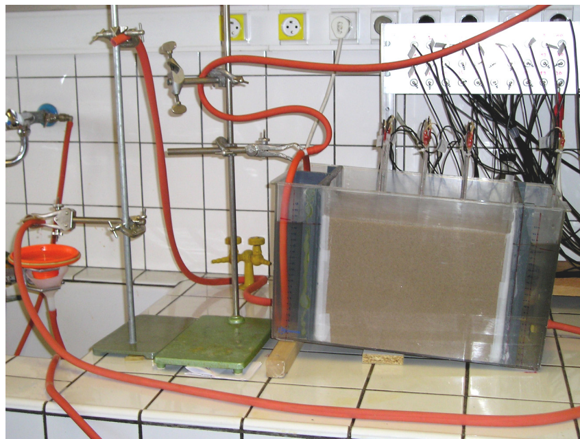
Figure 2.4. Cuve en configuration 1D. La cuve est inclinée et les hauteurs d'eau par rapport au fond de la cuve, au niveau des deux limites sable-réservoir, sont maintenues égales, générant ainsi un écoulement unidimensionnel (parallèle à l'axe d'inclinaison). Notez que la séparation en deux parties du réservoir amont, dans le sens de la longueur, correspond à la configuration pour les expériences avec réaction.
