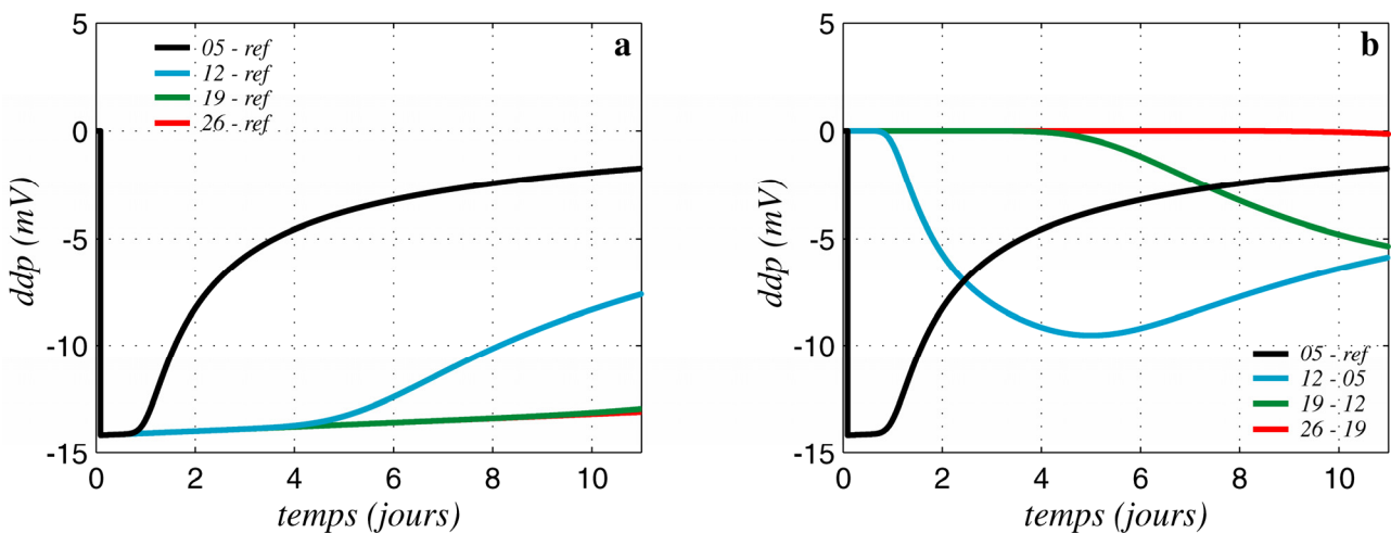
Figure 4.3. Modélisation 1D de la diffusion, D^* = D_m / \tau . a: différences de potentiel (ddp) par rapport à la référence; courbe noire: électrode de mesure à y = 5 cm; bleue: à y = 12 cm; verte: à y = 19 cm; rouge: à y = 26 cm. b: ddp locales; courbe noire: ddp entre l'électrode à y = 5 cm et la référence; bleue: à y = 12 cm et y = 5 cm; verte: à y = 19 cm et y = 12 cm; rouge: à y = 26 cm et y = 19 cm (voir figure 3.4).
