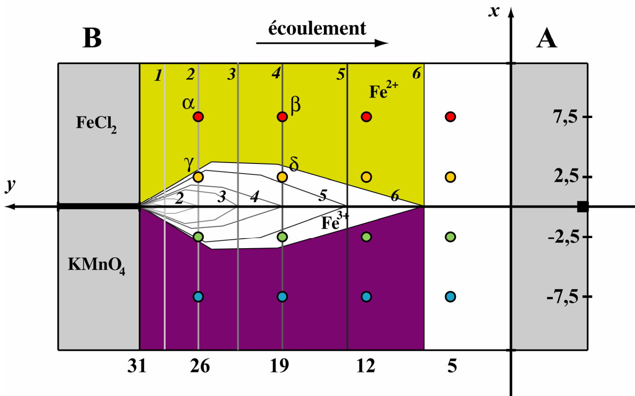
Figure 5.20. Modèle de progression des fronts et de la zone de mélange. Vert-jaune: zone de \text{FeCl}_2 (réduite pour le fer); violet: zone de la solution de \text{KMnO}_4 ; blanc: zone de réaction, oxydée pour le fer. La zone de réaction a une forme de double chevron, dont l'ouverture augmente avec le temps. Explications dans le texte.
