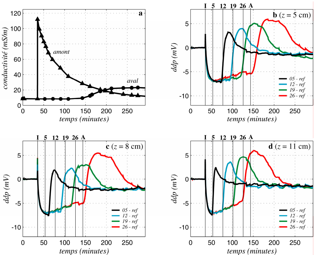
Figure 4.12. Différences de potentiel (ddp) par rapport à la référence pour l'advection 1D de KCl, réduites de leur valeur moyenne sur le temps pré-injection. a: conductivité du réservoir amont ( triangles ) et du réservoir aval ( cercles ). b: ddp à la cote z = 5 cm; c: à z = 8 cm; d: à z = 11 cm. Courbes noires: électrodes de mesure à y = 5 cm; bleues: à y = 12 cm; vertes: à y = 19 cm; rouges: à y = 26 cm (voir figure 3.4). Barre verticale I: temps d'injection; barres 5, 12, 19, 26: temps de passage théorique du front salin aux électrodes à y = 5, 12, 19 et 26 cm respectivement; barre A: temps d'arrivée théorique dans le réservoir aval. Les ddp chutent dès la mise en place du front, puis croissent brusquement, changent de polarité à l'arrivée du front à l'électrode de mesure, et retournent à zéro. Notez la forte amplitude et la forme du signal post-changement de polarité, très différentes du comportement du NaCl (figure 4.10).
