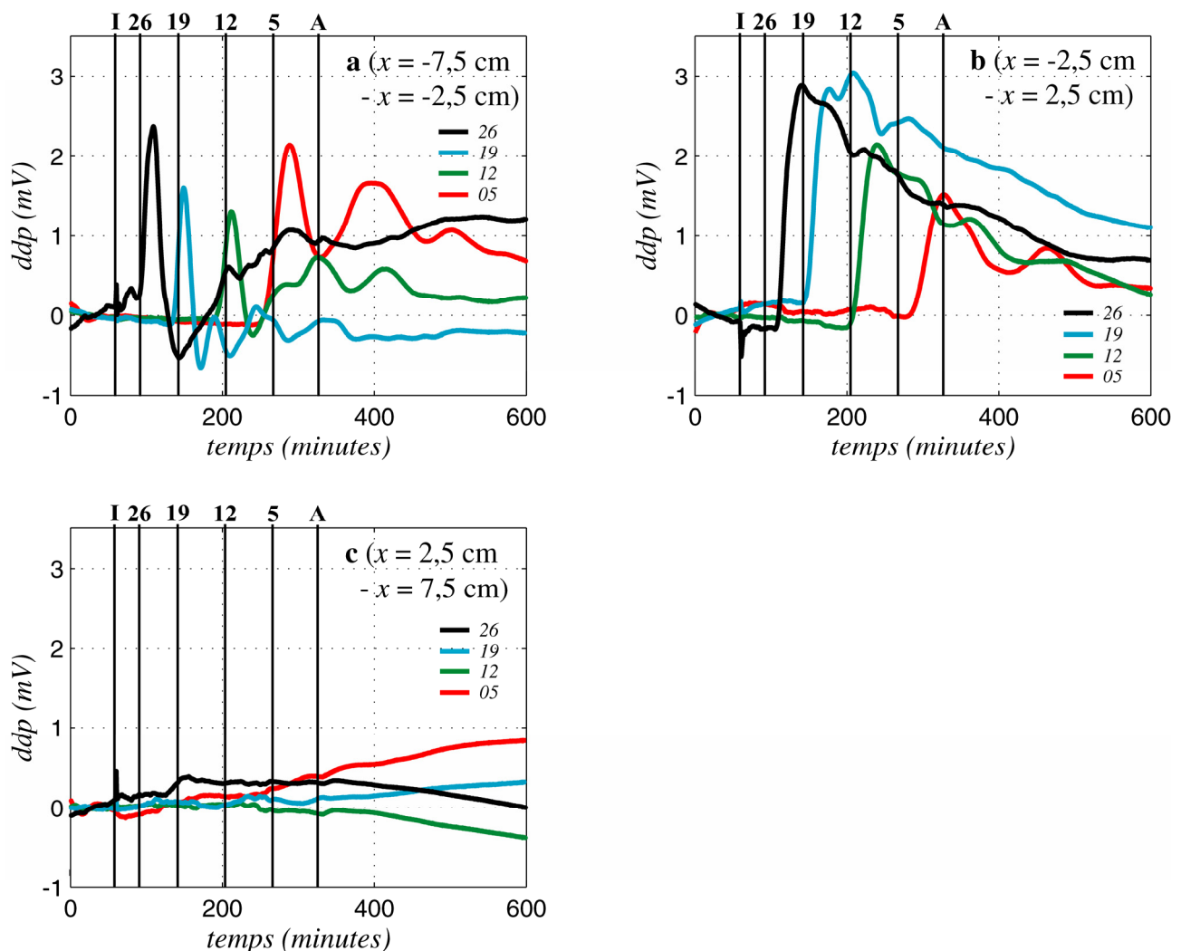
Figure 5.8. Différences de potentiel locales transverses pour la réaction HCl-NaOH , réduites de leur valeur moyenne sur le temps pré-injection. a : différences transverses dans la zone liée à l'injection d'acide chlorhydrique (liée au réservoir B - , x = -7,5 cm – x = -2,5 cm); b : différences transverses au travers du plan médian ( x = -2,5 cm – x = 2,5 cm); c : différences transverses dans la zone liée à l'injection de soude (liée au réservoir B + , x = 2,5 cm – x = 7,5 cm) (voir figure 5.1). Courbes noires: électrodes à y = 26 cm; bleues: à y = 19 cm; vertes: à y = 12 cm; rouges: à y = 5 cm. Barre verticale I: temps d'injection; barres 26, 19, 12, 5: temps de passage théorique du front salin aux électrodes dans l'hypothèse unidimensionnelle à y = 26, 19, 12 et 5 cm respectivement; barre A: temps d'arrivée théorique dans le réservoir aval.
