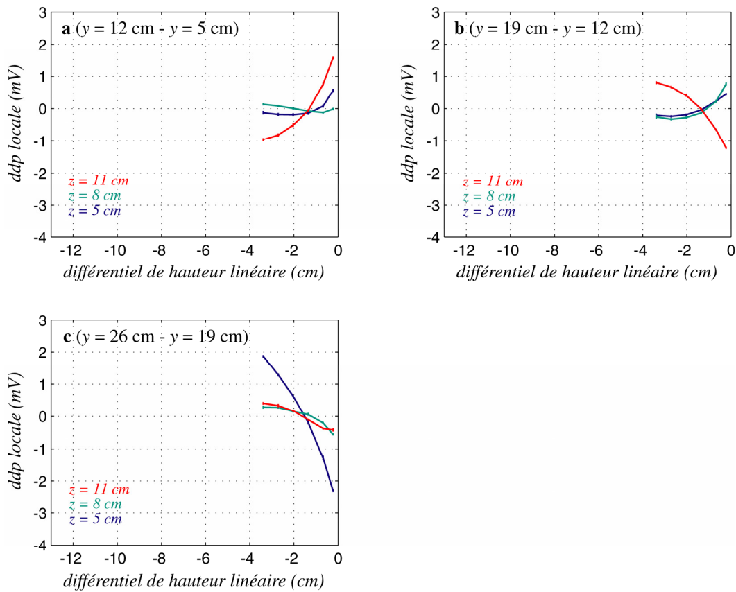
Figure 3.9. ddp sur les paliers (réduites de leur moyenne) en fonction de la différence de niveau entre les réservoirs A et B interpolée linéairement. Données de la figure 3.7. Cf texte.
