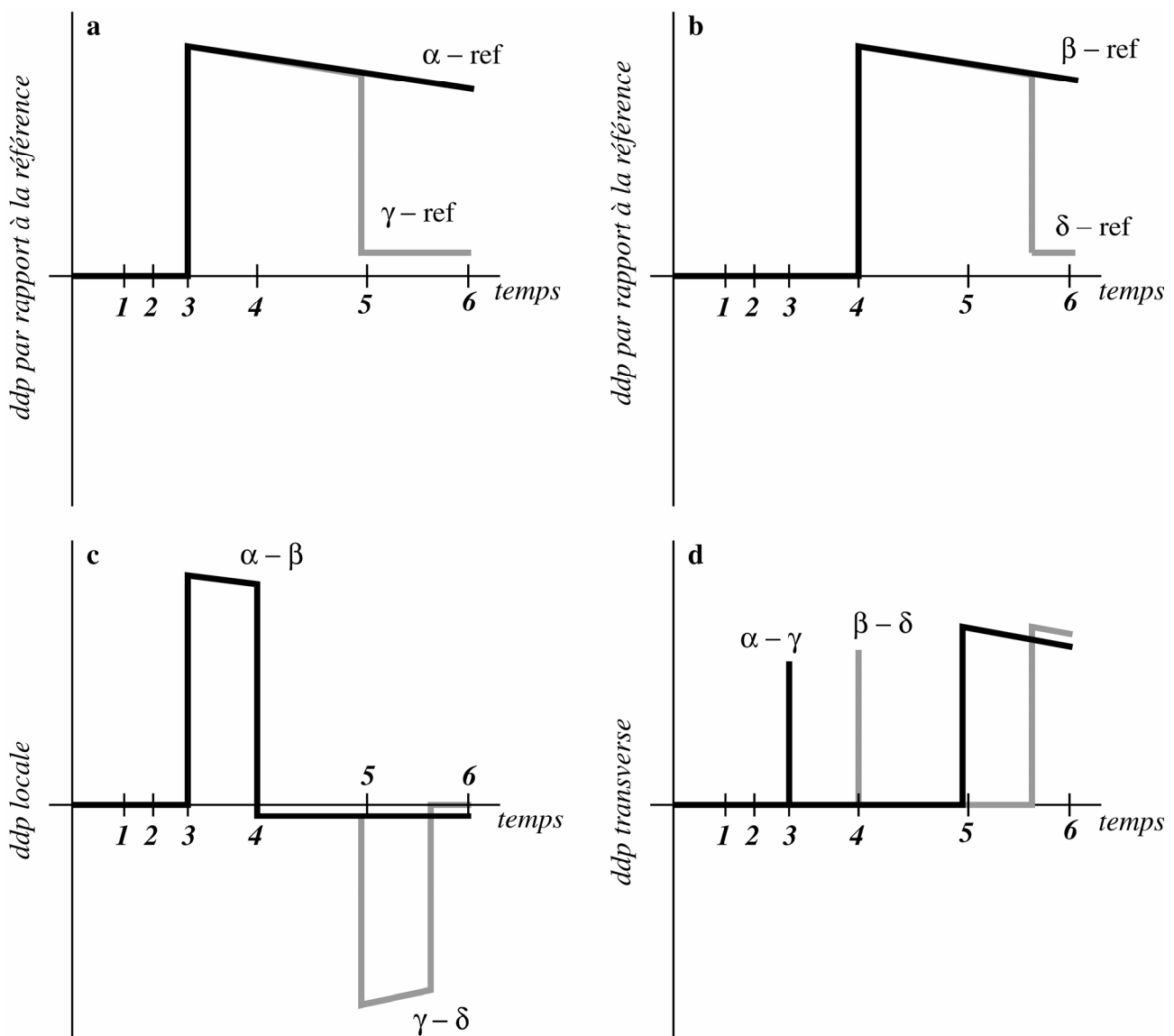
Figure 5.21. Evolution schématique des différences de potentiel sur les électrodes \alpha , \beta , \gamma et \delta , en fonction du modèle d'évolution des fronts et de la zone de mélange présenté sur la figure 5.20. a , b : ddp par rapport à la référence, c : ddp locales; d : ddp transverses. La forme des courbes explique relativement bien les données de la figure 5.19. Explications dans le texte.
