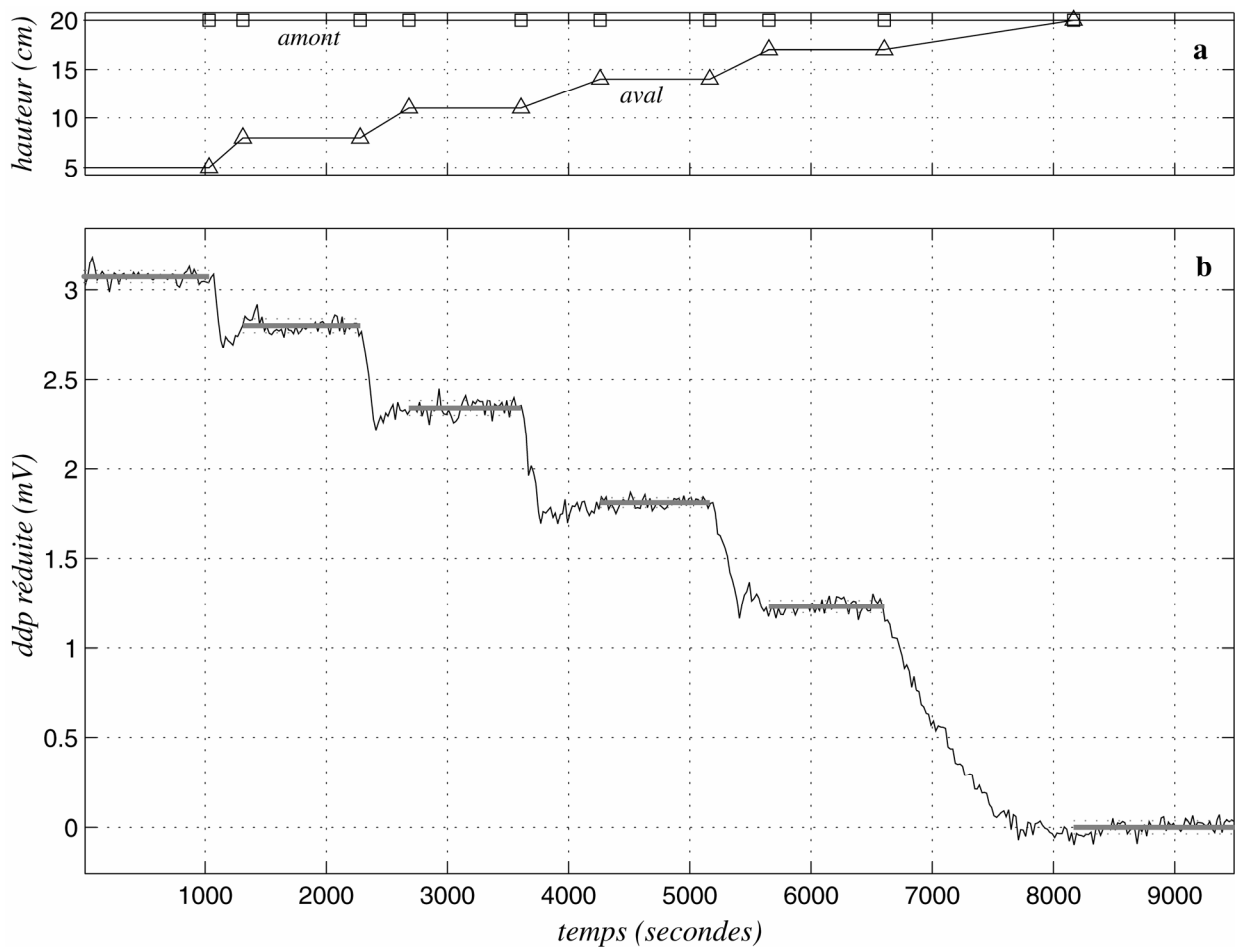
Figure 3.5. Exemple de calcul des valeurs de différence de potentiel (ddp) sur les paliers. a: le niveau du réservoir amont (A) est maintenu à 20 cm, celui du réservoir aval (B), initialement à 5 cm, est augmenté par pas de 3 cm (les transitions entre paliers intègrent les effets transitoires). b: ddp correspondante (noir) entre une électrode de mesure et la référence. La valeur de ddp \Delta V associée à chaque palier hydraulique est prise égale à la moyenne de la ddp stabilisée (gris). La ddp moyenne sur le palier correspondant à l'écoulement nul sert à fixer le zéro.
