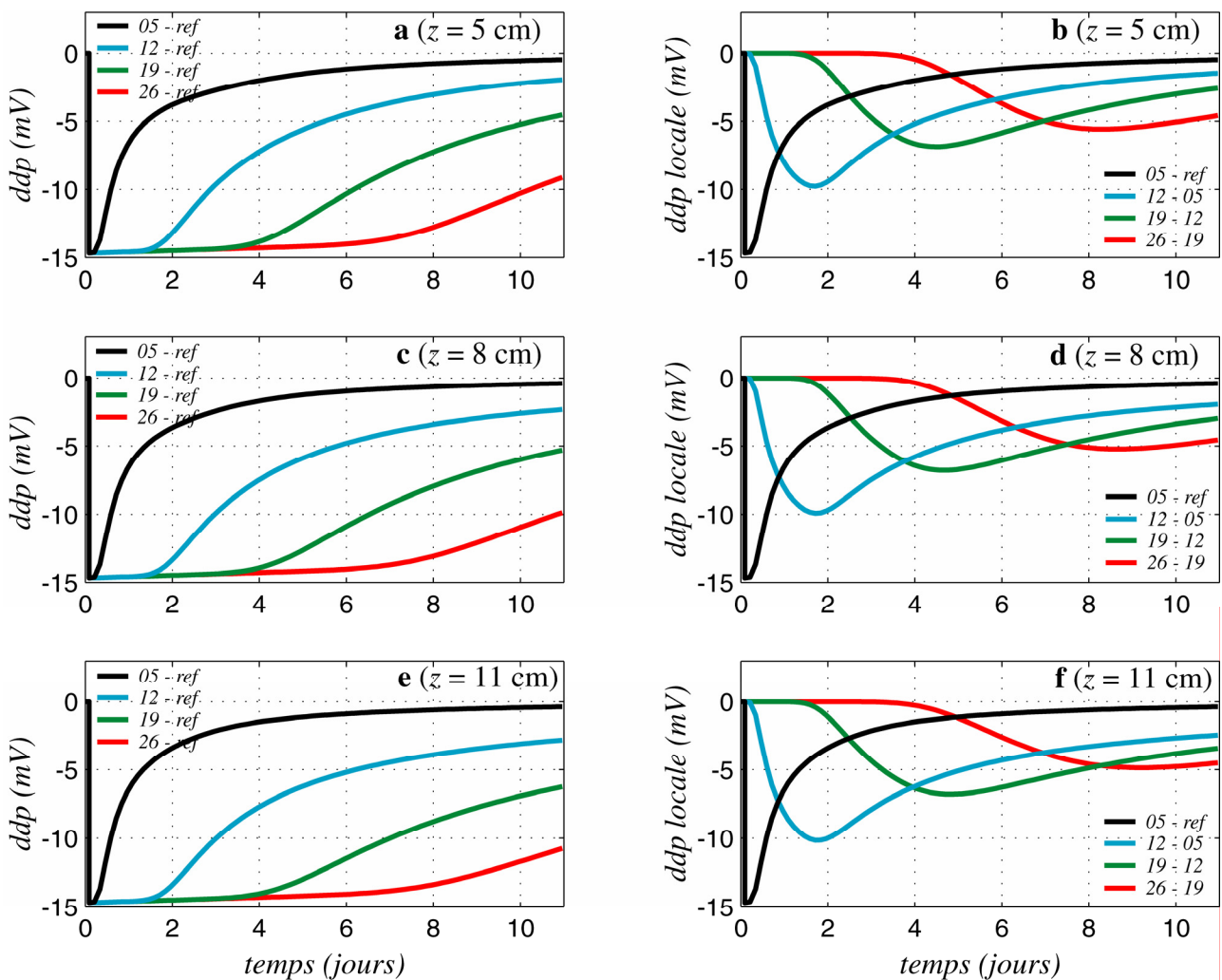
Figure 4.9. Modélisation 2D de la diffusion, D^* = 2 \cdot D_m Différences de potentiel de jonction (ddp) par rapport à la référence, à la cote z = 5 cm (a), z = 8 cm (c) et z = 11 cm (e); courbes noires: électrodes de mesure à y = 5 cm; bleues: à y = 12 cm; vertes: à y = 19 cm; rouges: à y = 26 cm. Ddp locales, à la cote z = 5 cm (b), z = 8 cm (d) et z = 11 cm (f); courbes noires: ddp de jonction entre les électrodes à y = 5 cm et la référence; bleues: à y = 12 cm et y = 5 cm; vertes: à y = 19 cm et y = 12 cm; rouges: à y = 26 cm et y = 19 cm (voir figure 3.4).
