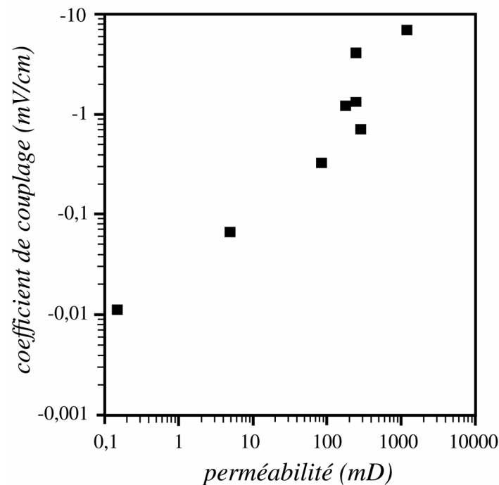
Figure 1.20. Coefficient de couplage électrocinétique du grès non broyés de Fontainebleau entier, en fonction de la perméabilité (échantillons entiers, eau distillée à 1 \text{ mS.m}^{-1} et \text{pH} = 5 ). D'après Jouniaux et Pozzi, 1995a.
