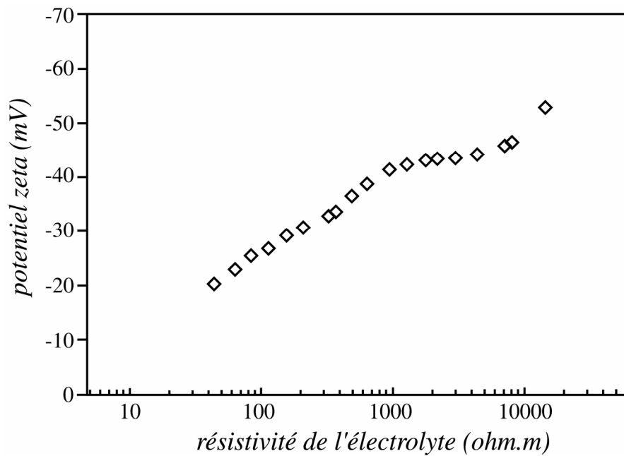
Figure 1.23. Potentiel \zeta du grès de Fontainebleau broyé à 150 \mu\text{m} , en fonction de la résistivité de l'électrolyte (solutions de KCl à pH = 5,7). D'après Lorne et al., 1999a.
