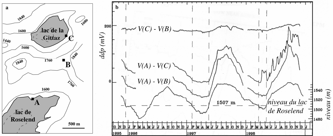
Figure 1.6. Expérience de Sur-Frêtes. a: situation géographique. b: variation des différences de potentiel (ddp) entre les points A, B et C, et variation du niveau du lac de Roselend (la ligne 1507 m indique le niveau du lac en dessous duquel la réponse des électrodes est fortement réduite). Les variations des ddp sur les deux dipôles dans l'axe Gittaz-Roselend sont fortement corrélées avec les variations du niveau du lac de Roselend. Les changements d'écoulements souterrains et de contraintes induits par les variations de niveau d'eau expliquent cette réponse électrique corrélée. D'après Trique et al., 2002.
