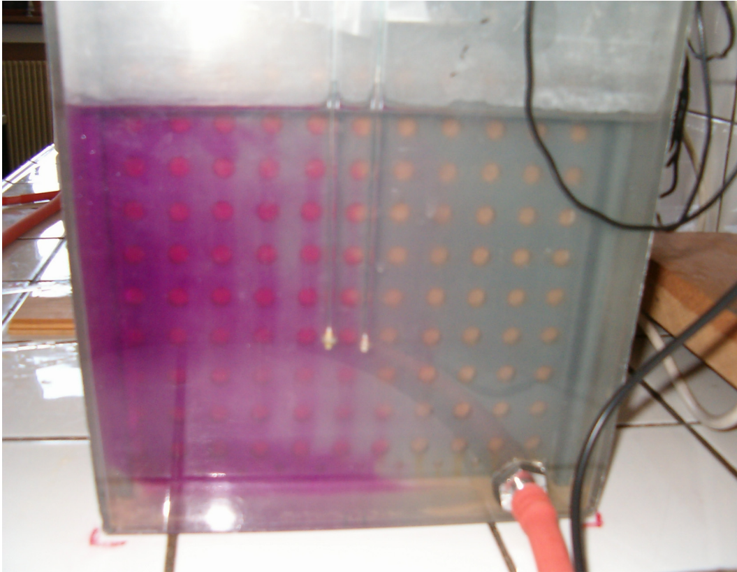
Figure 5.10. Réaction \text{KMnO}_4\text{-FeCl}_2 : sortie des réactifs, vue de face. Vue de face du réservoir aval peu après l'arrivée des réactifs. Violet : permanganate de potassium; incolor : chlorure de fer II. La zone de contact est localisée suivant le plan médian vertical longitudinal.
