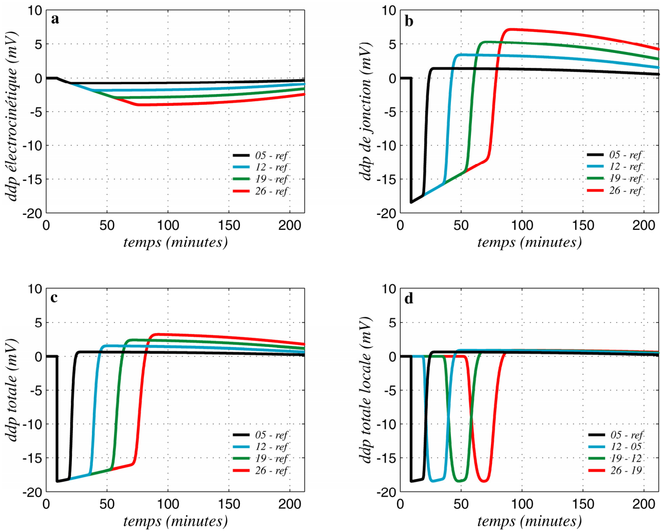
Figure 4.20. Modélisation de l'advection 1D de NaCl pour un régime en puissance avec \alpha^* = 2,2 \cdot \phi \cdot \alpha . a: différences de potentiel (ddp) électrocinétique par rapport à la référence, réduites de leur valeur initiale; b: ddp de jonction par rapport à la référence, réduites de leur valeur initiale; c: ddp totales réduites; courbes noires: électrodes de mesure à y = 5 cm; bleues: à y = 12 cm; vertes: à y = 19 cm; rouges: à y = 26 cm. d: ddp locales; courbes noires: ddp entre les électrodes à y = 5 cm et la référence; bleues: à y = 12 cm et y = 5 cm; vertes: à y = 19 cm et y = 12 cm rouges: à y = 26 cm et y = 19 cm (voir figure 3.4). La modélisation explique relativement bien les observations (voir figures 4.10 et 4.11).
