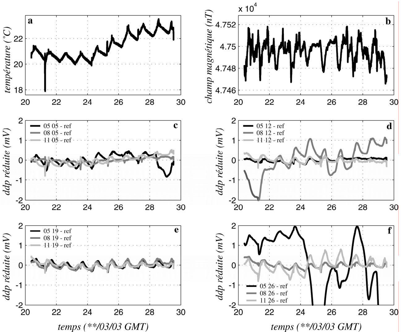
Figure 2.20. Etude des variations journalières. a: température ambiante; b: intensité du champ magnétique à l'observatoire magnétique de Chambon-la-Forêt; c, d, e, f: différences de potentiel (ddp) entre électrodes et référence pour la cuve mise en eau et au repos; le premier chiffre correspond à la coordonnée z, le second à la coordonnée y de l'électrode; les électrodes z = 5 (resp. 8, 11) cm sont à x = -6 (resp. 0, 6) cm (voir figure 2.3), la référence étant placée dans le réservoir amont. Les ddp semblent très fortement corrélées avec la température. Les électrodes à comportement anormal (comme 08 12 ou 05 26) n'ont pas été utilisées par la suite.
