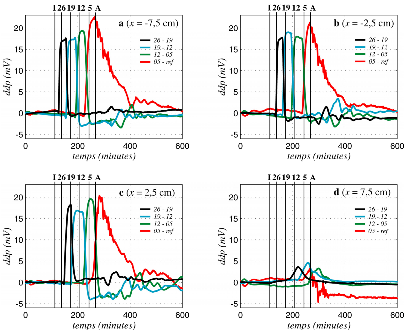
Figure 5.3. Différences de potentiel locales pour l'expérience de contrôle, réduites de leur valeur moyenne sur le temps pré-injection. a et b : séries longitudinales dans la zone liée à l'injection de chlorure de sodium (liée au réservoir B - , x = -7,5 cm et x = -2,5 cm); c et d : séries longitudinales dans la zone liée à la circulation d'eau déionisée pure (liée au réservoir B + , x = 2,5 cm et x = 7,5 cm) (voir figure 5.1). Courbes noires: différences de potentiel entre les électrodes à y = 26 cm et y = 19 cm; bleues: à y = 19 cm et y = 12 cm; vertes: à y = 12 cm et y = 5 cm; rouges: à y = 5 cm et la référence. Barre verticale I: temps d'injection; barres 26, 19, 12, 5: temps de passage théorique du front salin aux électrodes dans l'hypothèse unidimensionnelle à y = 26 , 19, 12 et 5 cm respectivement; barre A: temps d'arrivée théorique dans le réservoir aval. La réponse est de type advectif ( a et b ; voir section 4.2.2). Le sel contamine rapidement la zone située au-delà du plan médian ( c ), mais n'atteint le bord opposé que tardivement ( d ).
