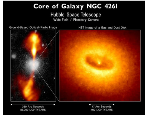
Fig. 1.9: Le noyau de la galaxie NGC 4261. À gauche, la galaxie vue en optique et en radio. Les jets sont bien visibles. À droite, le tore de poussière vu par le télescope spatial Hubble. Image NASA STScI.
