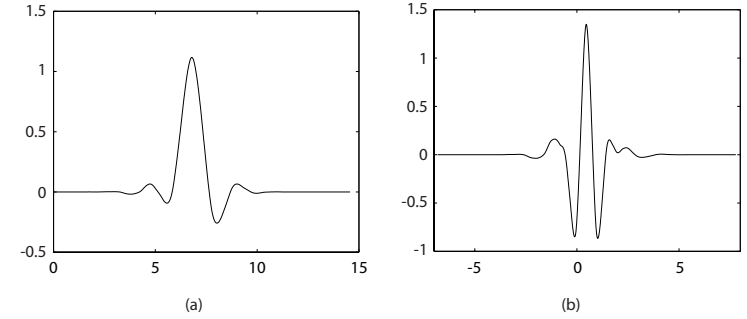
Fig. C.7: (a) La fonction d'échelle \phi et (b) la fonction ondelette \psi symmetre d'ordre 8. D'après [157].
