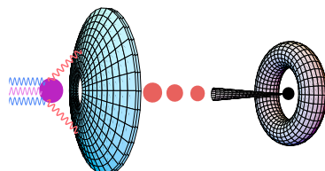
Fig. 2.16: Schéma illustrant le modèle cannonball. D'après [70].
