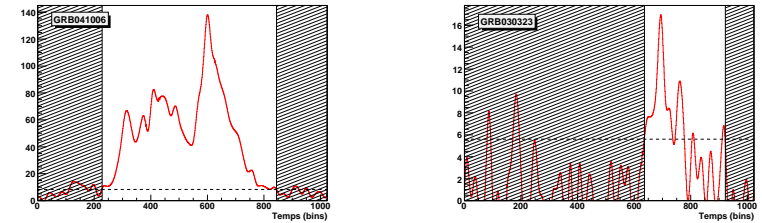
Fig. 9.4: Courbes de lumières débruitées et dont le bruit a été soustrait des sursauts GRB 041006 et GRB 030323. À gauche, pour le GRB 041006, la ligne horizontale correspond à 1\sigma_{\text{bck}} . À droite, pour le GRB 030323, la ligne horizontale correspond à 0.5\sigma_{\text{bck}} . Les zones hachurées montrent les parties des courbes de lumières qui n'ont pas été prises en compte pour la recherche des extrema. L'axe des abscisses est gradué en bins et non pas en secondes.
