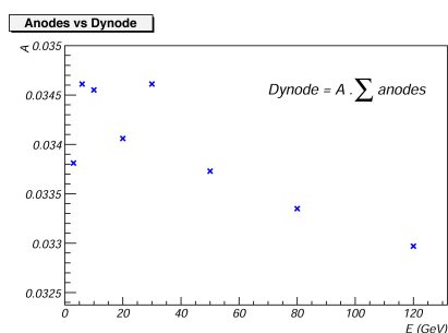
Fig. 6.33: Variations de A en fonction de l'énergie.
