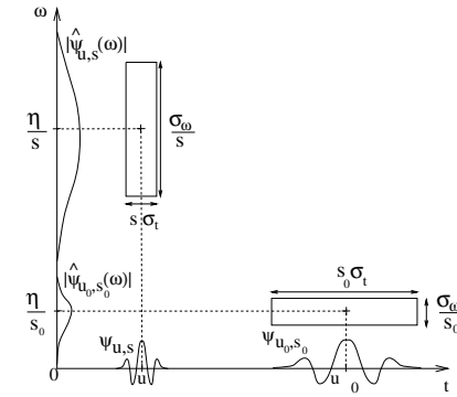
Fig. C.5: Boîtes d'Heisenberg de deux ondelettes \psi_{u_0,s_0} et \psi_{u,s} . L'axe des abscisses représente le temps t et l'axe des ordonnées la fréquence \omega . Dans le domaine fréquentiel, la résolution est donnée en calculant la transformée de Fourier \hat{\psi} de \psi . Lorsque l'échelle augmente, la résolution en fréquence diminue et la résolution en temps augmente. L'aire des boîtes reste constante et égale à \sigma_t\sigma_\omega . D'après [157].
