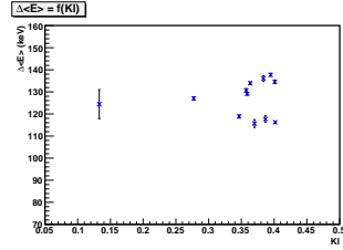
Fig. 10.1: Ecarts moyens en énergie \Delta < E > en fonction du paramètre K_l dans le cas du scénario #2. Deux populations sont visibles pour K_l > 0.3 .
