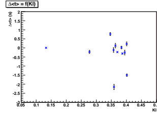
Fig. 10.2: Ecarts moyens en temps \Delta < t > en fonction du paramètre K_l dans le cas du scénario #2. On ne remarque aucune corrélation particulière entre \Delta < t > et la distance des sursauts.
