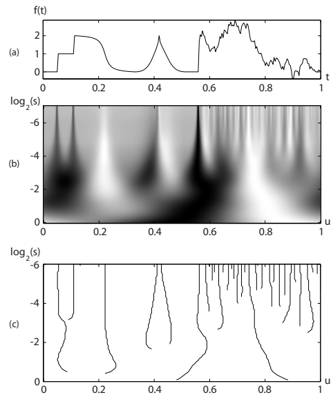
Fig. C.11: CWT et modules maximaux. (a) Le signal de départ. (b) La transformée en ondelette continue. Les valeurs de |Wf(u,s)| sont représentées par une échelle de gris. (c) Les modules maximaux. Chaque courbe correspond à une singularité que l'on suit lorsque l'échelle diminue. D'après [157].
