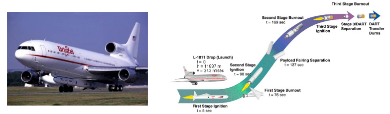
Fig. 4.1: Un lancement de la fusée Pegasus. Le lanceur est initialement accroché à un avion qui l'emporte jusqu'à une altitude d'environ 12000 m, avant de le larguer. Le reste de l'ascension s'effectue avec un moteur fusée. La figure de droite illustre le lancement de DART, un satellite destiné à expérimenter les rendez-vous spatiaux automatiques.
