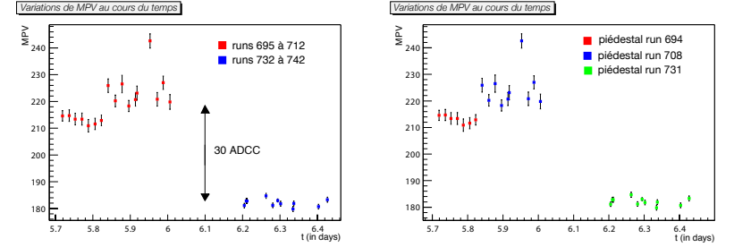
Fig. 6.12: Variation de la MPV au cours du temps. À gauche, les couleurs mettent en évidence les deux populations de MPV. À droite, chaque couleur correspond au run piédestal utilisé.
