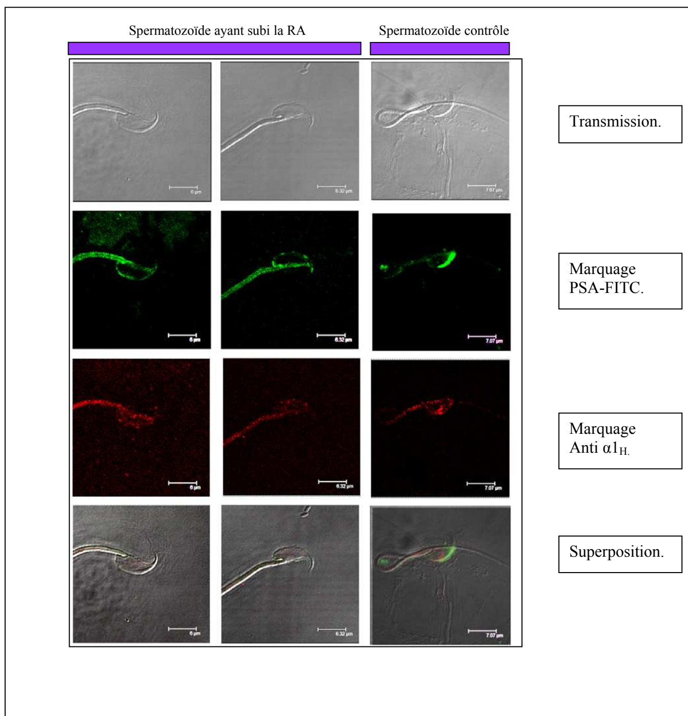
Figure 30 : Immunolocalisation d' \alpha 1_H au niveau de spermatozoïdes contrôle et de spermatozoïdes ayant accompli leur RA.
