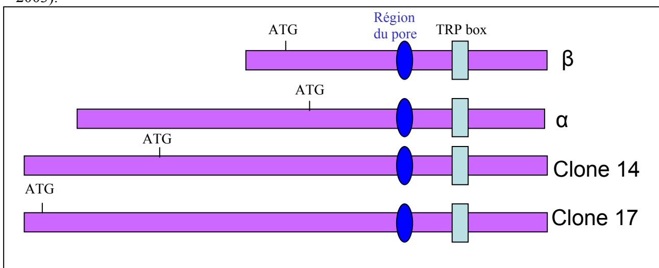
Figure 10: TRPC2 est codé par quatre différents isoformes. Ces isoformes diffèrent par leur séquence Nter et par la position du codon d'initiation (ATG) (d'après Chu et al., 2002).
