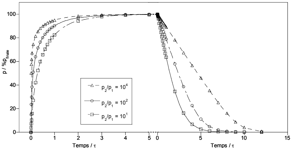
Figure V-20 : Simulation du temps de réponse d'un capteur pour un rapport de pression de (□) 10^1 , (○) 10^2 et (Δ) 10^4
