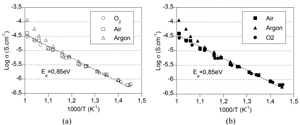
Figure IV-35: conductivité sous oxygène ( \square ), air ( \circ ) et argon ( \Delta ) pour le mélange E (20% \text{Na}_2\text{Ti}_3\text{O}_7 -80% \text{Na}_2\text{Ti}_6\text{O}_{13} ) et (b) un mélange équivalent à E préparé avec les phases pures
