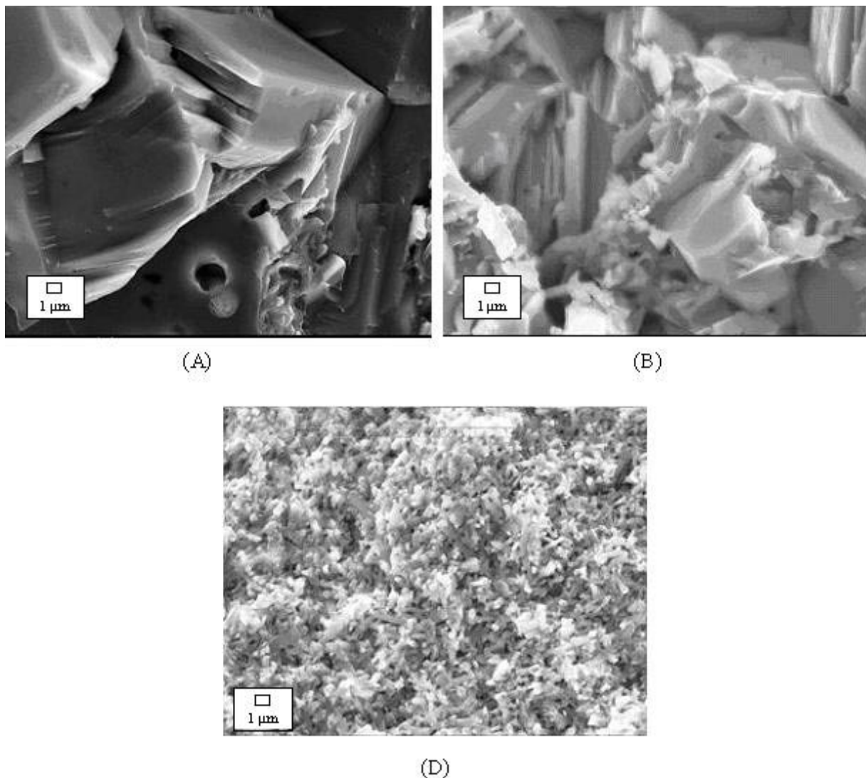
Figure IV-31 : Micrographie de pastilles frittées à 1050^\circ\text{C} pendant 2 heures élaborée à partir des mélanges de composition : (a) 80\%\text{Na}_2\text{Ti}_3\text{O}_7\text{-}20\%\text{Na}_2\text{Ti}_6\text{O}_{13} (A), 55\%\text{Na}_2\text{Ti}_3\text{O}_7\text{-}45\%\text{Na}_2\text{Ti}_6\text{O}_{13} (B) et 35\%\text{Na}_2\text{Ti}_3\text{O}_7\text{-}65\%\text{Na}_2\text{Ti}_6\text{O}_{13} (D)
