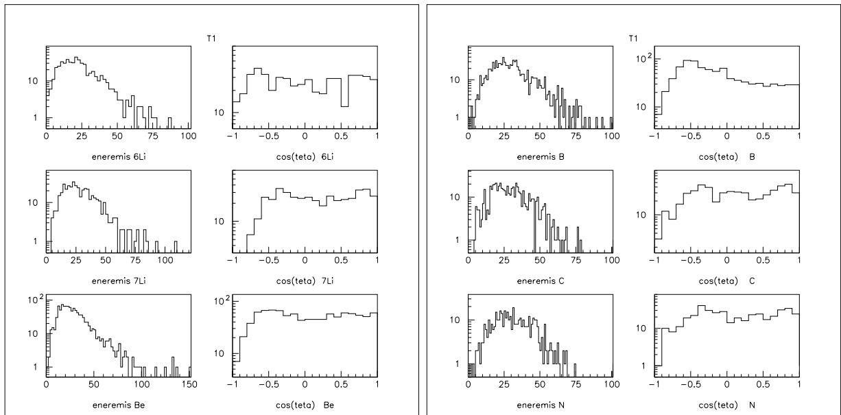
FIG. B.13 – Distributions d'énergie et distributions angulaires dans le repère de la source pour les 6Li , 7Li , Be , B , C et N , pour la tranche T1 .
