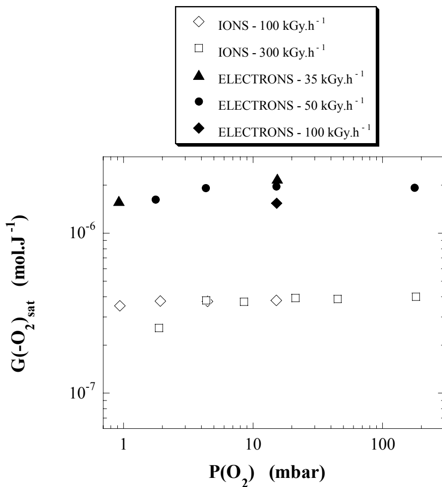
Fig. III-14 : Evolution de G(-O_2)_{\text{sat}} (corrigé de la limitation de l'oxydation par la perméation de l'oxygène dans le matériau) avec la pression moyenne régnant dans la cellule durant l'irradiation pour des irradiations aux ions ^{13}\text{C} ( E=10,75 \text{ MeV.A}^{-1} ) et aux électrons ( E=1 \text{ MeV} ).
