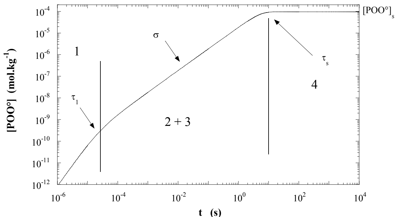
Fig. I-11 : Evolution temporelle de la concentration des radicaux POO^\circ . Le plateau aux temps longs correspond à l'état stationnaire. Les paramètres pris sont les mêmes que ceux de la figure I-10. L'échelle est logarithmique pour les deux axes.
