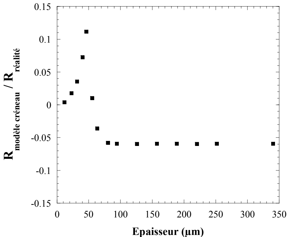
Fig. VII-1 : Comparaison entre le modèle créneau et les valeurs du calcul complet (provenant de la résolution de l'équation de diffusion de Fick) du rapport R = G(-O_2)_{\text{exp}} / G(-O_2)_{\text{surface}} en fonction de l'épaisseur d'échantillon. Pour ce graphique, l'épaisseur critique est égale à 46 µm.
