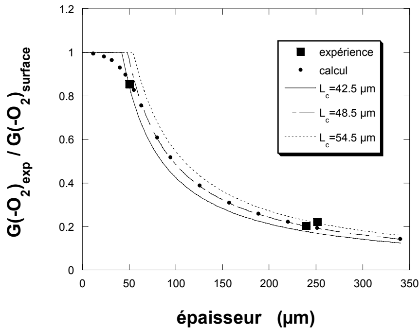
Fig. VII-2 : Evolution de G(-\text{O}_2)_{\text{exp}}/G(-\text{O}_2)_{\text{surface}} avec l'épaisseur d'échantillon. Comparaison entre l'ajustement des trois points expérimentaux par le modèle créneau (défini à la valeur de l'épaisseur critique choisie près) et la courbe obtenue par la résolution de l'équation de Fick avec p=1,23 \cdot 10^{-17} \text{ m}^2 \cdot \text{mol} \cdot \text{s}^{-1} \cdot \text{kg}^{-1} \cdot \text{Pa}^{-1} , P(\text{O}_2)=8,7 \text{ mbar} et I=280 \text{ kGy} \cdot \text{h}^{-1} . Le profil v(u) utilisés est celui de la figure I-16 (page 73).
