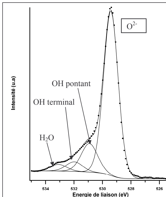
Figure 18 : Spectre XPS du pic O_{1s} de la poudre de rutile non sorbée.
