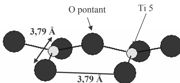
Figure 4 : Unité de surface de la face (001) de la phase anatase.
