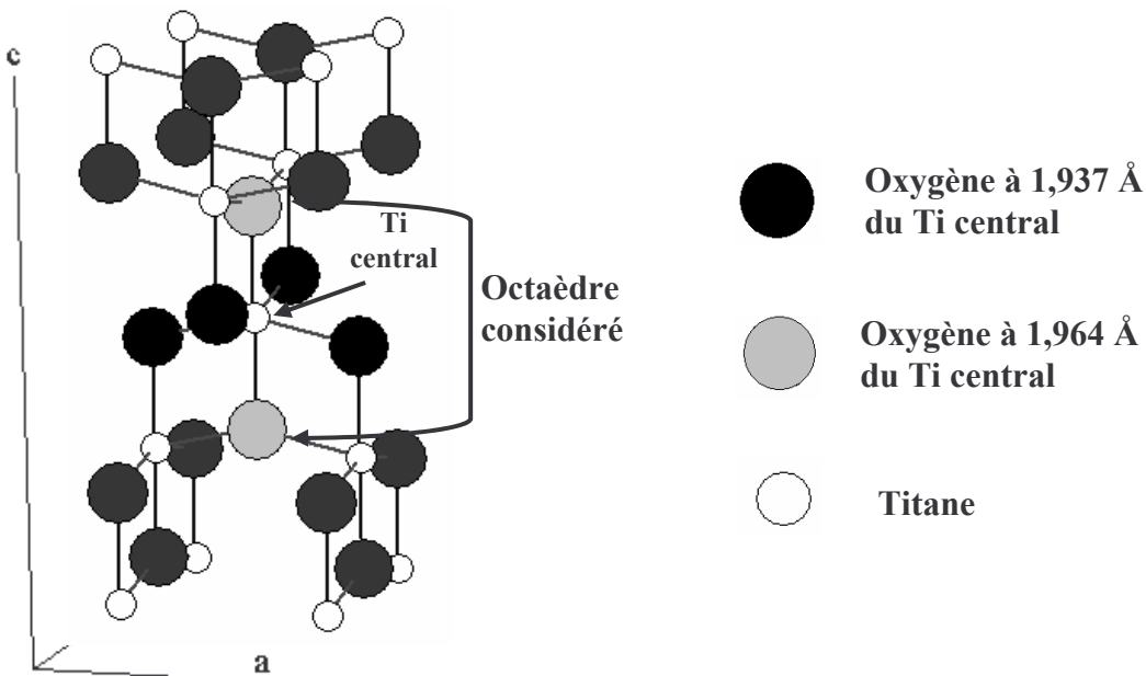
Figure 2 : Représentation de la maille de la phase anatase.
