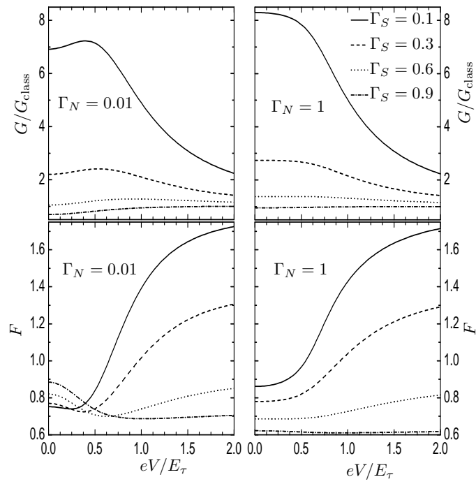
Fig. 5.7: Conductance différentielle et facteur de Fano en fonction de eV/E_\tau à température nulle. Les deux barrières ont une distribution de transparence monomodale. Dans l'encart gauche, la jonction N-N' est tunnel ( \Gamma_N = 0.01 ) et dans l'encart droit la jonction N-N' est transparente ( \Gamma_N = 1 ).
