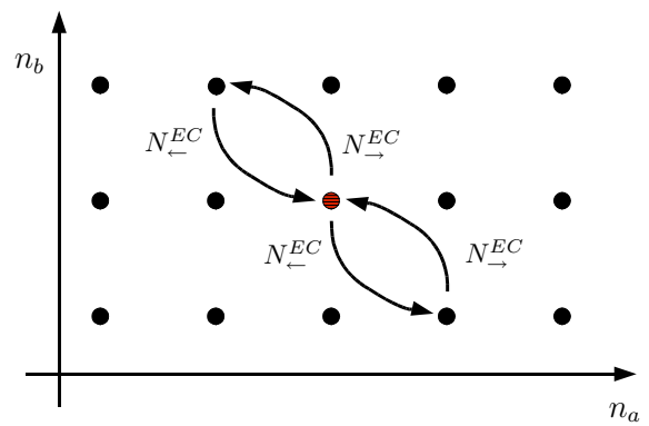
(c) Cotunneling élastique
