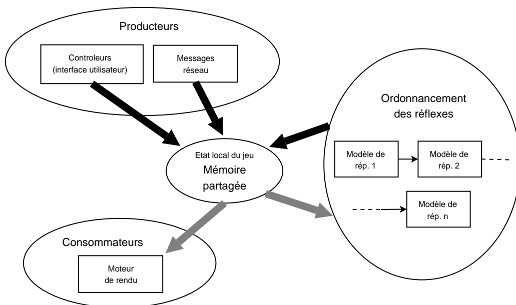
FIG. 4.2 – Architecture des processus de l'application sur un hôte
