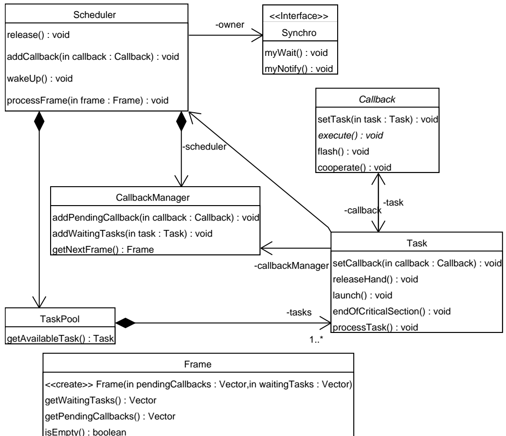
FIG. 6.1 – Ordonnement des réflexes, diagramme de classes
