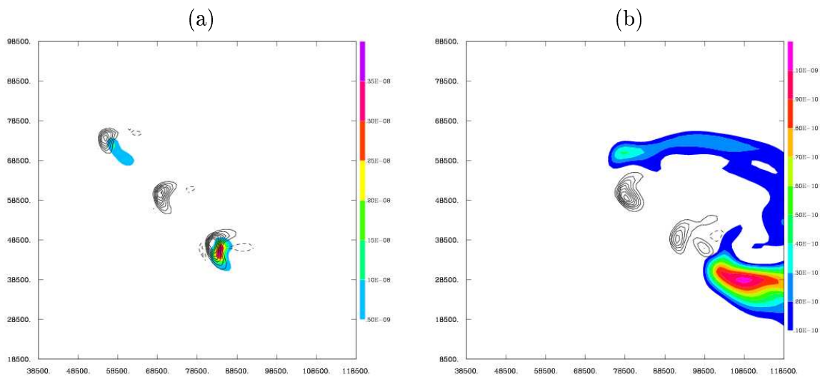
FIG. 5.16 – Coupes horizontales des rapports de mélange des LiNO x (surfaces colorées) et de la vitesse verticale (isocontours noirs) à (a) 3600 s et (b) 9000 s.
