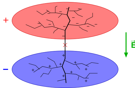
FIG. 2.7 – La région rouge représente une zone chargée positivement, et la région bleue située au dessous, une zone chargée négativement. Le vecteur champ électrique est donc dirigé vers le bas. La croix rouge représente le point de déclenchement de l'éclair, et la trajectoire de l'éclair est matérialisée par les lignes noires. Les branches positives se propagent donc dans la zone de charge négative, et c'est l'inverse pour les branches négatives.
