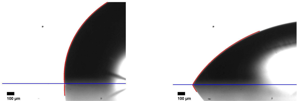
FIG. 4.9: Profils de gouttes typiques extraits numériquement, pour 0 et 1100 V. Sur les photos de la figure 4.8, en rouge les profils extraits. Le trait horizontal bleu désigne la position de la ligne triple. Échelle 100 \mu\text{m} .
