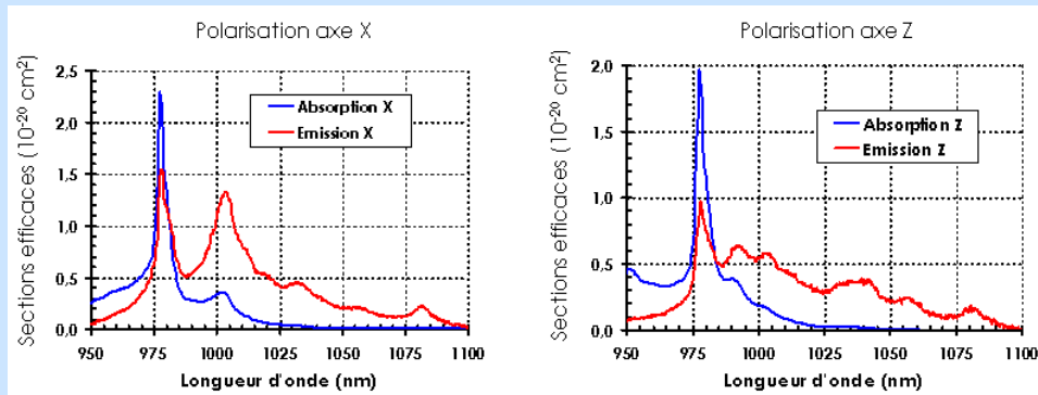
Spectres d'absorption (en bleu) et d'émission (en rouge) selon les deux polarisations accessibles (X et Z) de nos échantillons d'Yb:YSO.
