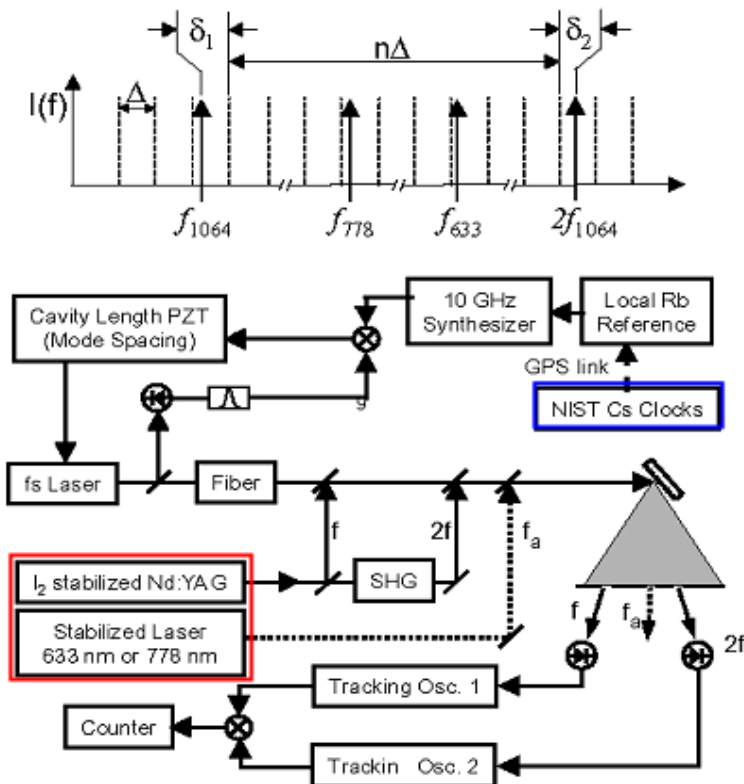
Figure A-5b : Chaînes de mesures de fréquences de lasers stabilisés à 532, et 633 ou 778 nm par peigne de fréquences d'un oscillateur femtoseconde [Diddams, 00] - A gauche (encadré gras) les lasers dont les fréquences sont à mesurer, à droite (encadré gras) l'horloge atomique à Cs de référence.
