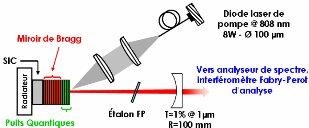
Figure C-16 : Schéma expérimental de la cavité pour une émission monomode longitudinale autour de 1003,4 nm. L'angle de pompage est d'environ 20° et la longueur de la cavité de 95 mm.
