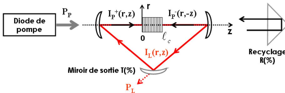
Figure B-35 : Cavité et notations utilisées pour les simulations.
