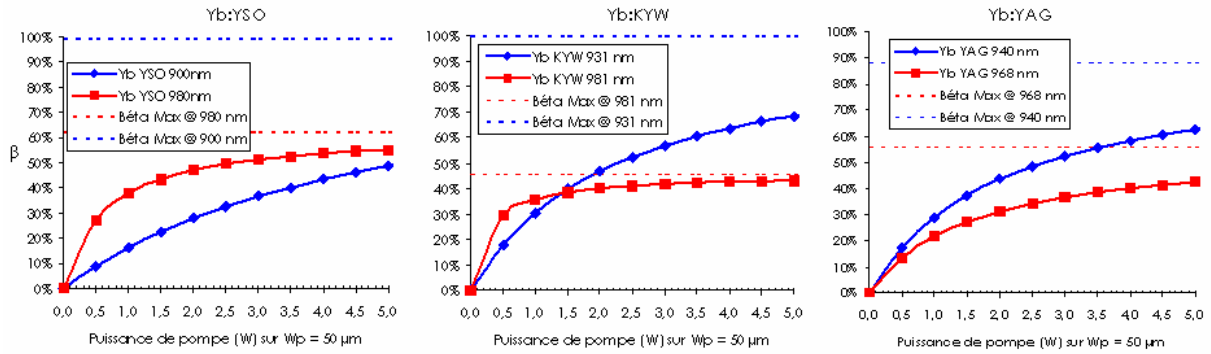
Figure B-7 : Comparaison de l'évolution du taux d'inversion de population \beta à deux longueurs d'onde de pompe pour les cristaux de Yb:YSO, Yb:KYW et Yb:YAG. Les limites en pointillés correspondent aux valeurs maximales de \beta pour les différentes longueurs d'onde de pompe, lorsque la puissance de pompe tend vers l'infini.
