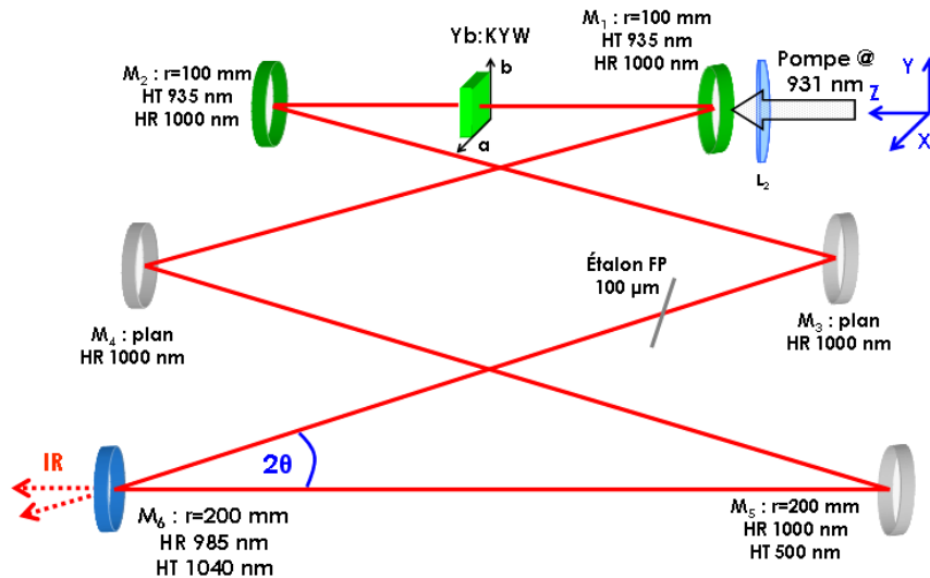
Figure B-33 : Cavité en anneau utilisée avec le cristal de Yb:KYW pompé à 931 nm pour l'oscillation laser à 1020 nm.
