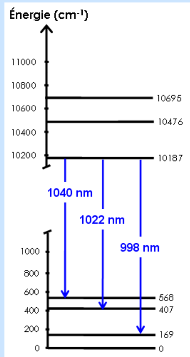
Niveaux énergétiques et transitions possibles pour \text{Yb}:\text{KYW} .
