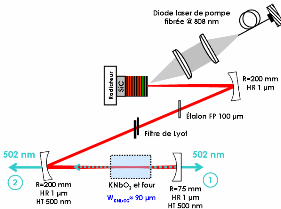
Figure C-19 : Cavité à 4 miroirs utilisée pour le doublement de fréquence de l'infrarouge vers le visible. Le mode de cavité au niveau de la \frac{1}{2} structure VCSEL est d'environ 100 µm et d'environ 90 µm au niveau du cristal non linéaire.
