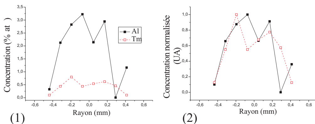
FIG. 2.25 – Mesure de la composition du cœur de A11 par EPMA sur une coupe transverse (1) en % mol et (2) normalisé
