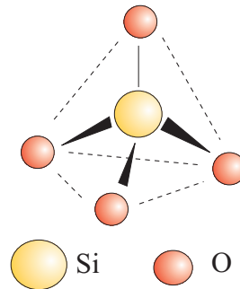
FIG. 1.20 – Tétraèdre SiO_4
