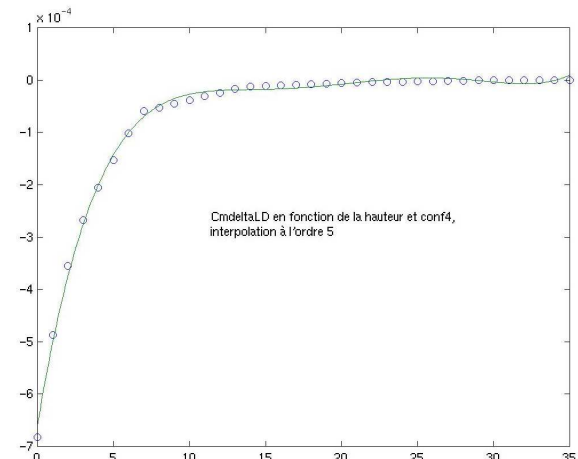
2.3.2.1.1.d : CmLD en fonction de la hauteur pour l'A321 en conf. 4 – Polynôme d'ordre 5
