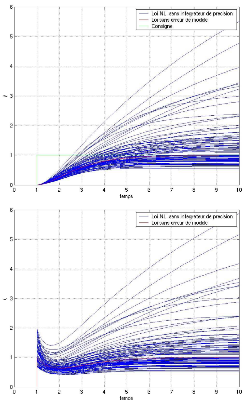
2.2.7.1.a : Tracés des résultats d'une loi de commande de type non-linéaire inverse (sans intégrateur de précision) synthétisée à partir d'un modèle incertain à +50%
