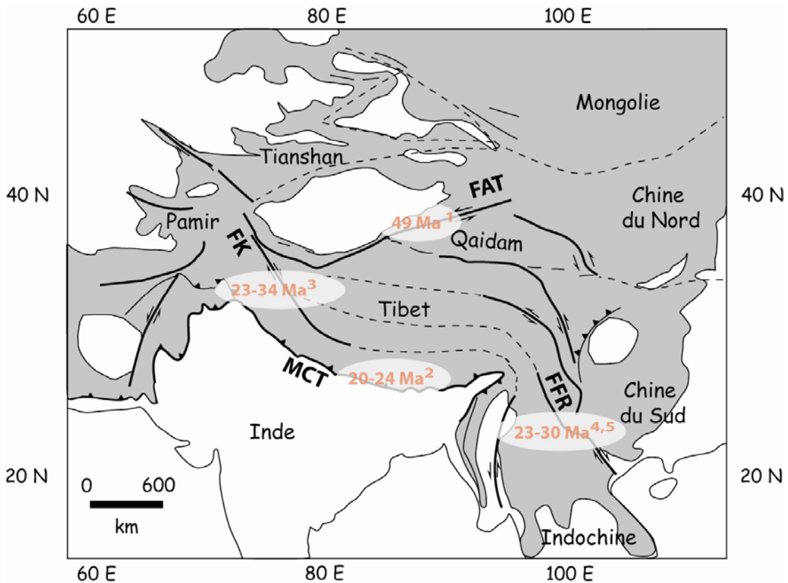
Fig. 1.7 : carte structurale des grands décrochements d'Asie du sud et centrale, et âges supposés des premiers mouvements décrochants dus à la collision Inde-Asie, FAT : faille de l'Altyntagh ; FK, faille de Karakorum ; FFR : faille du Fleuve Rouge ; MCT : Main Central Thrust ; 1 Yin et al. (1998) ; 2 Caltos et al. (2002) ; 3 Lacassin et al., (2001) ; 4 Tapponnier et al. (1990) ; 5 Sharer et al. (1994)
