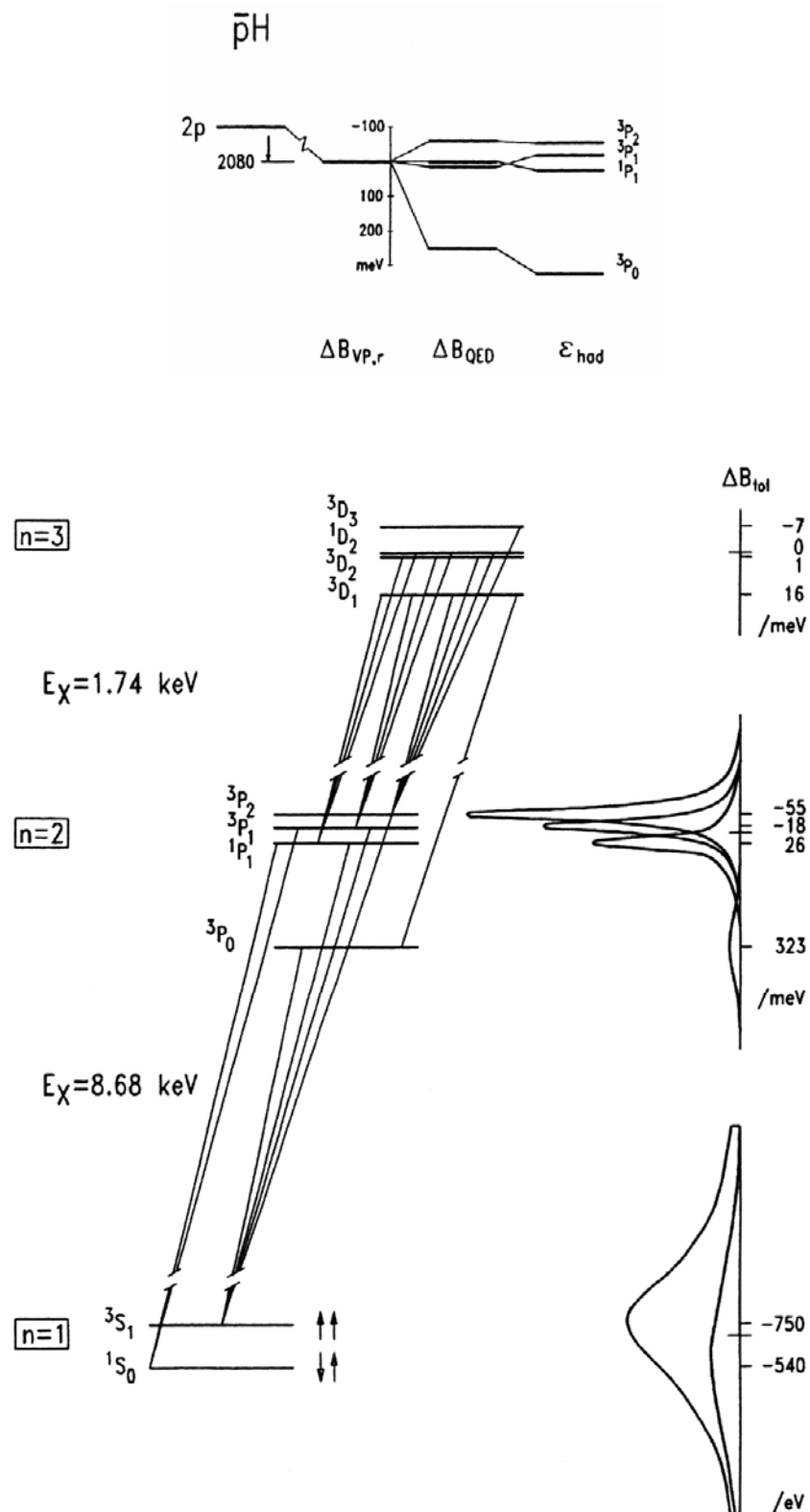
Figure 1-2: Séparation des niveaux 2p hyperfins (en haut) et cascade atomique 3d → 2p → 1s (en bas) dans le protonium. Les calculs électromagnétiques \Delta B_{QED} sont pris de [28], le décalage hadronique \mathcal{E}_{had} de [27].
