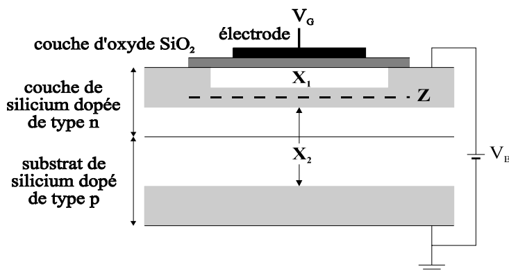
Figure 2-17: Création de zones de déplétion X_1 et X_2 près d'une électrode grâce aux tensions V_G et V_B . Pour une certaine tension V_B , les deux zones se rejoignent en Z et forment un puits de potentiel.
