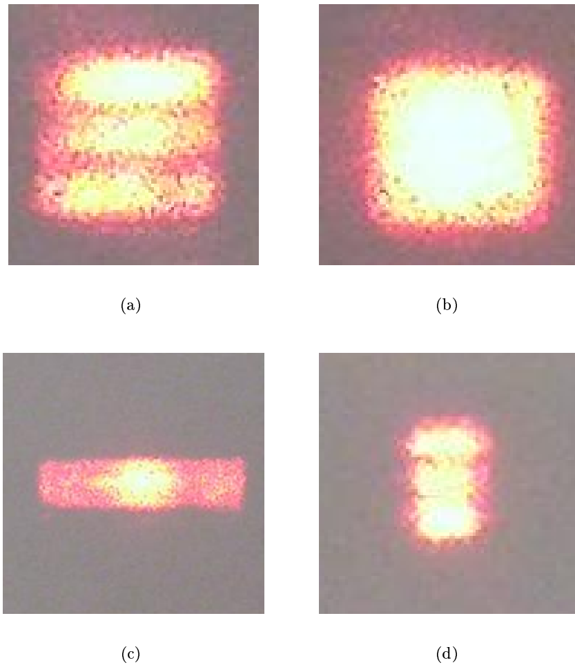
FIG. 5.8: Observations des sorties de différents guides creux métalliques dans le visible ( \lambda = 0,6\mu\text{m} ). Les figures a. et b. concernent un guide de dimensions 10\mu\text{m} \times 10\mu\text{m} , tandis que c. et d. concernent un guide de largeur 5\mu\text{m} comportant ou non un cornet en entrée.
