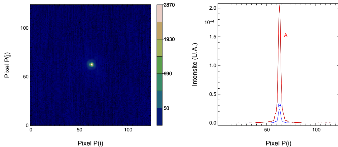
FIG. 4.25: Gauche : image de la tache d'entrée après injection dans un trou filtrant de diamètre 10\ \mu\text{m} dans un champ de 124 \times 124 pixels. Le niveau moyen du fond thermique a été soustrait à l'image brute. Droite : comparaison entre les taches de sortie dans le cas de la propagation libre du faisceau (courbe notée "A") et dans le cas d'un faisceau injecté (courbe notée "B"). L'intensité est donnée en unités arbitraires et est directement proportionnelle aux données de la caméra infrarouge.
