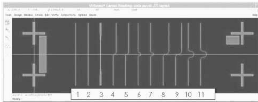
FIG. 5.2: Exemple de masque lors de la réalisation de guides creux. Le guide numéro 3 possède un cornet en entrée et en sortie.
