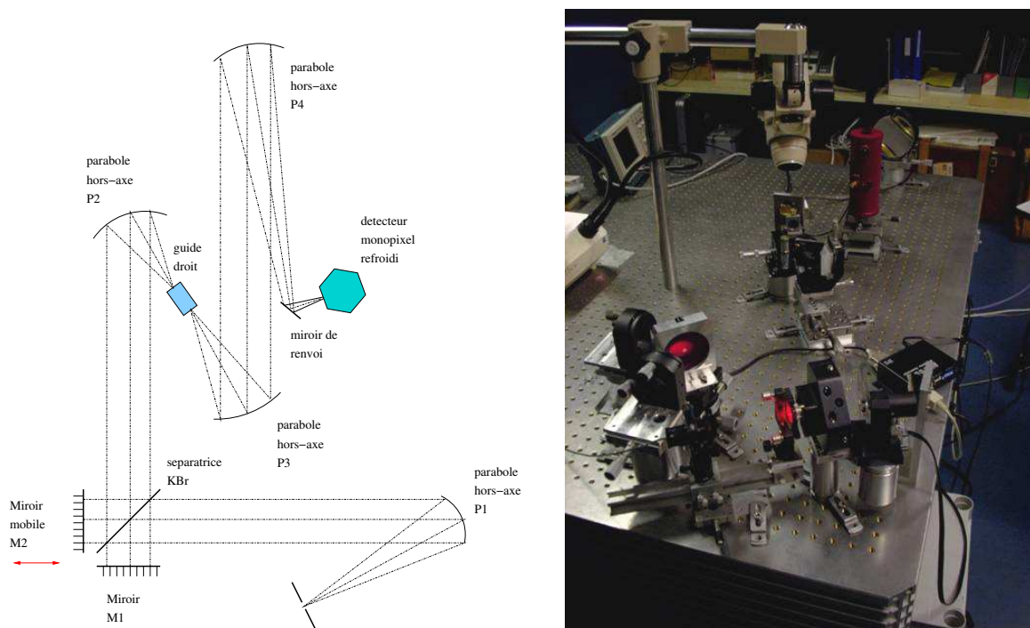
FIG. 4.33: Banc de spectrométrie par transformée de Fourier pour la mesure des coupures de modes sur différents types de guides d'onde. Le miroir mobile M_2 permet une course maximum de 2 cm au total.
