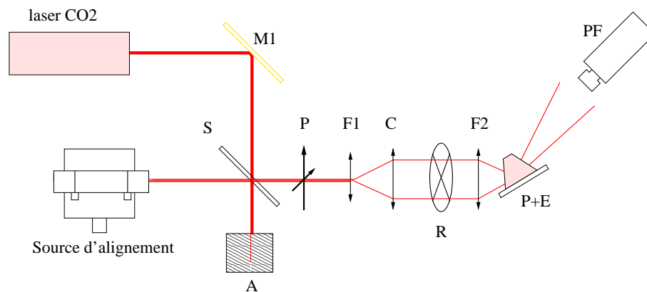
FIG. 4.8: Schéma optique du banc de m -lines développé à 10\mu\text{m} . M_1 : miroir de renvoi ; S : séparatrice en \text{ZnSe} , \varnothing 50\text{ mm} ; A : matériau absorbant ; P : polariseur à grille ; F_1 : première lentille de focalisation, f=25,4\text{ mm} ; C : collimateur, f=254\text{ mm} ; R : réticule ; F_2 : seconde lentille de focalisation, f=76,2\text{ mm} ; P+E : ensemble prisme-échantillon ; PF : plan focal de la caméra infrarouge.
