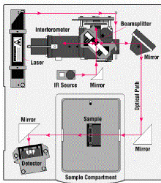
FIG. 4.1: Schéma descriptif d'un Spectromètre à transformée de Fourier
