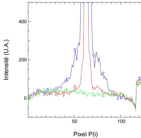
FIG. 4.27: Coupe des images enregistrées par la caméra pour le signal direct (bleu+carrés), pour le signal transmis à travers le trou de 10 \mu\text{m} (rouge+cercles) et pour le signal de "dark" (vert+croix). Le niveau de signal est en "unités arbitraires" (U.A.). La soustraction du niveau de fond thermique permet de supprimer les défauts du détecteur tels que l'artefact visible sur la droite de la courbe.
