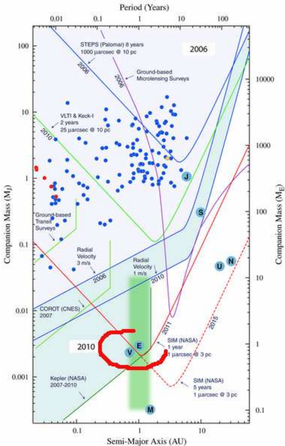
FIG. 2.1: Vue d'ensemble des méthodes de recherche de planètes extra-solaires en fonction de la masse et de la distance à l'étoile. Les différentes planètes de notre Système Solaire sont placés dans ce schéma. Le cercle rouge correspond à la zone des planètes telluriques habitables. Les différentes planètes de notre système solaire sont placés dans ce schéma. Image tirée de Lawson (2004)
