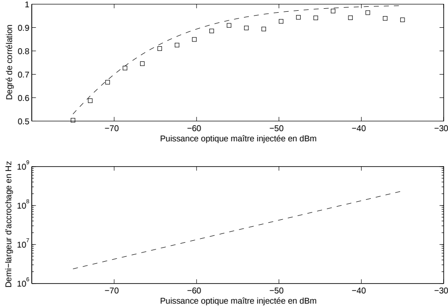
FIG. 6.2 – Mesure du degré de corrélation entre le laser maître et le laser esclave en fonction de la puissance injectée
