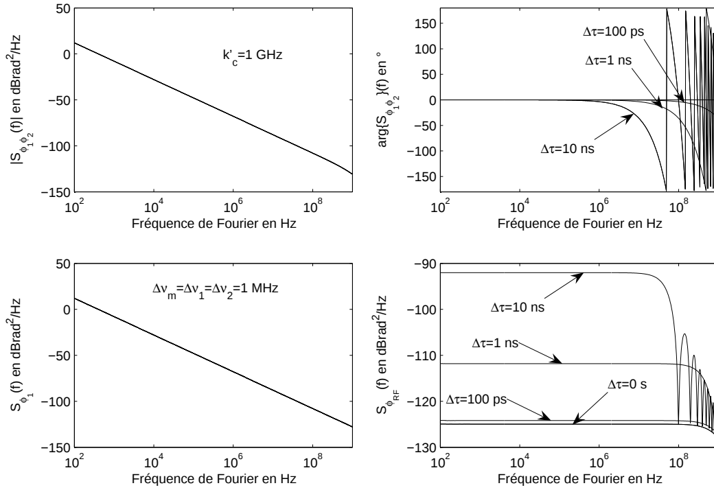
FIG. 7.6 – Influence d'un délai entre les deux ondes optiques sur le bruit de phase micro-onde
