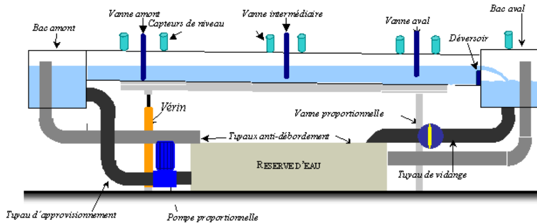
Figure 5.10 : Schéma de la maquette de micro-canal de Valence
