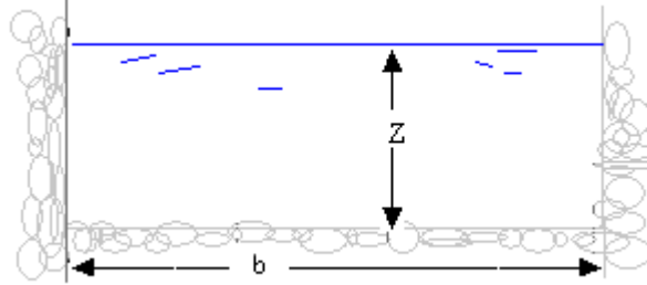
Figure 1.4 : Coupe transversale d'un canal rectangulaire
