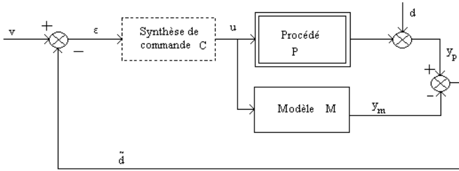
a. Structure de commande en boucle fermée
