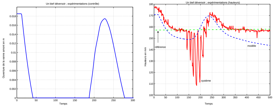
Figure 5.16 : Un bief déversoir ; perturbations
