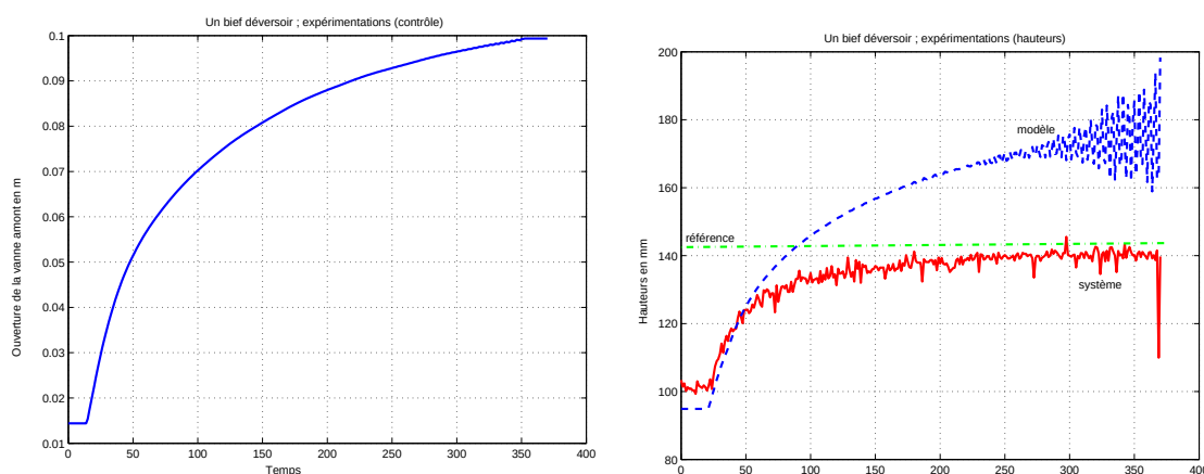
Figure 5.15 : Un bief déversoir ; variation de 50%
