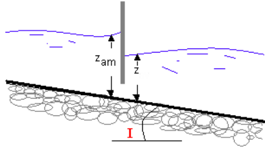
Figure 1.6 : Coupe d'une vanne noyée
