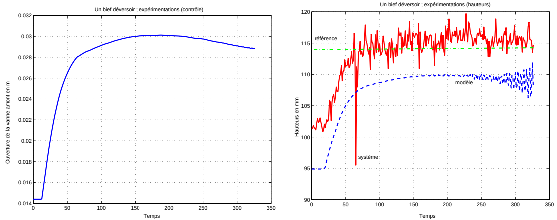
Figure 5.14 : Un bief déversoir ; \alpha_i = 2
