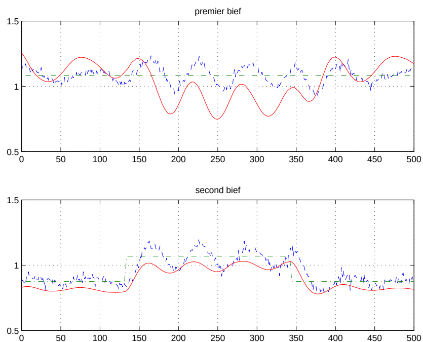
Figure 5.25 : Deux biefs, trois vannes
