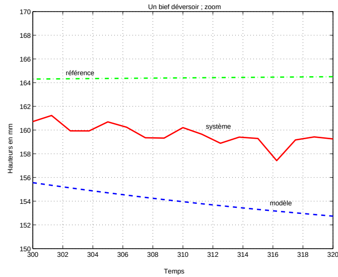
Figure 5.17 : Un bief déversoir ; zoom
