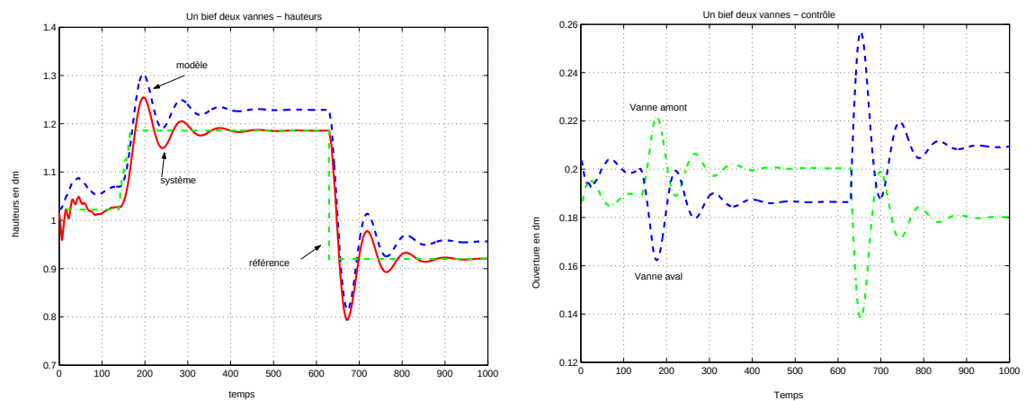
Figure 5.2 : Bief avec deux vannes ; Hauteurs et ouverture des vannes
