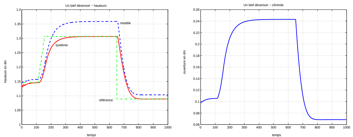
Figure 5.1 : Déversoir : hauteurs et ouverture de la vanne amont
