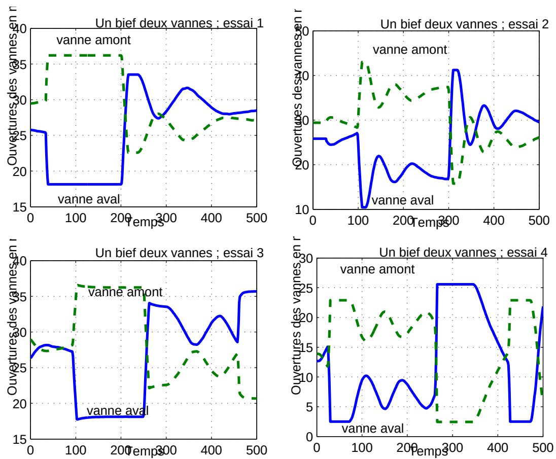
Figure 5.20 : Un bief deux vannes ; Ouverture des vannes
