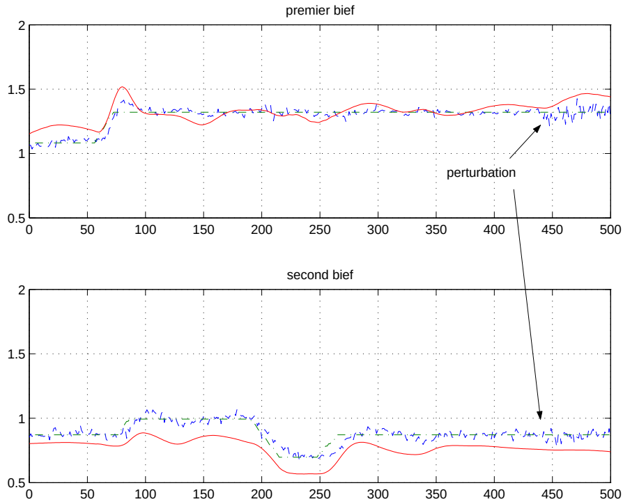
Figure 5.26 : Deux biefs, trois vannes ; perturbations (manuelles)
