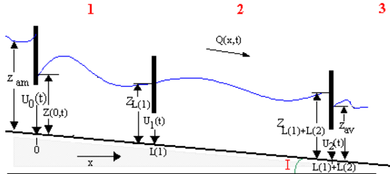
Figure 1.3 : Schéma d'un Canal : deux biefs en cascade
