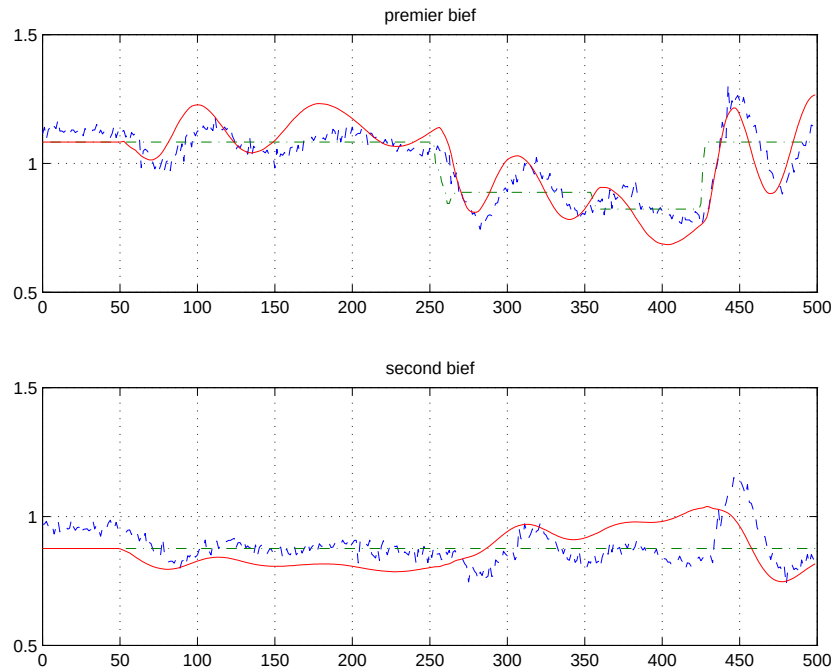
Figure 5.24 : Deux biefs, trois vannes
