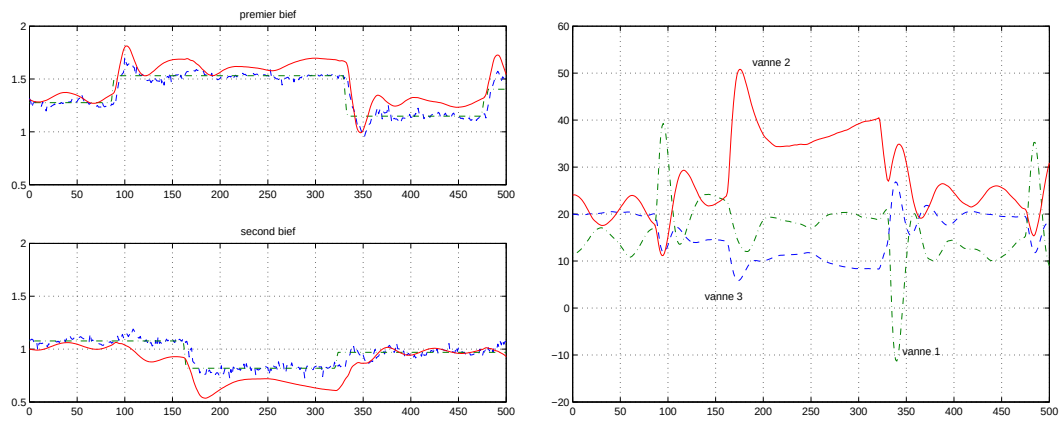
Figure 5.22 : Hauteur aval dans les 2 biefs (dm) et ouvertures des 3 vannes (mm)
