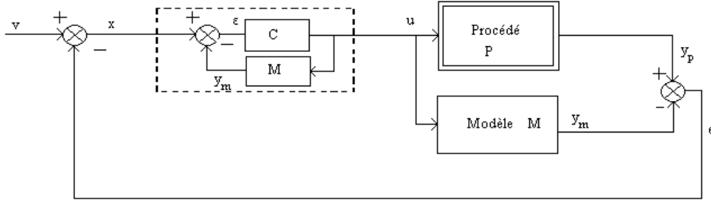
Figure 2.2 : Structure MCI modifiée
