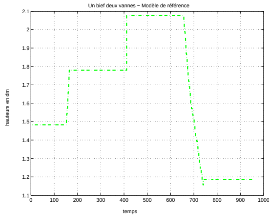
Figure 5.4 : Le modèle de référence
