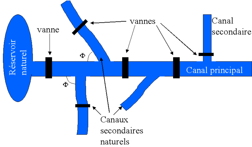
Figure 1.1 : Réseau de canaux d'irrigation
