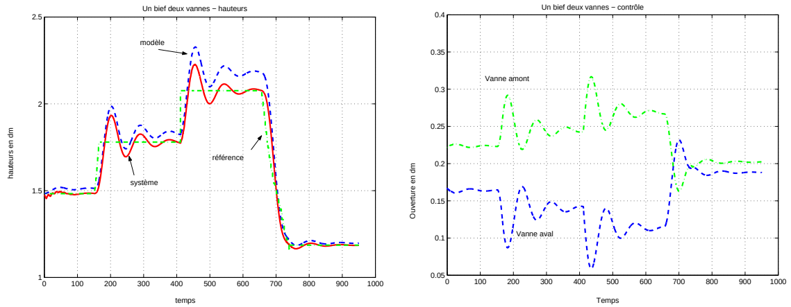
Figure 5.3 : Un bief deux vannes ; variation des pentes de la consigne
