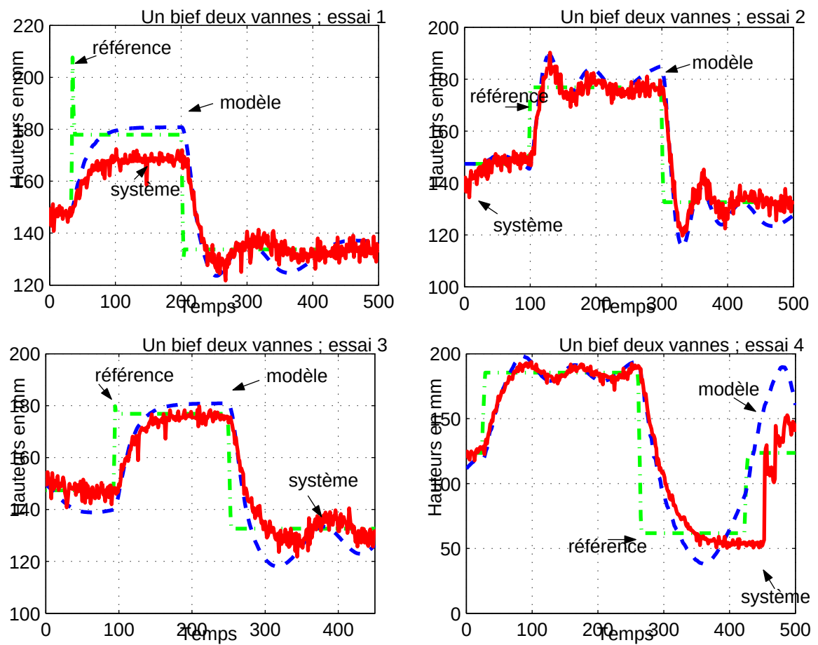
Figure 5.19 : Un bief deux vannes ; Hauteurs
