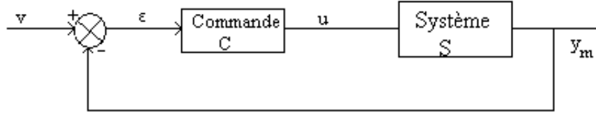
a. Structure de commande en boucle fermée
