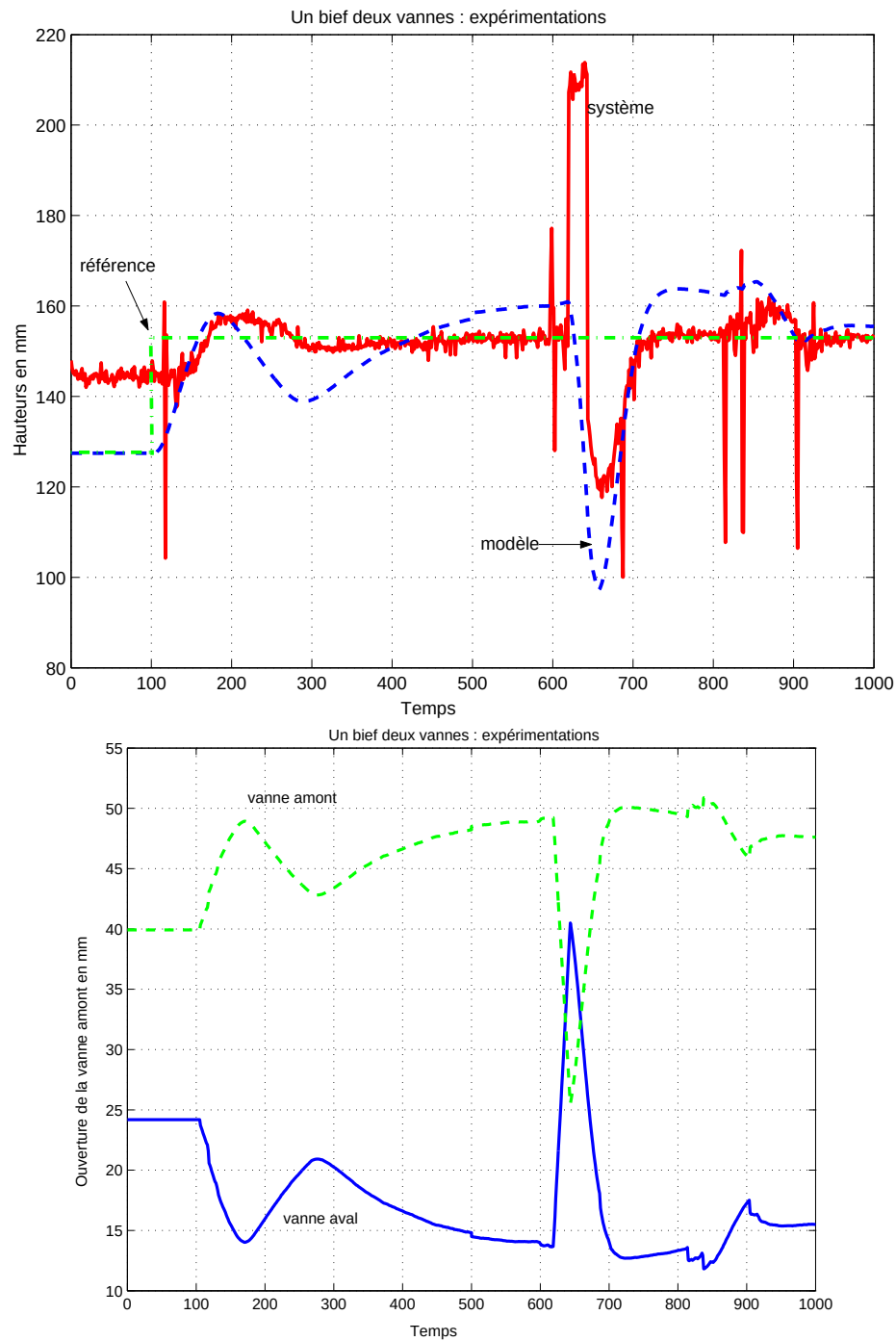
Figure 5.18 : Un bief deux vannes ; ouverture des vannes et hauteurs d'eau
