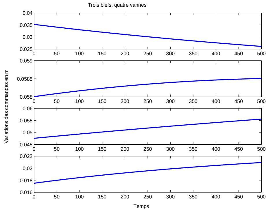
Figure 5.6 : Trois biefs avec quatre vannes : ouverture des vannes
