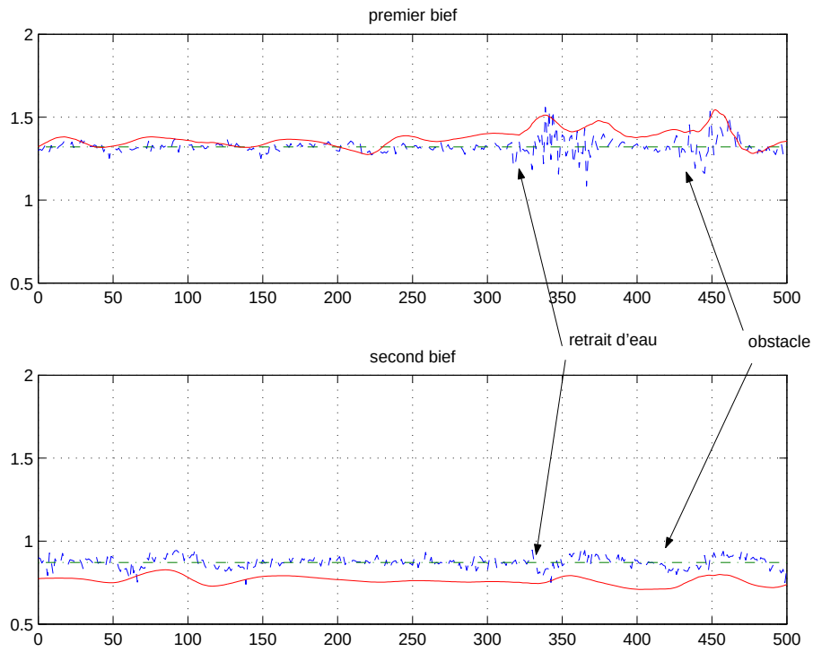
Figure 5.27 : Deux biefs, trois vannes ; perturbations (retraits d'eau et obstacles)
