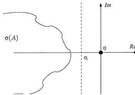
Figure 4.2 : Spectre de l'opérateur A_e
