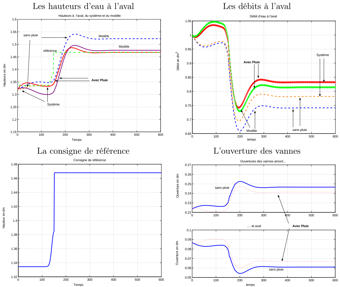
Figure 5.7 : Perturbation : phénomène de pluie
