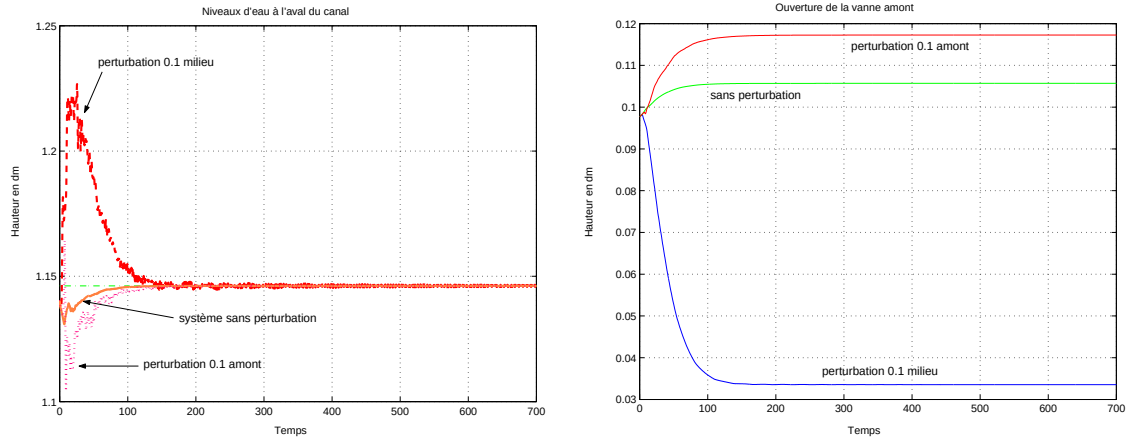
Figure 5.8 : Perturbation : jonction d'un canal secondaire
