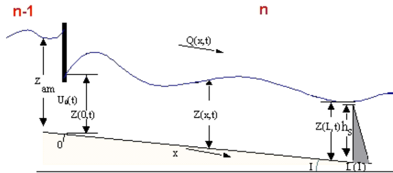
Figure 1.2 : Schéma d'un Canal : un bief déversoir
