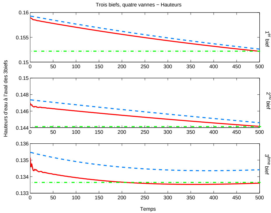
Figure 5.5 : Trois biefs avec quatre vannes : hauteurs
