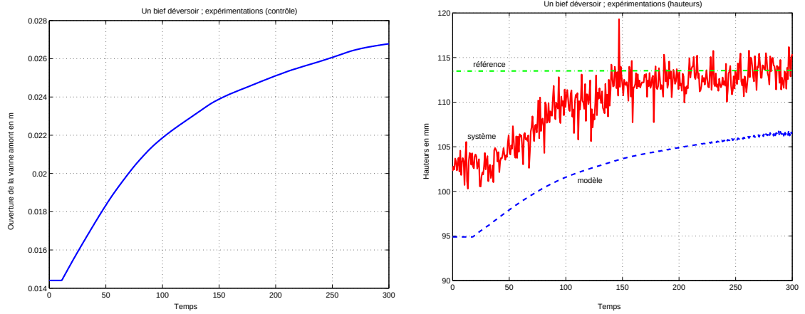
Figure 5.13 : Un bief déversoir ; ouverture de la vanne et hauteurs d'eau
