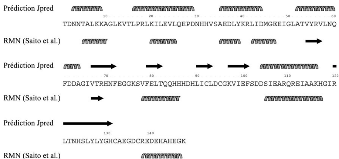
Figure I.20 : Comparaison de la prédiction de structure secondaire obtenue avec Jpred (34, 56) avec les données RMN obtenue par Saito et al. (95). La prédiction de structure avec le serveur JPred suggère la présence d'un motif de liaison à l'ADN de type hélice-coude-hélice ailé. Les données RMN et la prédiction de structure ne sont pas en accord.
