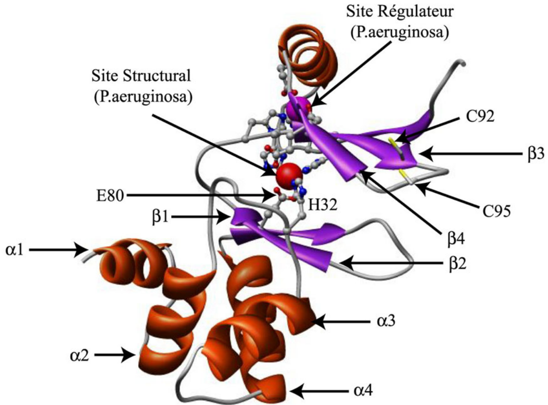
Figure VII.2 : Modèle de Zn R Zn S FUR D de FUR d' E.coli réalisé avec Swiss-model à partir de la structure cristallographique de Zn R Zn S FUR D de P.aeruginosa . Les Zn(II) (sphères rouge et violette) correspondent aux Zn(II) observés dans la structure cristallographique de FUR de P.aeruginosa .
