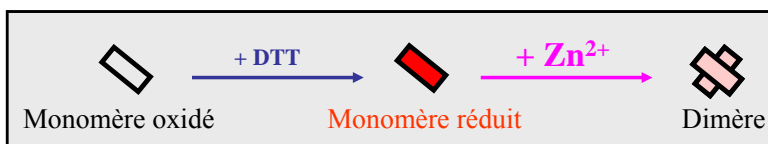
Figure IV.4 : Le passage du monomère au dimère nécessite d'abord la réduction des cystéines puis l'incorporation de zinc.
