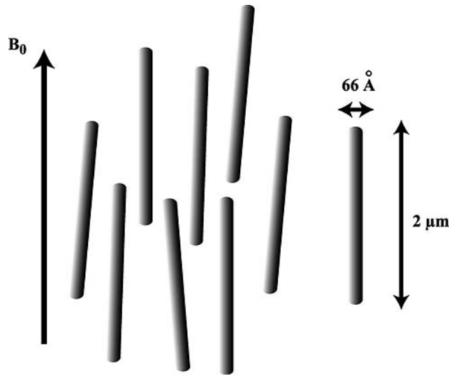
Figure II.16 : Schéma représentant l'alignement des phages dans un champ magnétique B_0 .
