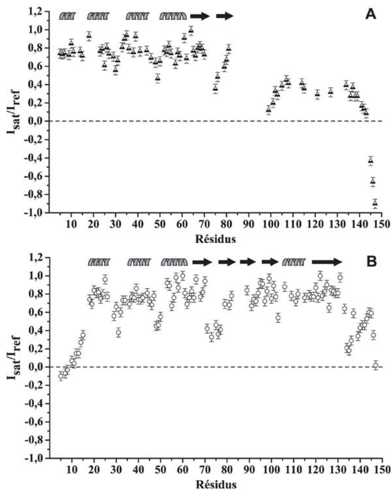
Figure IV.14 : NOE ^1\text{H} - ^{15}\text{N} enregisté à 600 MHz à l'équilibre du monomère (A) et du dimère (B).
