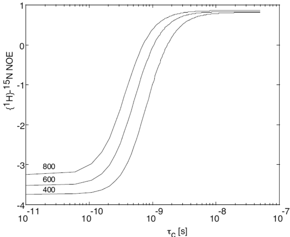
Figure II.25 : Variation du paramètre NOE ^1\text{H}-^{15}\text{N} en fonction du \tau_c du vecteur N-H. le NOE hétéronucléaire ^1\text{H}-^{15}\text{N} permet d'identifier des mouvement dans la gamme [10^{-10} : 10^{-8}] s.
