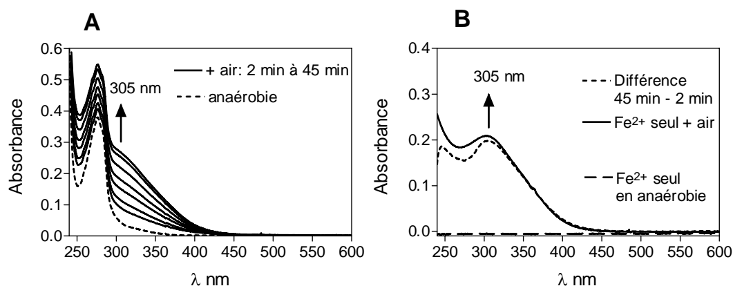
Figure V.4 : Spectre d'absorption électronique. (A) Monomère à une concentration de 56 \mu\text{M} dans un tampon BTP 0,1M, KCl 0,1M, pH = 7,5 + 1 éq de \text{Fe}^{2+} préparé en anaérobie. Spectre enregistré en anaérobie (trait pointillé), spectres enregistrés 2, 5, 10, 15, 22, 35 et 45 minutes après ouverture à l'air (traits pleins). (B) Comparaison des spectres de différence du monomère + \text{Fe}^{2+} entre 45 minutes et 2 minutes après ouverture à l'air et d'une solution de sel de Mohr ( \text{Fe}(\text{SO}_4)_2(\text{NH}_4)_2 \cdot 6\text{H}_2\text{O} ) à 55 \mu\text{M} dans le tampon BTP 0,1M, KCl 0,1M à pH = 7,5 avant et après ouverture à l'air. (Repris de la thèse de B.D'Auréaux (4))
