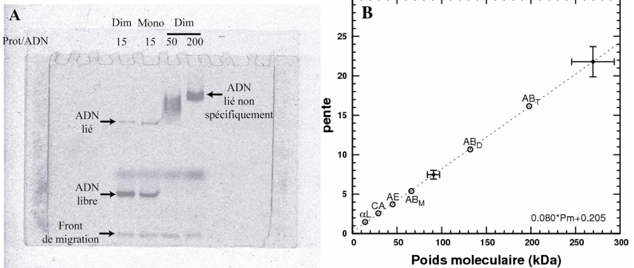
Figure VI.11 : Détermination du poids moléculaire du complexe FUR D /ADN. A) exemple de gel visualisé par fluorescence montrant la migration de l'ADN. B) Graphique représentant la variation de migration des espèces suivant le % d'acrylamide (pente) en fonction du poids moléculaire des espèces. Les marqueurs utilisés sont l' \alpha -lactalbumine ( \alpha L), l'anhydrase carbonique (CA), l'albumine d'œuf (AE) et l'albumine bovine que l'on trouve sous forme monomère (AB M ) dimère (AB D ) et tétramère (AB T ). Les points \blacklozenge avec les barres d'erreurs correspondent aux valeurs de pentes obtenues pour les complexes FUR D /ADN.
