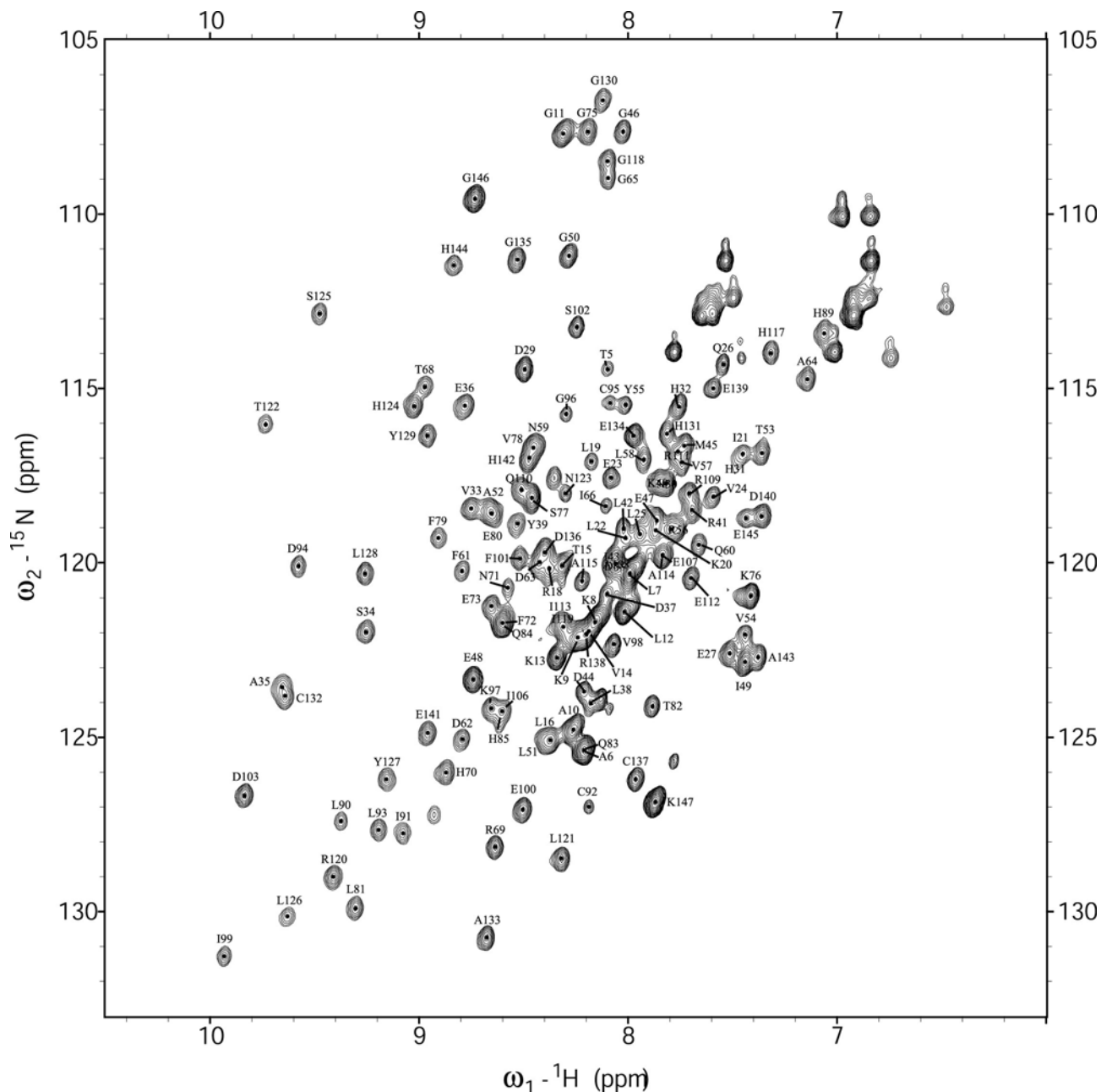
Figure III.4 : Spectre HSQC ^1\text{H} - ^{15}\text{N} du dimère \text{Zn}_5\text{FUR}_D avec l'attribution
