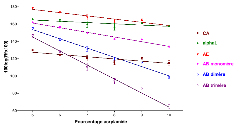
Figure VI.10 : Migration des différents marqueurs en fonction du pourcentage d'acrylamide.
