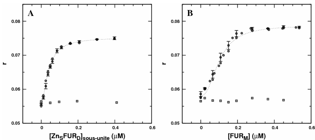
Figure VI.8 : Titration par anisotropie de fluorescence de 10 nM d'ADN consensus dans MOPS 20 mM KCl 125 mM poly-dIdC 10\ \mu\text{g.mL}^{-1} \text{MgSO}_4 12 mM pH 7 par une concentration croissante de FUR dimère (A) ou monomère (B). Les cercles correspondent aux expériences réalisées en présence de 1 mM de \text{MnSO}_4 et les carrés correspondent aux expériences réalisées en absence de \text{MnSO}_4 . Les données sont ajustées avec l'équation de Hill (courbe pointillées) afin d'obtenir un K_d apparent. A) K_d apparent de 40 \pm 1\ \text{nM} B) K_d apparent de 102 \pm 2\ \text{nM} .
