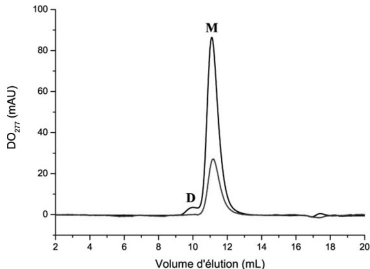
Figure VI.3 : Profil d'élué par chromatographie d'exclusion sur gel (Superdex 75 HR 10/30) d'une solution de 80 \mu M de monomère issu de la dernière étape de purification puis incubé 15 minutes en présence de 10 équivalents de Mn^{2+} (en noir). Profil d'élué d'une solution à 25 \mu M de monomère sélectionné après incubation avec 10 équivalents de Mn^{2+} (normalement incapable de dimériser) et réincubé avec 10 équivalents de Mn^{2+} (en gris). Le monomère obtenu de cette façon est incapable de dimériser. L'absence d'un pic correspondant au volume d'élué du dimère montre que le monomère oxydé reste monomère en présence d'un excès de Mn^{2+} .
