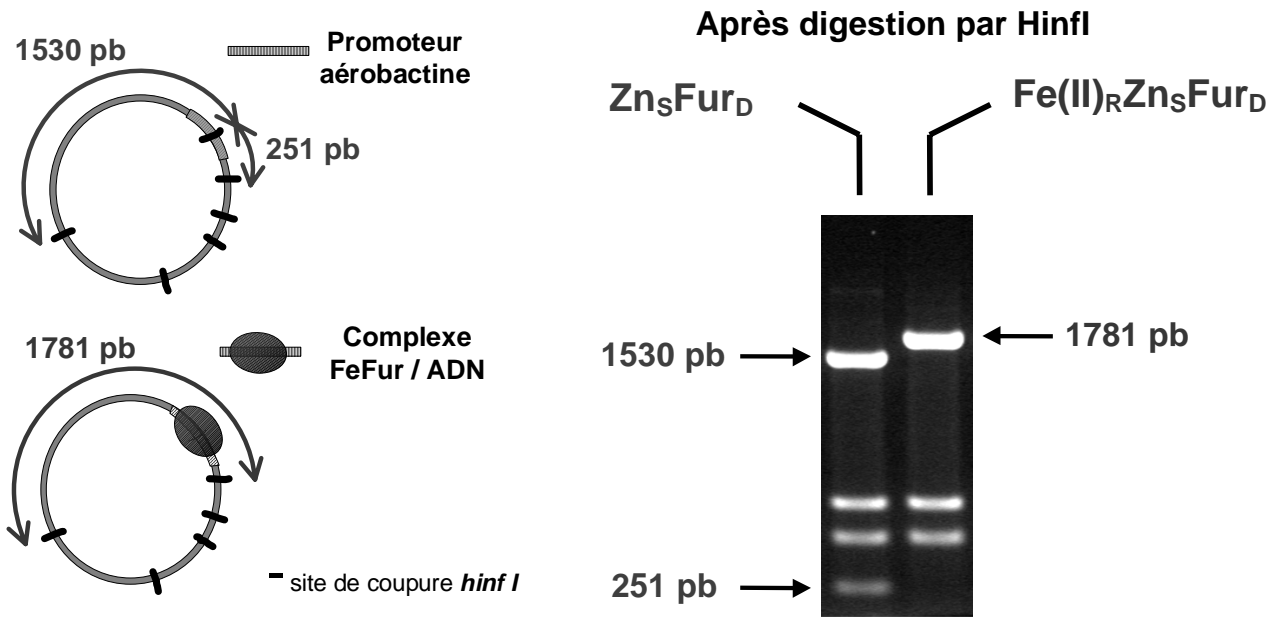
Figure VI.1 : Test de protection à la coupure par HinfI .
