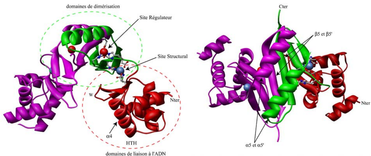
Figure I.26 : Structure cristallographique du dimère de Pseudomonas aeruginosa FUR ayant incorporée du zinc dans le site régulateur ( Zn_RZn_SFUR_D ). Une sous-unité est représentée en magenta. Dans l'autre sous-unité, le domaine de liaison à l'ADN (en rouge) est constitué d'un motif hélice-coude-hélice ailé dans lequel \alpha 4 est l'hélice d'interaction avec l'ADN. Le domaine de dimérisation (en vert) est formé d'un long brin béta ( \beta 5 ) et d'une hélice ( \alpha 5 ) à l'origine des interactions inter-sous unité. Le zinc du site structural est représenté en bleu et celui du site régulateur en rouge.
