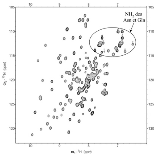
Figure III.2 : Spectre HSQC ^1\text{H} - ^{15}\text{N} de \text{Zn}_5\text{FUR}_D à 2,6 mM dans MOPS 100 mM KCl 500 mM pH 7.5 DTT 10 mM à 298 K. Le spectre montre une bonne dispersion des résonances indiquant que la protéine est structurée. On dénombre \sim 150 pics sans compter les \text{NH}_2 des chaînes latérales des Asn et Gln correspondant approximativement au nombre de résidus par monomère indiquant que le dimère est symétrique.
