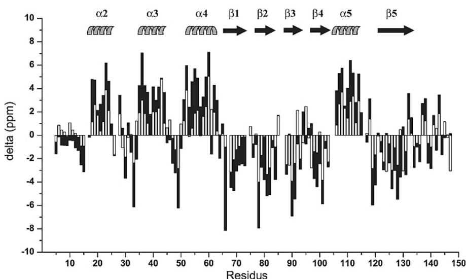
Figure III.5 : Superposition des valeurs de déplacement chimique secondaire (delta = \delta_{\text{exp}} - \delta_{\text{random coil}} ) obtenues pour les noyaux CO (barres vides) et C \alpha (barres pleines) du dimère. Plusieurs résidus successifs ayant un delta positif sont organisés en hélice \alpha et plusieurs résidus successifs ayant un delta négatif sont organisés en brin \beta . La troisième hélice est l'hélice supposée de reconnaissance de l'ADN.
