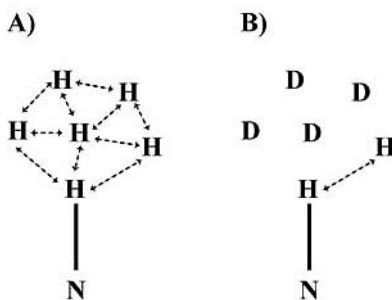
Figure II.4 : Diminution de la densité de proton due à la deutération et expliquant la diminution de la diffusion de spin. Les flèches en pointillés correspondent aux interactions ^1\text{H} - ^1\text{H} à l'origine de la diffusion de spin. (reproduit d'après (4))
