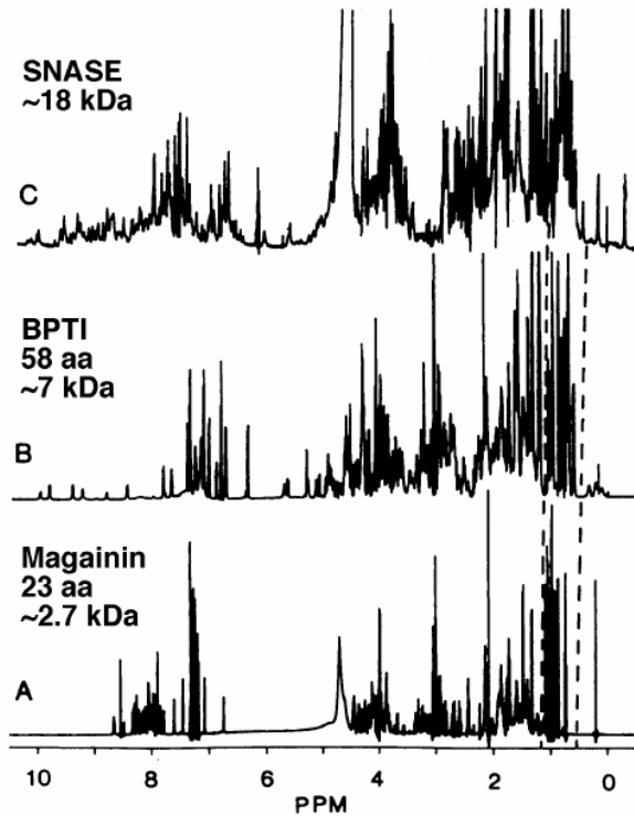
Figure II.1 : Spectre 1D 1 H de 3 protéines de tailles différentes. L'augmentation du nombre de résidus entraîne une augmentation des superpositions sur le spectre.
