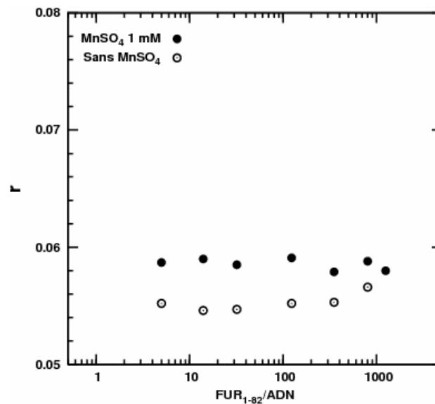
Figure VI.12 : Titration de 10 nM d'ADN consensus par des concentrations croissantes de FUR 1-82 dans du tampon MOPS 20 mM KCl 125 mM MgSO 4 12 mM dIdC 10 µg.mL -1 pH 7 en présence ou non de 1 mM de MnSO 4 1 mM.
