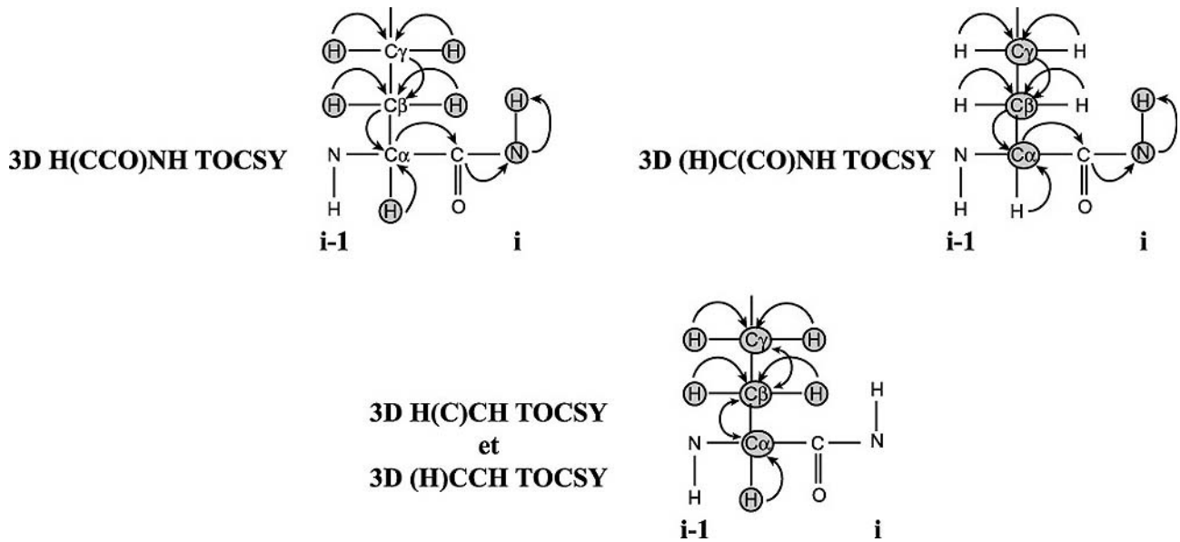
Figure II.10 : Principe des expériences permettant l'attribution des chaînes latérales.
