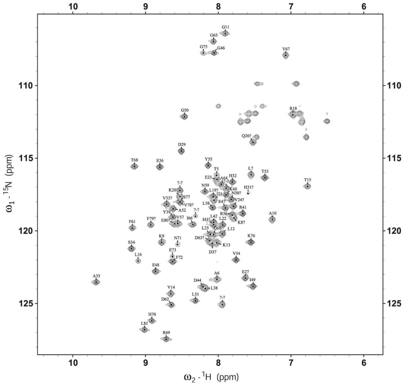
Figure VI.14 : Spectre ^1\text{H} - ^{15}\text{N} HSQC enregistré à 600 MHz de \text{FUR}_{1-82} à 1.8 mM dans MOPS 100 mM KCl 500 mM pH 7.5 avec l'attribution déduite de l'attribution du monomère.
