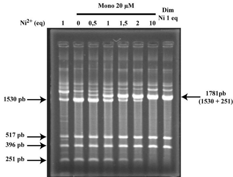
Figure VI.4 : Test d'activité de protection à la coupure par HinfI du monomère en présence de concentrations croissantes de Ni 2+ . 50 nM de plasmide pDT10 ont été incubés avec 20 μM de monomère.
