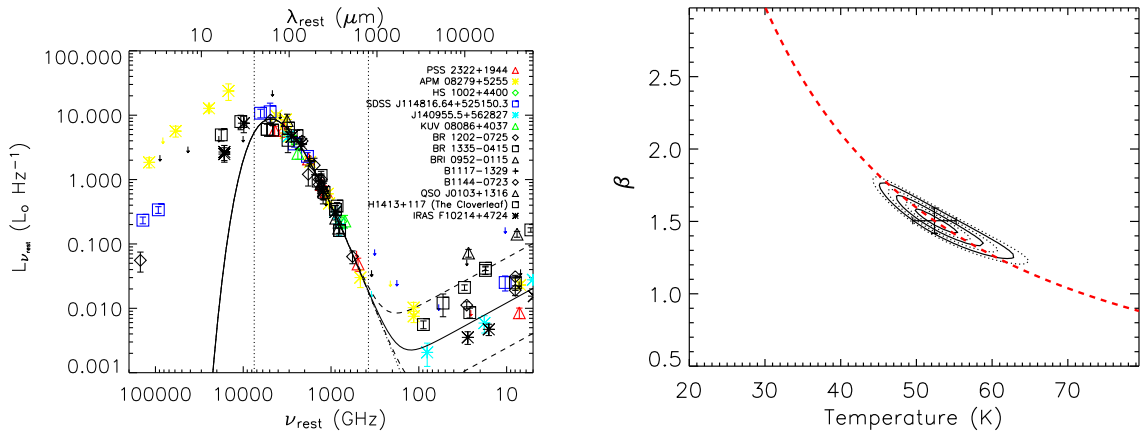
FIG. 2.3 – Gauche : Distribution spectrale d'énergie combinée des quasars à grand décalage spectral pour les 6 quasars observés à 350 \mu\text{m} de ce chapitre et les sources discutées dans Benford et al. (1999) et Priddey & McMahon (2001). La ligne continue présente le meilleur ajustement sur les données comprises entre les deux lignes pointillées verticales. L'émission radio a été extrapolé à partir de la luminosité infrarouge lointain en suivant la corrélation infrarouge radio (et sa dispersion - tiret pointillée) vu dans les ULIRGs locaux (voir texte). Droite : Contours iso- \chi^2 dans le plan \beta - T_{\text{dust}} correspondants au meilleur ajustement présenté à gauche. Les contours présentent les incertitudes à 1,2,et 3\sigma .
