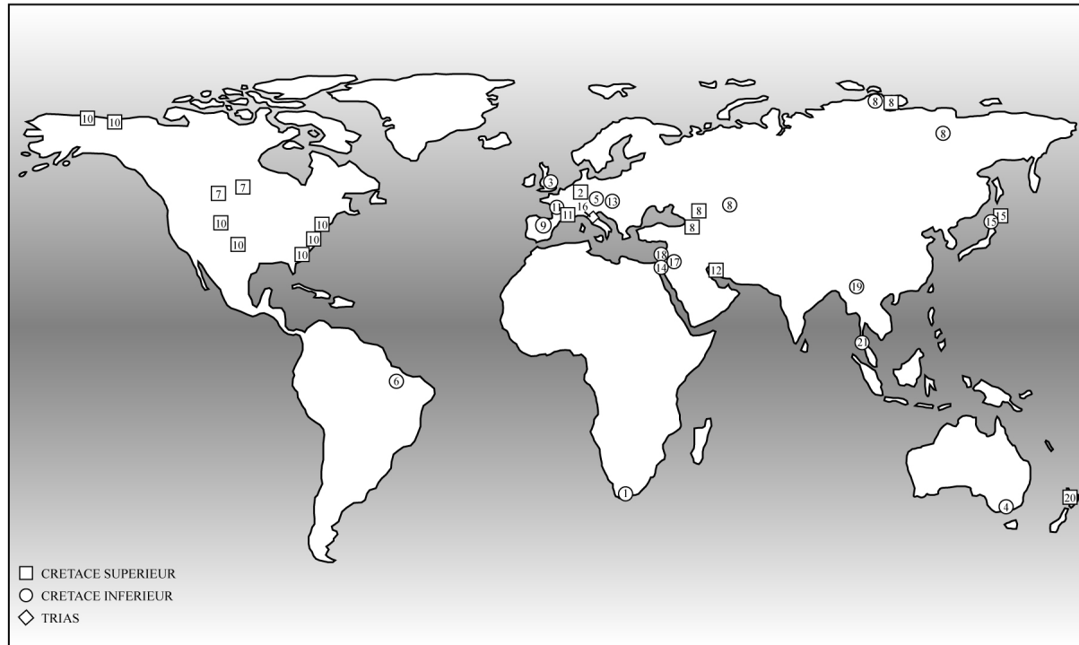
Fig. 4. Localisation des gisements d'ambre dans le monde. Les numéros correspondent aux gisements décrits dans le texte pages 6 à 10.
