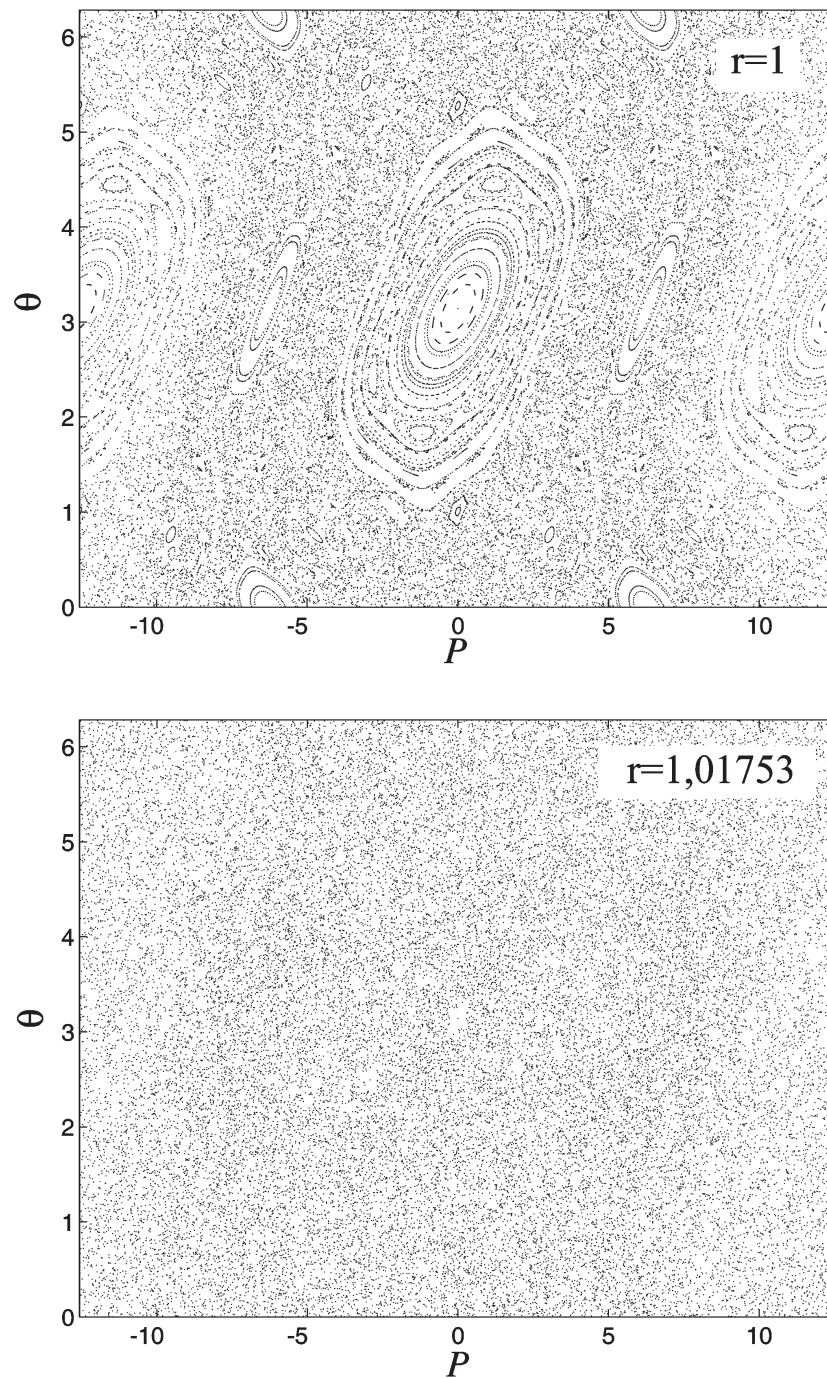
Figure 3.5: Portraits de phase classiques de système bicolore (modulation de phase) obtenus avec K = 2,5 dans les cas où r = 1 et r = 1,01753 . Alors que des îlots de stabilité sont encore très visibles dans le cas périodique, ils ont déjà disparu dans le cas quasi-périodique. La destruction de la périodicité facilite la destruction des trajectoires stables.
