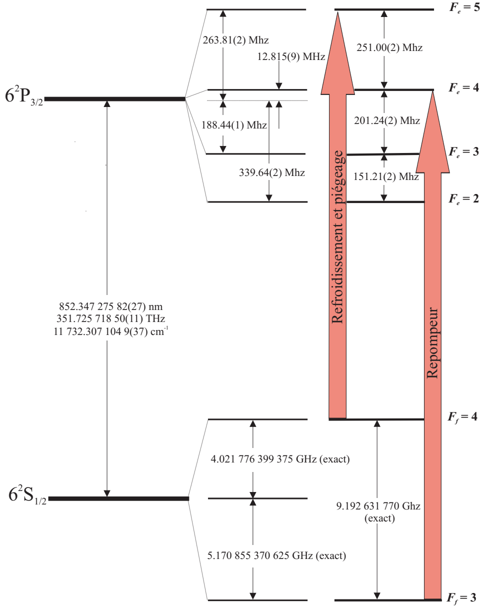
Figure 2.2: Structure hyperfine de la transition D_2 du césium. Les états 6^2S_{1/2} sont dits fondamentaux et les états 6^2P_{3/2} excités. Le cycle de fluorescence pour le refroidissement fait intervenir les niveaux |F_f = 4\rangle et |F_e = 5\rangle . Les atomes ayant suivi le chemin |F_f = 4\rangle \rightarrow |F_e = 4\rangle \rightarrow |F_f = 3\rangle sont récupérés par un laser repompeur de fréquence |F_f = 3\rangle \rightarrow |F_e = 4\rangle .
