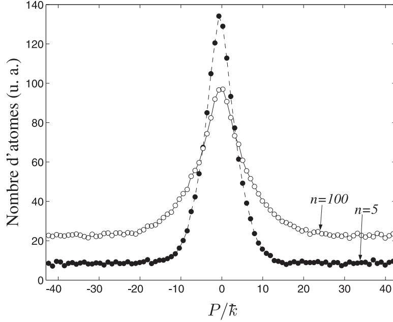
Figure 2.12: Deux distributions d'impulsions obtenues avec K_{moy} = 8,5 et \bar{k} = 3,46 pour n = 5 et n = 100 . Elles reposent toutes deux sur un signal de fond causé par la détection d'atomes ayant subi une émission spontanée. A l'augmentation de ce fond correspond une diminution de l'aire de la distribution d'impulsions. Un traitement de base des données consiste à leur soustraire ce fond.
