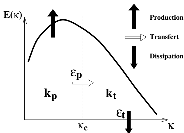
FIG. 1.1 – Schéma de base - découpage du spectre en deux zones.
