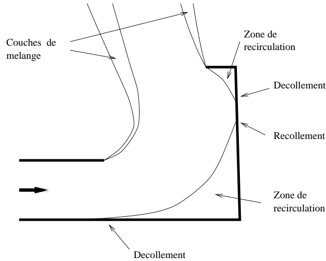
FIG. 3.3 – Représentation schématisée des phénomènes physiques présents dans l'inverseur de poussée à bord de déviation plat.
