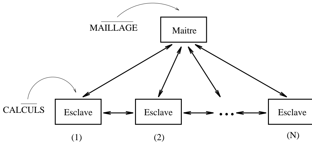
FIG. C.2 – Architecture "Maître-Esclave" de l'algorithme parallèle.
