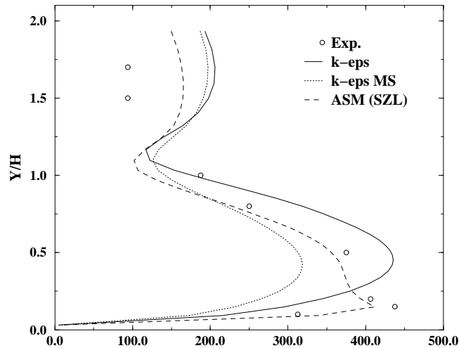
FIG. 1.7 – Profils de la viscosité turbulente en amont du point de recollement X = X_r - 2h .
