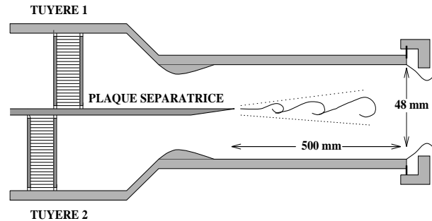
FIG. 2.1 – Montage expérimental [88].
