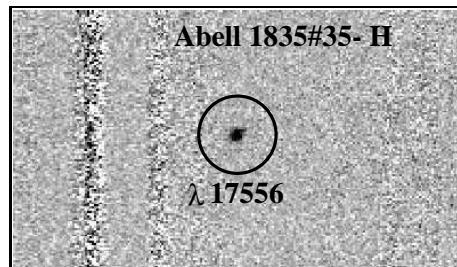
Fig. 4.40: Agrandissement de la région du spectre bidimensionnel autour de la raie H_\alpha pour le candidat A1835#35. Cette raie est très bien détectée, alors que celle de de l’azote ( [N_{II}] , prédite à \lambda = 17645 \text{ \AA} ) n’est pas visible.
