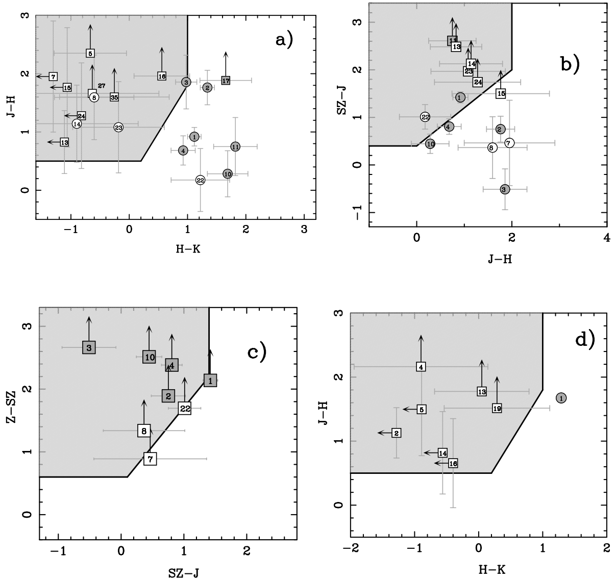
Fig. 4.19: Diagrammes couleur-couleur observés représentés dans les filtres du proche-infrarouge : pour Abell 1835 dans les bandes (a) J-H-K s , (b) SZ-J-H s et (c) Z-SZ-J, pour AC 114 dans les bandes (d) J-H-K s . Les cercles représentent les sources détectées dans les trois filtres, les carrés dans deux filtres uniquement (la flèche indique alors la limite supérieure ou inférieure sur la couleur). Les symboles colorés correspondent aux objets satisfaisant au critère des EROs. Les barres d'erreur présentées sont calculées avec la formule 4.11.
