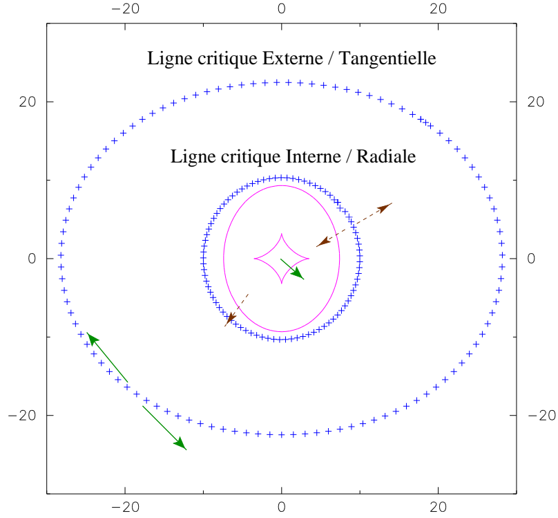
Fig. 1.21: Formation d'images multiples pour le modèle de masse PIEMD. On distingue deux lignes critiques théoriques (croix) : la ligne interne (ou radiale ) et la ligne externe (ou tangentielle ). Les lignes caustiques correspondantes (trait plein) ont une forme d'ellipse et d'astroïde, respectivement. Une source coupant la ligne caustique radiale (flèches en tirets) formera une paire d'images presque symétriques, ou arc radial dans la direction opposée au centre. Une source coupant la ligne caustique tangentielle (flèches en trait plein) formera également une paire d'images symétriques ou arc tangentiels sur la ligne critique externe. D'après Golse (2002).
