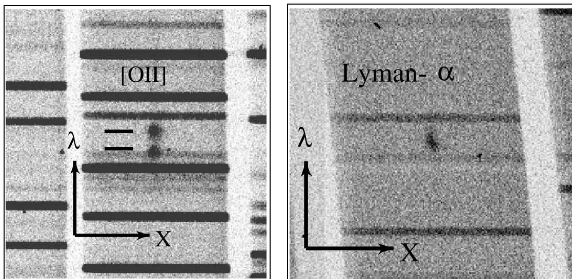
Fig. 2.22: Confirmation / Infirmer du décalage spectral des sources avec ESI : à gauche, séparation des deux composantes du doublet de [ O_{II} ]. A droite, détection d'un profil asymétrique pour la raie Lyman- \alpha .
