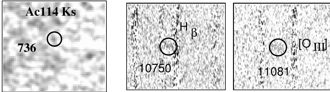
Fig. 4.42: Objet faible à z = 1.213 , observé dans la même fente que AC114#16. De gauche à droite : image en bande K_s , raies en émission de H\text{-}\beta et de [O\text{III}] dans les spectres. Une convolution avec une gaussienne de \sigma = 1 pixel a été appliquée pour la présentation.
