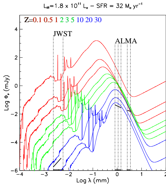
Fig. 6.3: Prédiction de spectres observés pour une galaxie formant des étoiles, avec une luminosité L \simeq 1.8 \times 10^{11} L_{\odot} et un taux de formation stellaire \text{SFR} = 32 M_{\odot} par an, pour différentes valeurs de décalage spectral (0.1, 0.5, 1.0, 2.0, 3.0, 5.0, 10.0, 20.0 et 30.0). Superposées aux courbes, les limites de détection du JWST dans le proche-infrarouge et de ALMA dans le domaine millimétrique (en traits épais). L'allure générale de la distribution spectrale en énergie entraîne un niveau de détection similaire d'ALMA pour tous les décalages spectraux. D'après Melchior et al. (2001)
