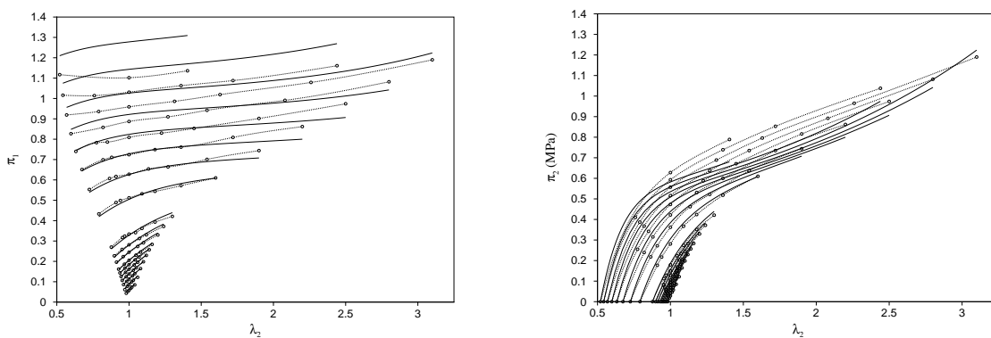
Figure A.23 : Modèle de Hart-Smith, (o) essais de Kawabata et al. , (—) modèle de Hart-Smith G = 0,145 \text{ MPa} ; k_1 = 8,42 \cdot 10^{-4} ; k_2 = 1,13 \cdot 10^{-4}
