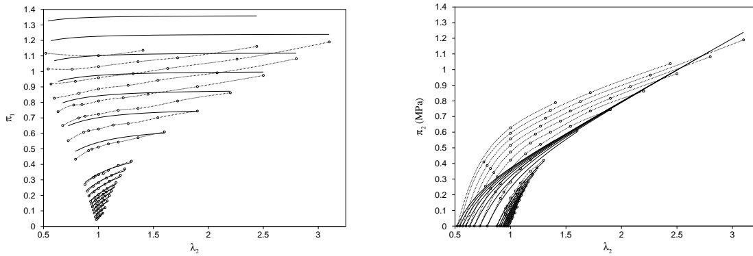
Figure A.33 : Modèle néo-hookéen de Treloar, (o) essais de Kawabata et al. , (—) modèle néo-hookéen \frac{1}{2}nkT = 0,2 \text{ MPa}
