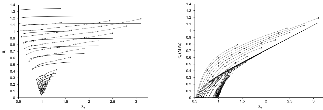
Figure A.36 : Modèle 3-chaînes, (o) essais de Kawabata et al. , (—) modèle 3-chaînes \frac{1}{2}nkT = 0,356 \text{ MPa} ; N = 365 ;
