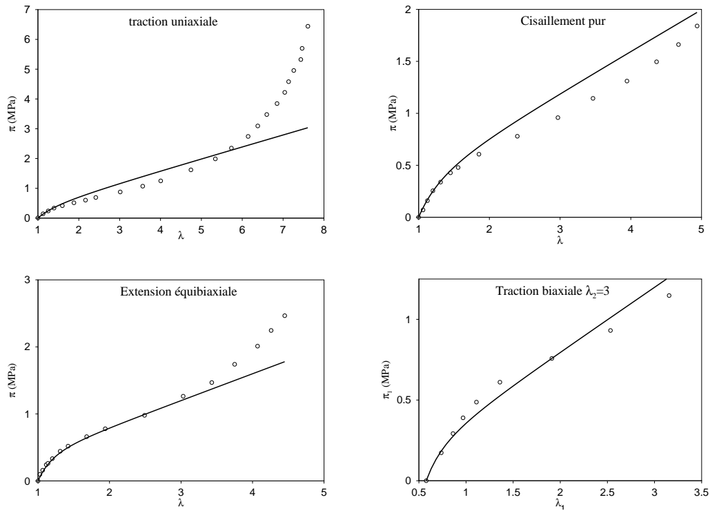
Figure A.32 : Modèle néo-hookéen de Treloar, (o) essais de Treloar, (—) modèle néo-hookéen \frac{1}{2}nkT = 0,2 \text{ MPa} ;
