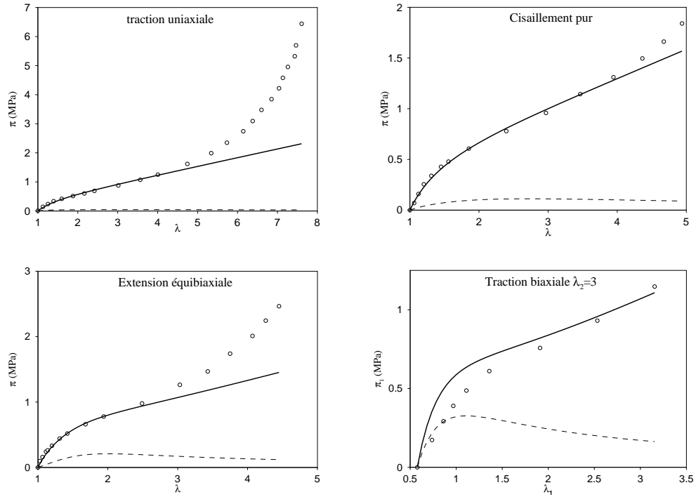
Figure A.42 : Modèle slip-link, (o) essais de Treloar, (—) modèle slip-link N_c kT = 0,3 \text{ MPa} ; N_s kT = 0,53 \text{ MPa} ; \eta = 1,9 , (- -) contribution de W_c
