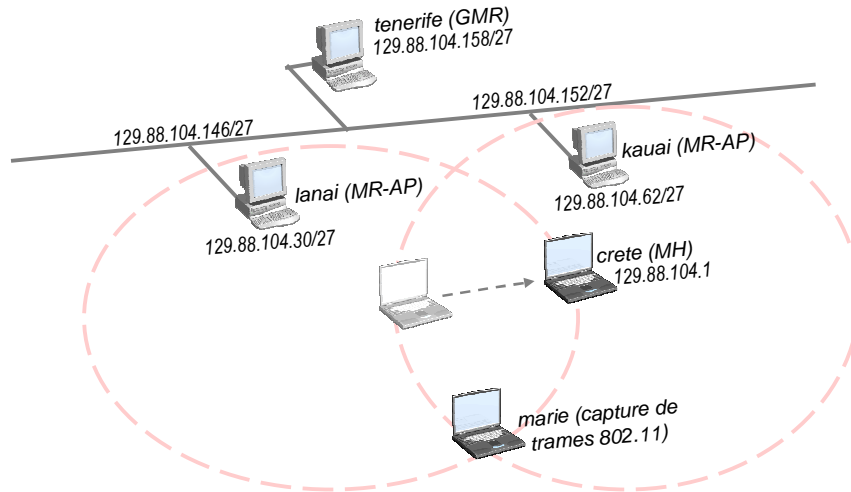
FIG. 8.6.: Configuration de la plate-forme de test
