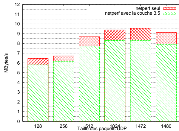
FIG. 9.4.: Surcharge introduite par la couche 3.5
