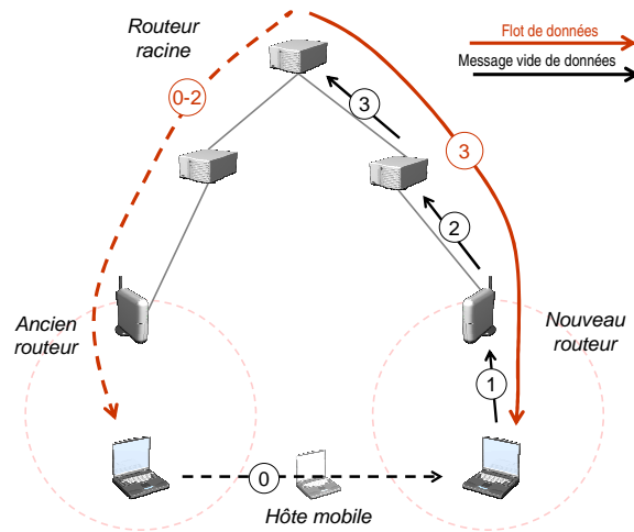
FIG. 4.4.: Le handoff dans Cellular IP
