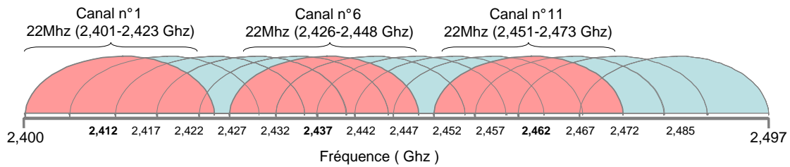
FIG. 7.1.: Les canaux de transmission dans 802.11b
