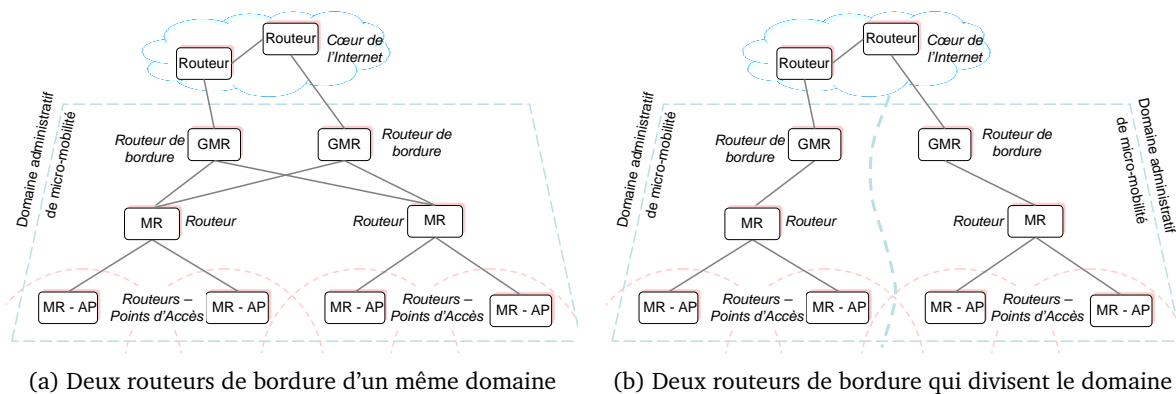
FIG. 8.2.: Domaines de mobilité avec plusieurs routeurs de bordure
