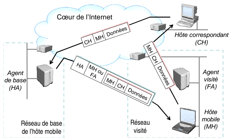
FIG. 4.1.: L'architecture de Mobile IP
