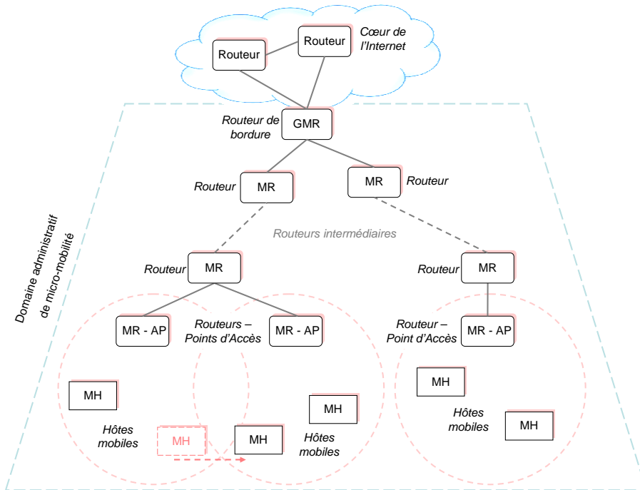
FIG. 8.1.: La topologie standard du domaine de micro-mobilité
