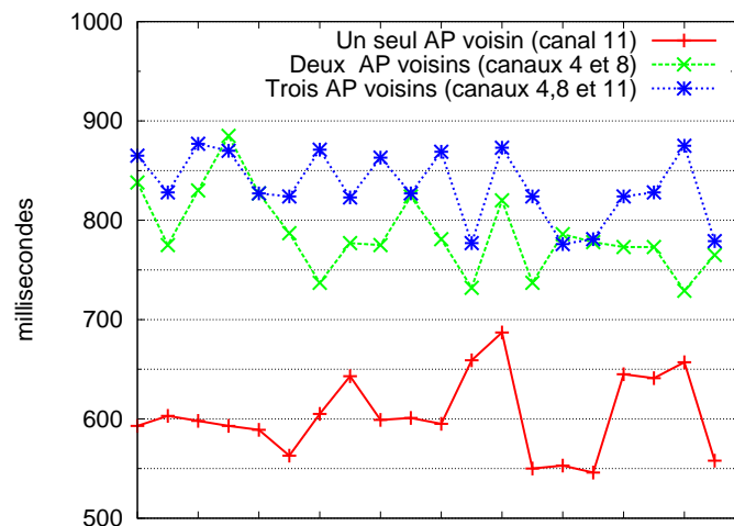
FIG. 7.9.: Le temps de détection en fonction du nombre des points d'accès voisins
