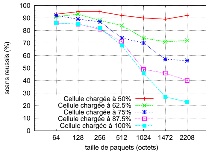
FIG. 7.11.: Taux de réussite des scans en fonction du volume de trafic
