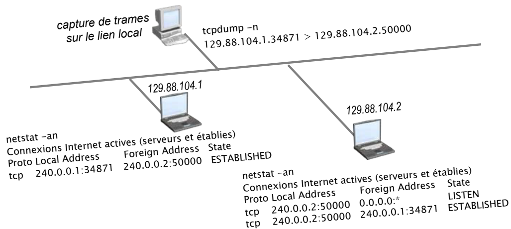
FIG. 9.3.: Fonctionnement de la couche 3.5
