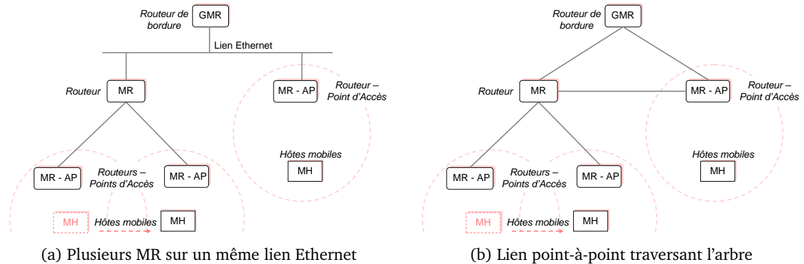
FIG. 8.3.: Topologies contenant des boucles
