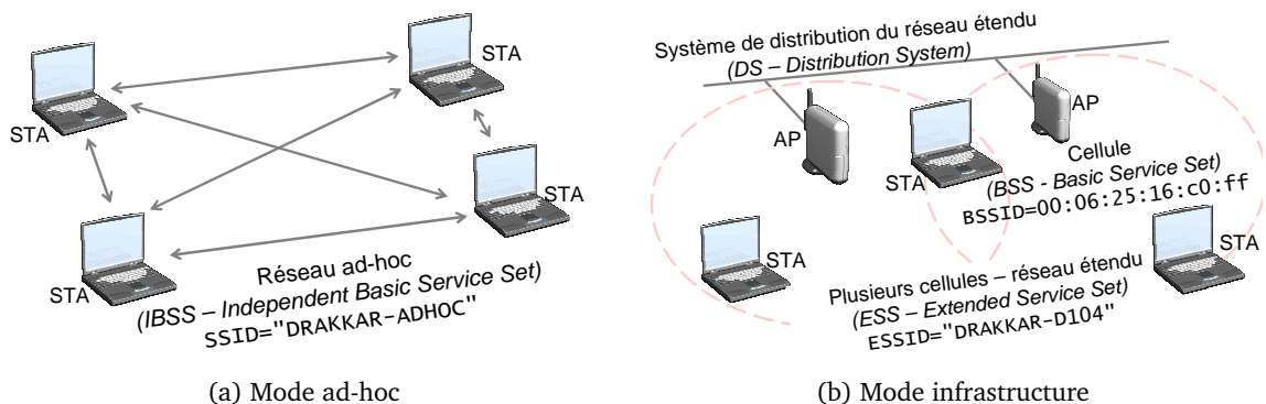
FIG. 7.2.: L'architecture d'un réseau sans-fil
