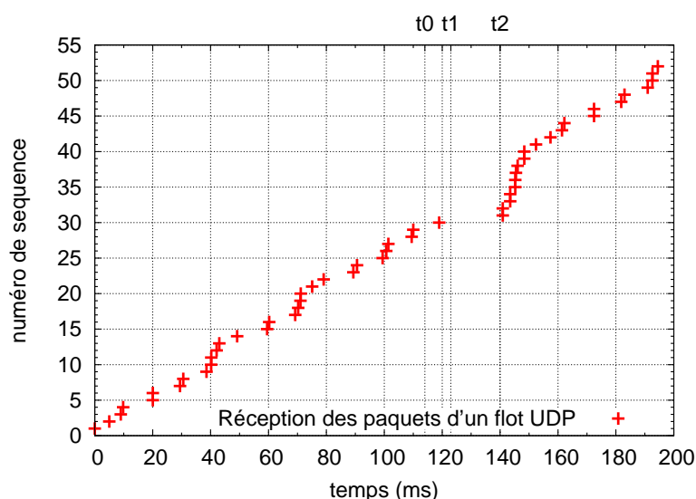
FIG. 8.9.: Capture du flot UDP lors du handoff
