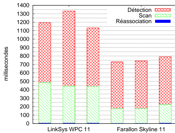
FIG. 7.10.: Comparatif des délais des trois phases du handoff
