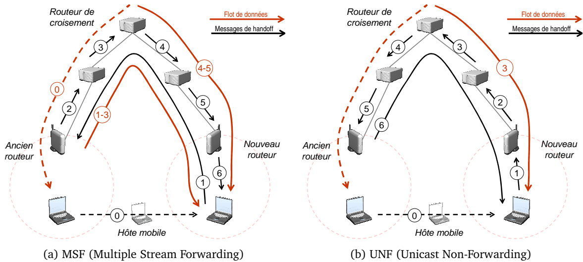
FIG. 4.3.: Le schémas de handoff dans HAWAII
