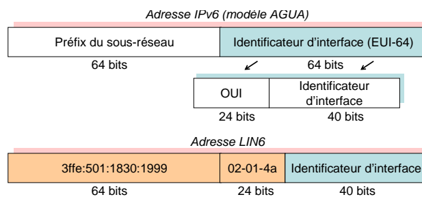
FIG. 4.6.: La structure des adresses LIN6
