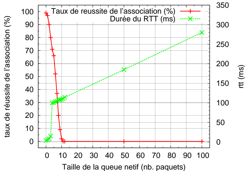
FIG. 7.12.: Taux de réussite de l'association dans une cellule chargée
