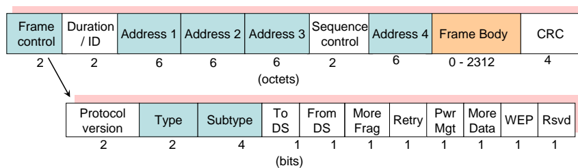
FIG. 7.3.: La structure d'une trame 802.11
