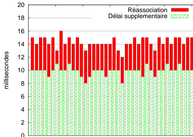
FIG. 7.13.: Délai de la réassociation directe
