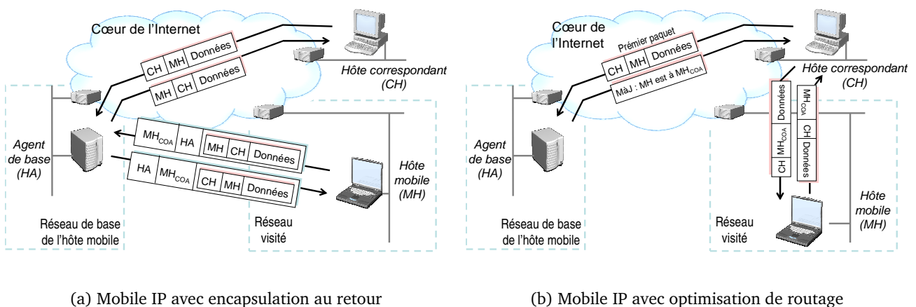
FIG. 4.2.: Extensions de Mobile IP
