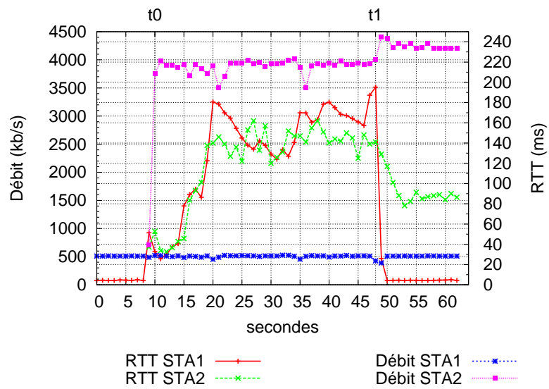
FIG. 7.15.: Équilibrage de charge : évolution du débit et de la latence
