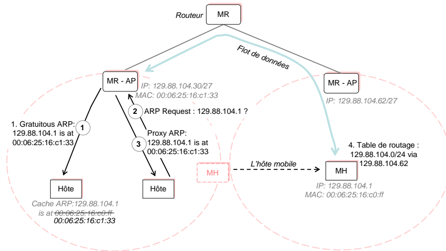
FIG. 8.4.: La communication avec les hôtes de l'ancien sous-réseau
