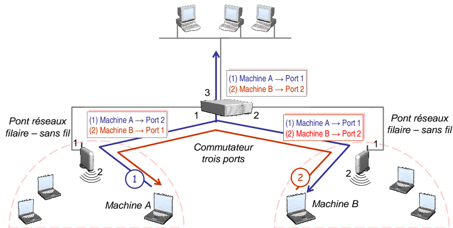
FIG. 3.3.: Les équipements actifs au niveau liaison
