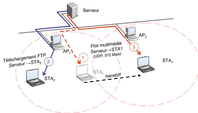
FIG. 7.14.: Configuration de test
