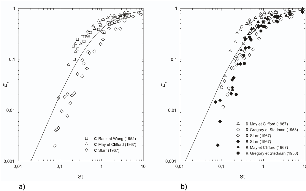
FIG. 6.3 – Dépôt par impaction inertielle en a) sur cylindres isolés (C) et en b) sur obstacles plans isolés, soit des disques (D) et des rubans (R). Les traits continus correspondent à l'équation (6.31) avec \beta_c = 0,6 pour les cylindres et \beta_p = 0,4 pour les obstacles plans.
