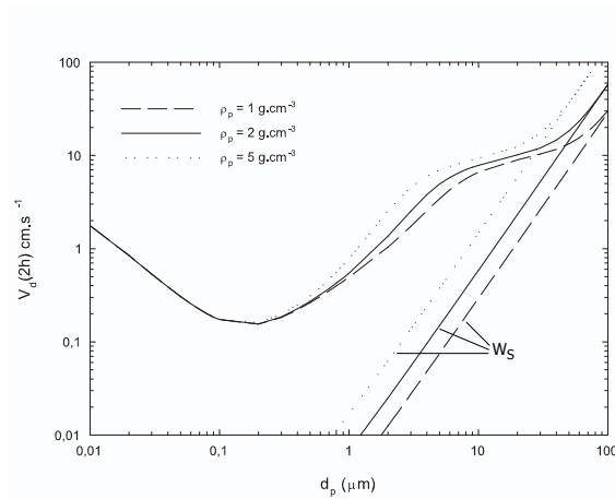
FIG. 7.33 – Sensibilité du modèle à la masse volumique de l'aérosol.
