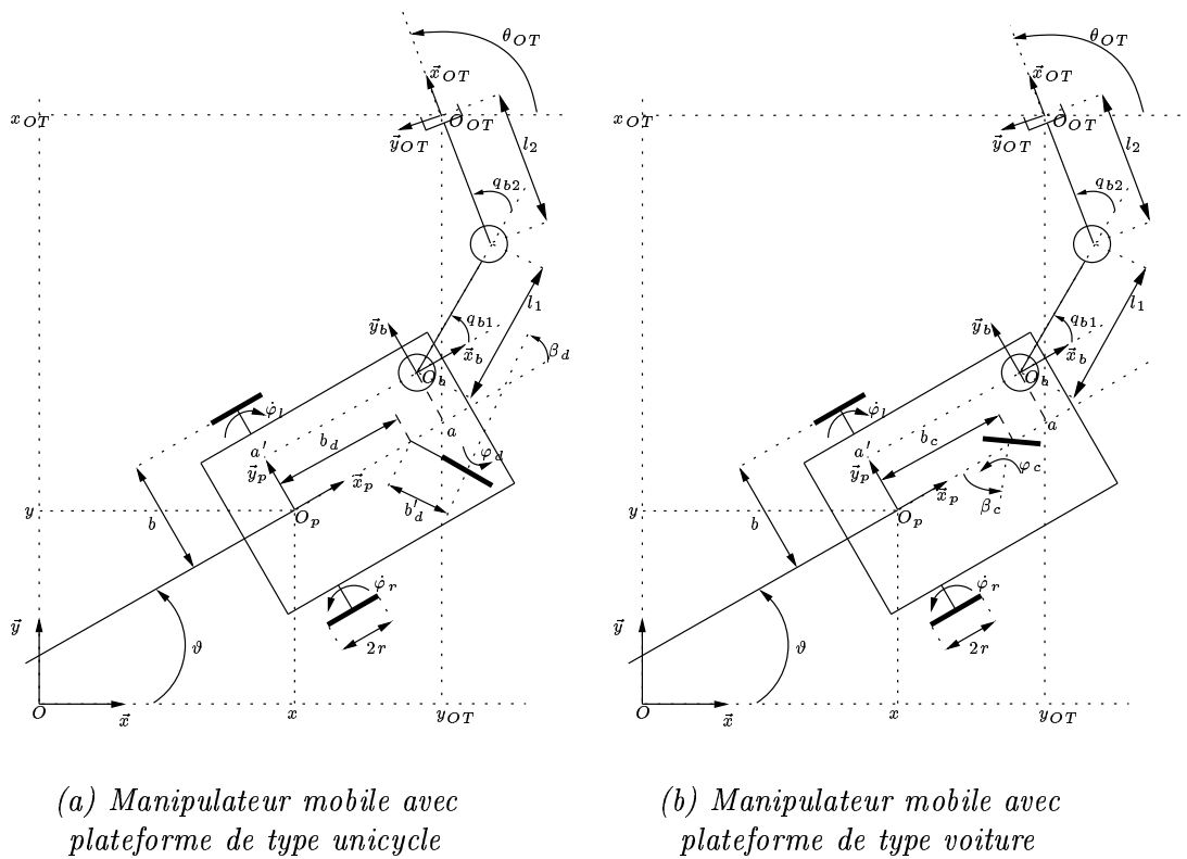
FIG. 2.5 – Deux types classiques de manipulateur mobile à roues
