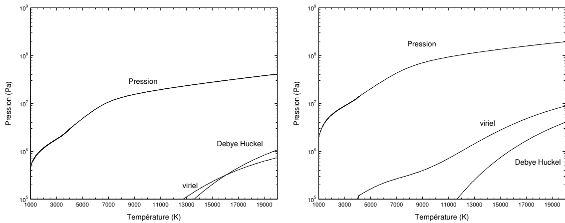
Fig. 2 : Calcul de la pression en fonction de la température dans le cas pu polyéthylène pour deux masses volumiques initiales différentes ( 1\text{kg/m}^3 et 5\text{ kg/m}^3 )
