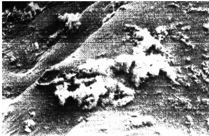
Fig. 4. : Vue au microscope électronique à balayage du cuivre sous forme d'une pellicule.
