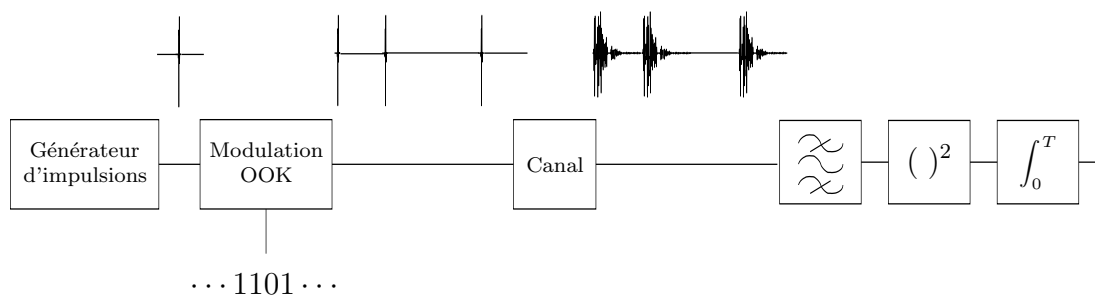
FIG. 4.4 – Système de transmission OOK non-cohérent.
