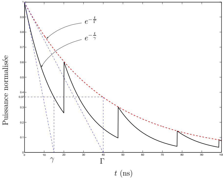
FIG. 3.13 – Représentation schématique du power delay profile .
