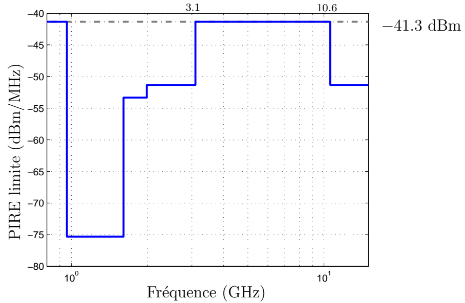
FIG. 2.1 – Masque FCC pour l'émission des signaux UWB en indoor .
