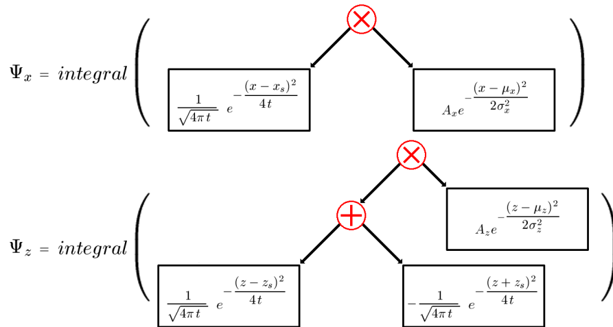
FIG. 2.2.1 – Représentation sous forme d’arbre binaire d’une solution élémentaire
