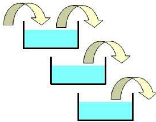
FIG. 4.1.1 – Modélisation capacitif monodirectionnel des transferts hydriques
