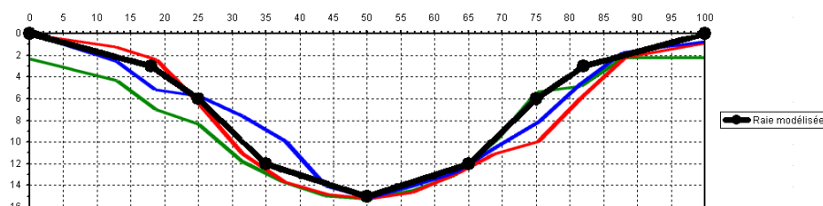
FIG. 1.2.1 – Profil de la raie modélisée
