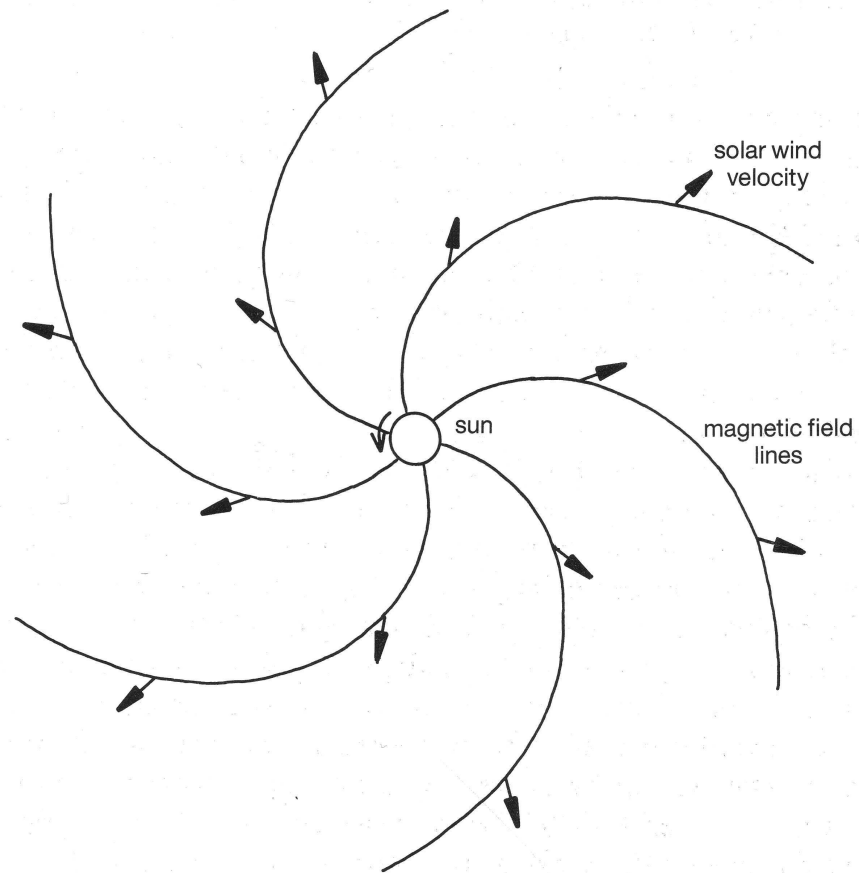
Fig. 1.15: Spirale de Parker, dessinée par les lignes de champ : elles restent connectées à la surface du Soleil pendant sa rotation. Les flèches représentent le vent solaire en expansion radiale, qui entraîne le champ magnétique avec lui (tiré de Phillips (1992)).
