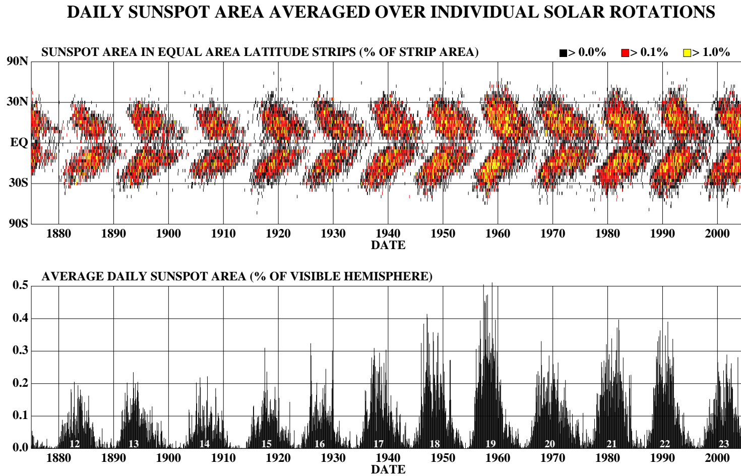
Fig. 1.10: Diagramme “papillon” : répartition en latitudes des taches observées tout au long des cycles solaires. Les taches apparaissent à une latitude d’environ 30° pendant la phase montante du cycle. Elles se rapprochent ensuite progressivement de l’équateur, où elles disparaissent, tandis que de nouvelles taches apparaissent aux hautes latitudes, au début du cycle suivant. (tiré de Hathaway (2004)).
