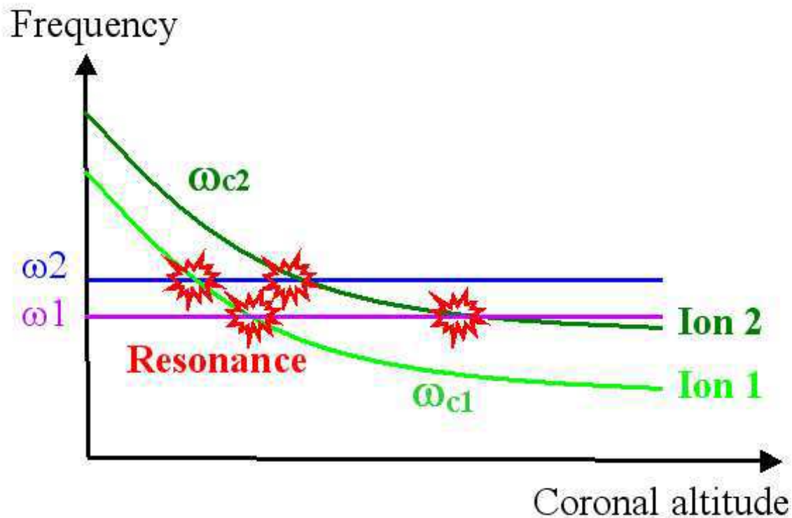
Fig. 2.4: Schéma de principe du chauffage préférentiel des espèces ioniques ayant les plus petites valeurs du rapport charge-sur-masse q/m . A mesure que l'altitude augmente dans la couronne solaire, le champ magnétique décroît, ce qui entraîne aussi la décroissance de la pulsation cyclotron \omega_{c,i} des ions (en tons de vert). Des ondes de pulsation \omega_i (bleu et violet) résonneront en premier avec les espèces ayant le plus petit q/m . Le fait que l'onde est absorbée lors de la résonance accentue cet effet, puisqu'il reste moins d'énergie à une fréquence donnée pour les autres espèces qui résonneraient à plus haute altitude (N.B. : ceci n'est qu'un schéma. La véritable condition de résonance fait aussi intervenir la vitesse, parallèle au champ magnétique, de l'ion, cf. Eq. 2.5).
