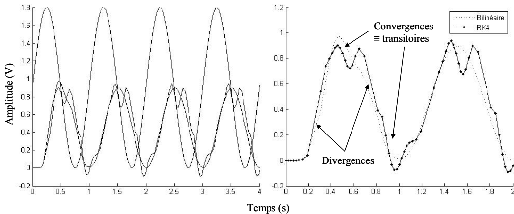
Figure 96 : Filtre de Butterworth d'ordre 10 déstabilisant la méthode RK4 (plan large et zoom)
