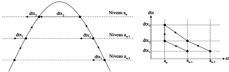
Figure 17 : Cycle hystérésis des intervalles de temps autour d'une crête
