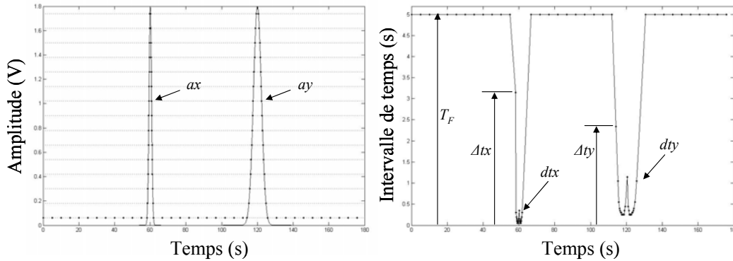
Figure 40 : Echantillonnage par traversée de niveaux de deux impulsions décalées. Des périodes inactives induisent la saturant du timer.
