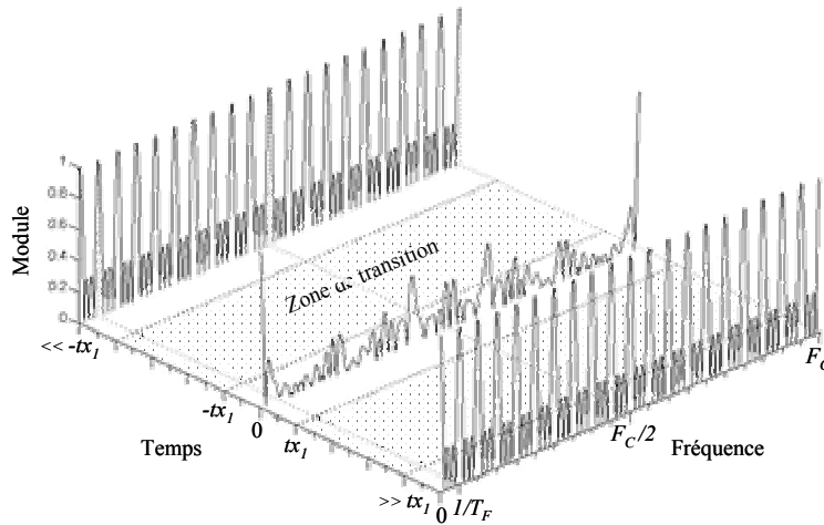
Figure 38 : Représentation temps-fréquence théorique du schéma d'échantillonnage d'un signal impulsionnel avec saturation du timer
