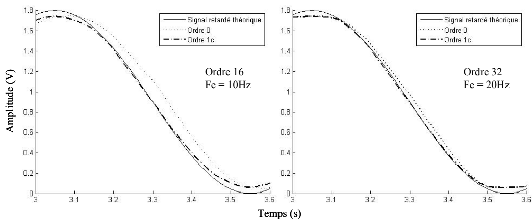
Figure 78 : Filtrages à phase linéaire d'un signal sinusoïdal
