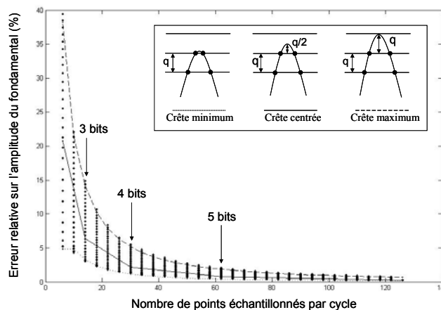
Figure 50 : Erreur relative sur l'amplitude du fondamental en fonction du nombre de points échantillonnés par cycle d'un signal sinusoïdal
