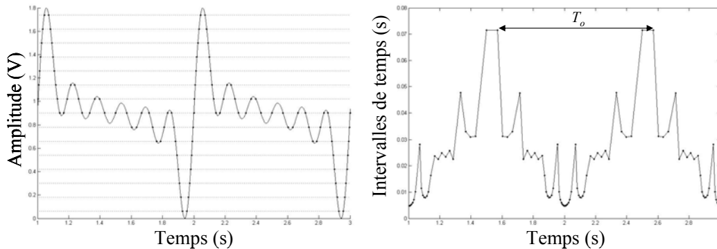
Figure 31 : Exemple d'un signal périodique non symétrique. L'échantillonnage est également non symétrique.
