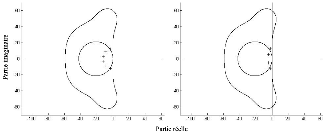
Figure 93 : Représentation dans le plan complexe analogique des pôles des filtres de Butterworth d’ordre 6 (à gauche) et de Chebyshev d’ordre 4 (à droite)
