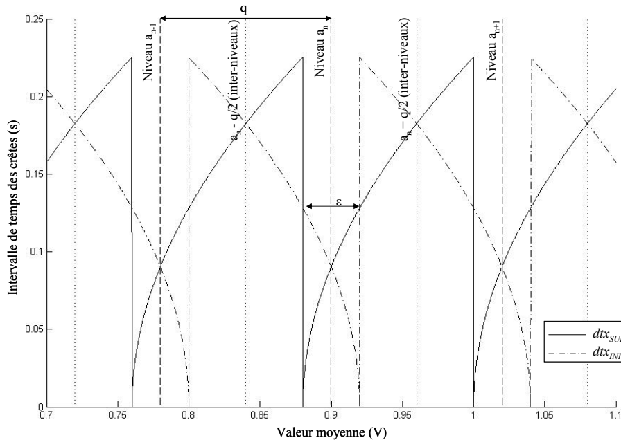
Figure 21 : Exemple d'évolution simulée des intervalles de temps en fonction de la valeur moyenne
