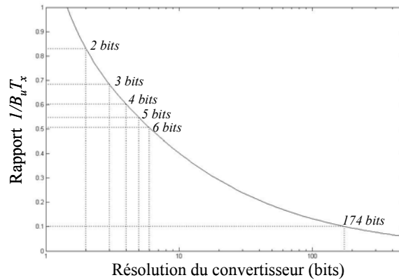
Figure 36 : Rapport de la largeur du lobe principal du schéma d'échantillonnage sur la bande passante du signal en fonction de la résolution du convertisseur
