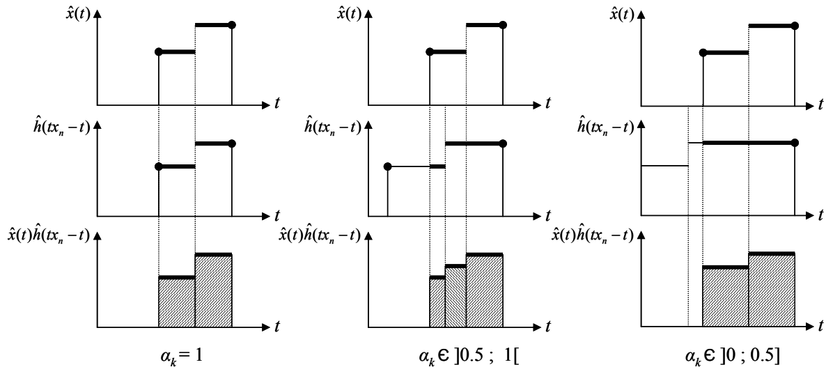
Figure 64 : Produit de convolution asynchrone d'ordre 0.5c
