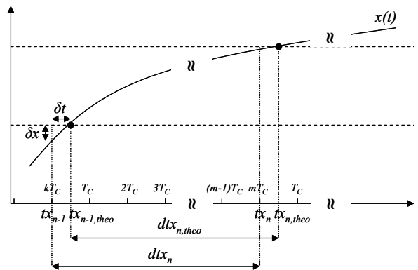
Figure 14 : Quantification du temps induite par le timer lors de la traversée d'un niveau
