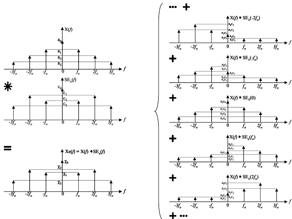
Figure 32 : Spectre d'un signal périodique échantillonné par traversée de niveaux
