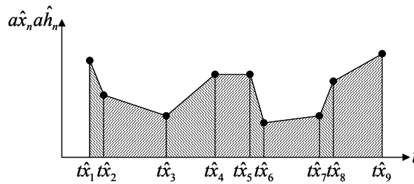
Figure 57 : Calcul simplifié de l'intégrale par multiplication des échantillons et utilisation de trapèzes élémentaires
