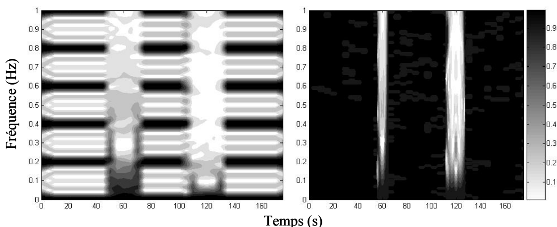
Figure 41 : Représentations temps fréquence à bande étroite (à gauche) et large bande (à droite) en lignes de niveaux du schéma d'échantillonnage de deux impulsions décalées
