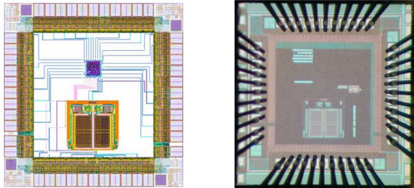
Figure 16 : Layout et photographie du convertisseur CANA
