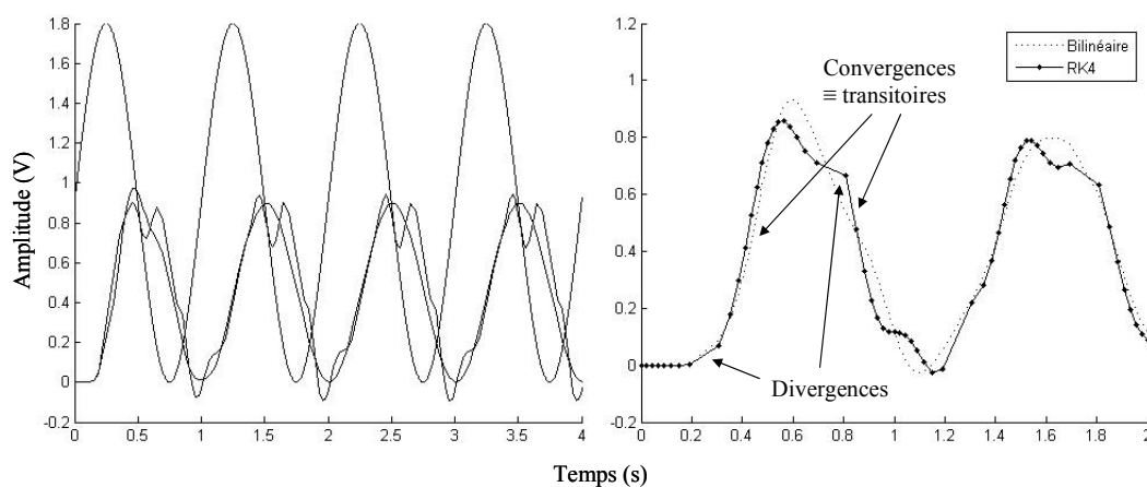
Figure 97 : Filtre de Chebyshev d'ordre 10 déstabilisant la méthode RK4 (plan large et zoom)
