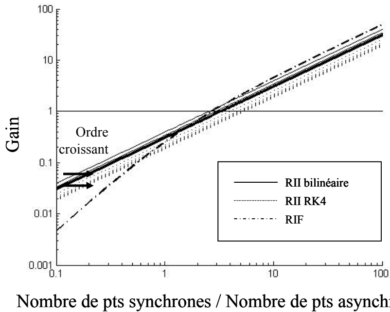
Figure 111 : Gain d'une chaîne de traitement numérique asynchrone en fonction du rapport entre le nombre d'échantillons synchrones et asynchrones. Pour le filtrage RII, les courbes de gains sont paramétrées par l'ordre du filtre. Il y a donc une série de courbes pour chaque méthode; les courbes tendent toutes vers une droite limite.
