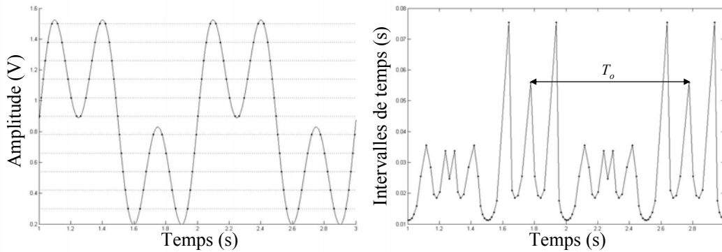
Figure 30 : Exemple d'un signal périodique symétrique échantillonné non symétriquement
