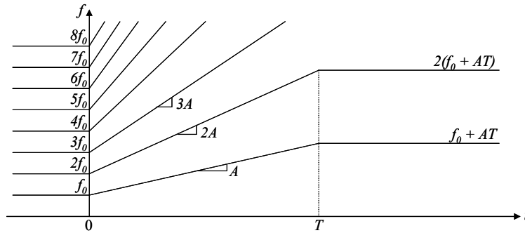
Figure 44 : Allure théorique du schéma d'échantillonnage et du spectre d'une modulation linéaire de fréquence échantillonnée
