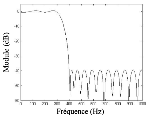
Figure 106 : Réponse en fréquence du filtre RIF
