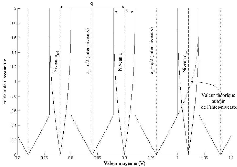
Figure 22 : Exemple d'évolution simulée du facteur de symétrie en fonction de la valeur moyenne
