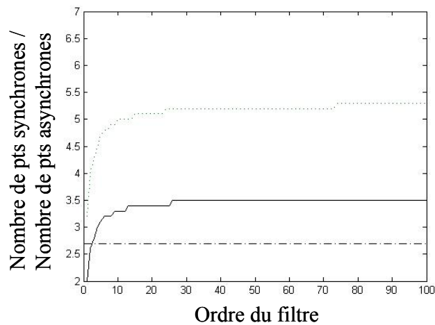
Figure 112 : Rapport minimum entre le nombre de points synchrones et le nombre de points asynchrones en fonction de l'ordre des filtres
