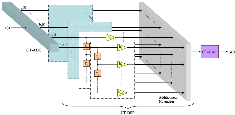
Figure 53 : Architecture de filtrage RIF à temps continu
