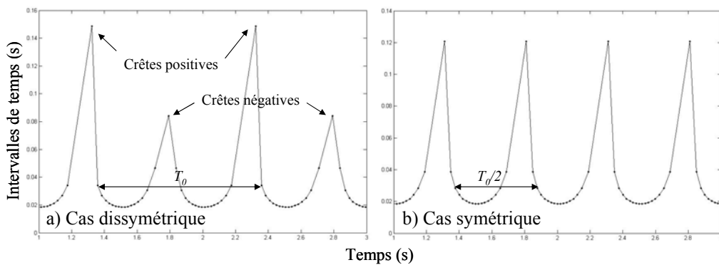
Figure 24 : Intervalles de temps d'un signal sinusoïdal échantillonné par traversée de niveaux.
