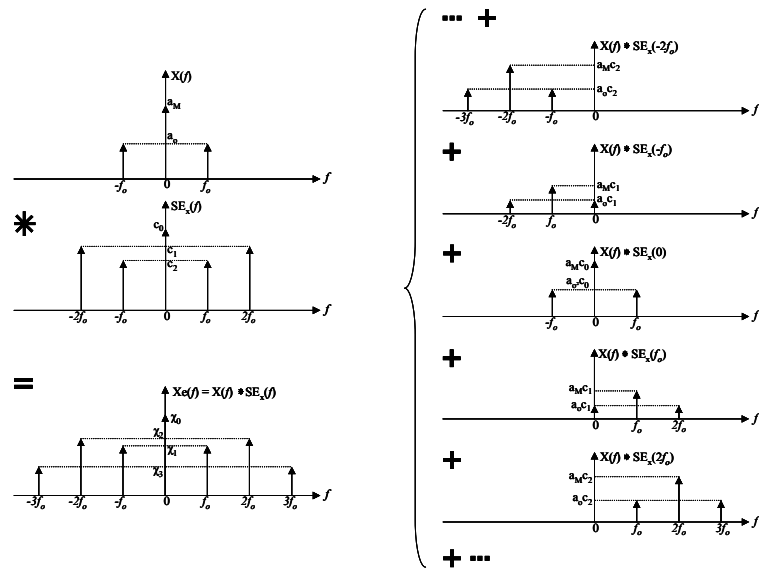
Figure 28 : Produit de convolution entre le spectre d'un signal sinusoïdal à temps continu et son schéma d'échantillonnage par traversée de niveaux
