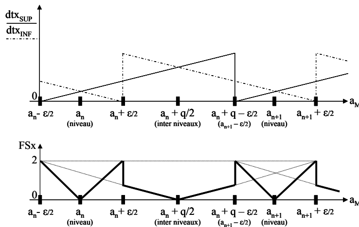
Figure 20 : Evolutions schématiques des intervalles de temps des crêtes et du facteur de symétrie en fonction de la valeur moyenne
