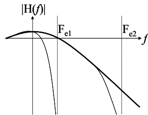
Figure 92 : Exemple de réponses en fréquence déformées par la méthode bilinéaire pour deux valeurs de fréquence d'échantillonnage (les périodisations ne sont affichées pour plus de clarté)
