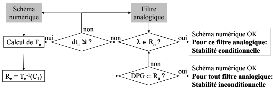
Figure 88 : Flot de conception d'un filtre numérique stable
