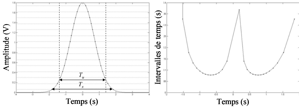
Figure 33 : Echantillonnage par traversée de niveaux d'un signal impulsionnel
