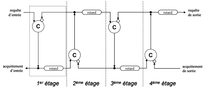
Figure 10 : Contrôle local d'un circuit Micropipeline
