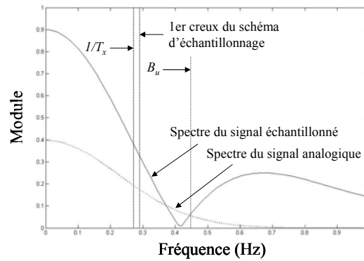
Figure 35 : Spectre d'un signal impulsionnel échantillonné par traversée de niveaux
