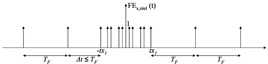
Figure 37 : Fonction d'échantillonnage d'un signal impulsionnel avec saturation du timer
