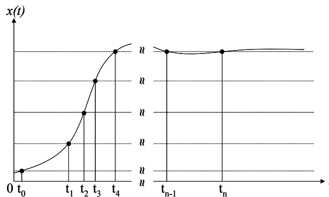
Figure 4 : Echantillonnage non uniforme par traversée de niveaux
