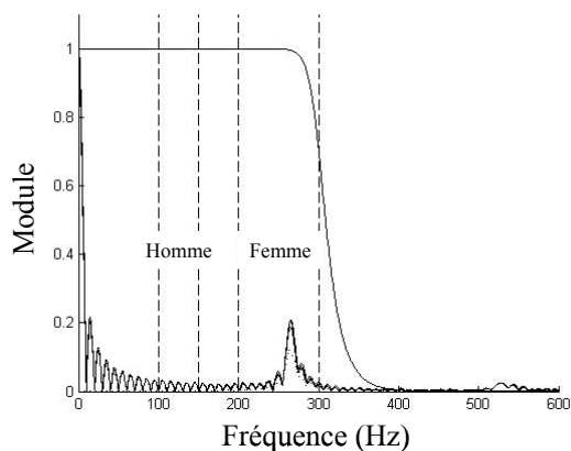
Figure 109 : Transformées de Fourier des signaux reconstruits à l'ordre 0
