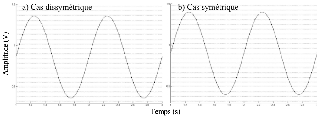
Figure 23 : Amplitude d'un signal sinusoïdal échantillonné par traversée de niveaux.
