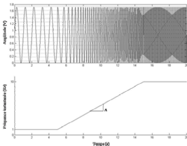
Figure 45 : Exemple de modulation linéaire de fréquence
