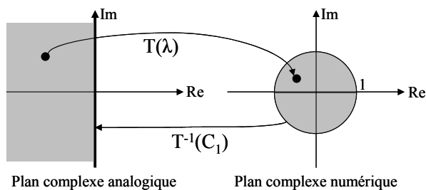
Figure 87 : Transformation du demi-plan gauche pour la méthode bilinéaire
