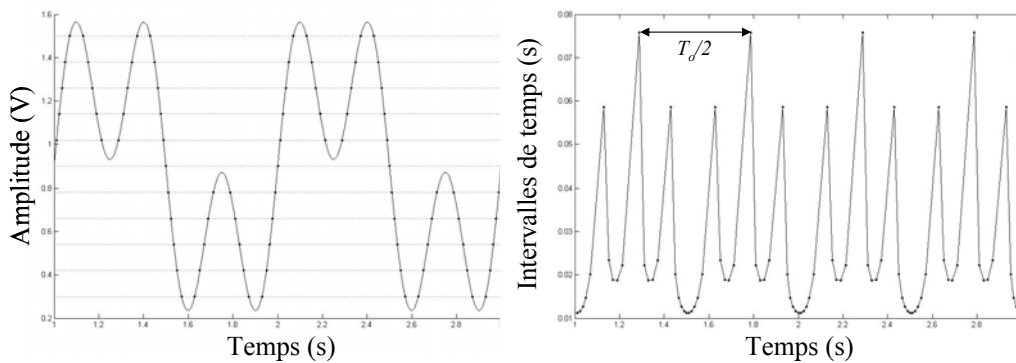
Figure 29 : Exemple de signal périodique symétrique échantillonné symétriquement
