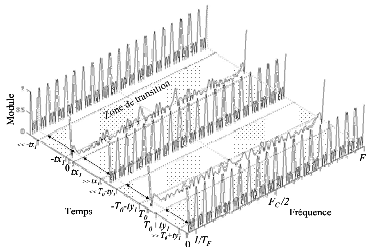
Figure 39 : Représentation temps-fréquence théorique du schéma d'échantillonnage d'un signal impulsionnel variable de période T_o avec saturation du timer
