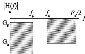
Figure 105 : Gabarit du filtre passe bas
