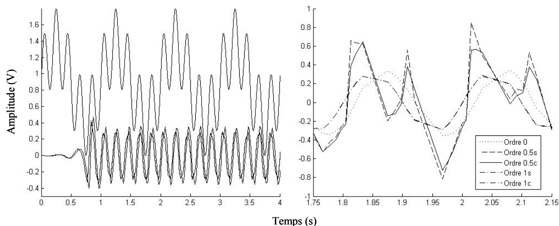
Figure 75 : Filtrage RIF passe-haut à 33 coefficients de fréquence de coupure f_c = 3\text{Hz} et échantillonnés à F_e = 20\text{Hz} selon les cinq interpolations (plan large et zoom)
