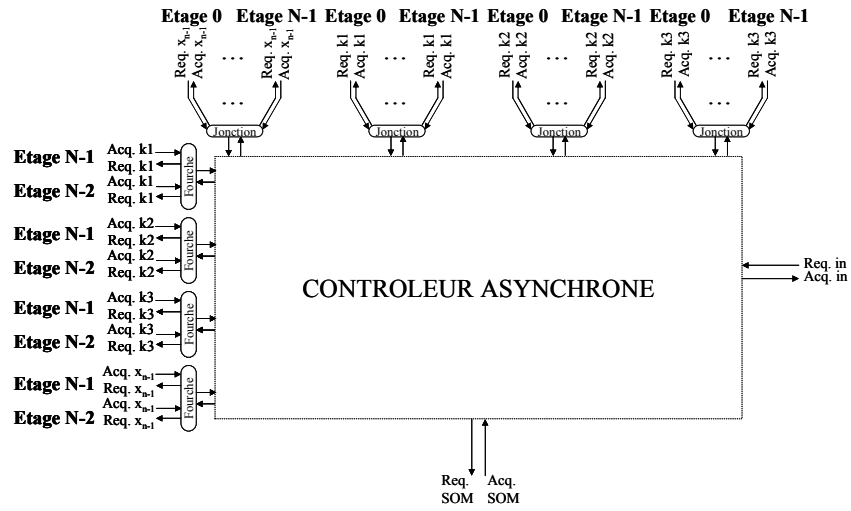
Figure 104 : Contrôleur asynchrone de la structure B utilisé par le schéma de Runge-Kutta d'ordre 4
