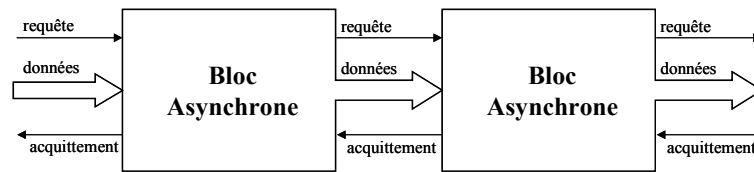
Figure 5 : Schéma fonctionnel d'un circuit asynchrone
