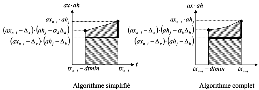
Figure 72 : Etude du pire cas de l'ordre 1
