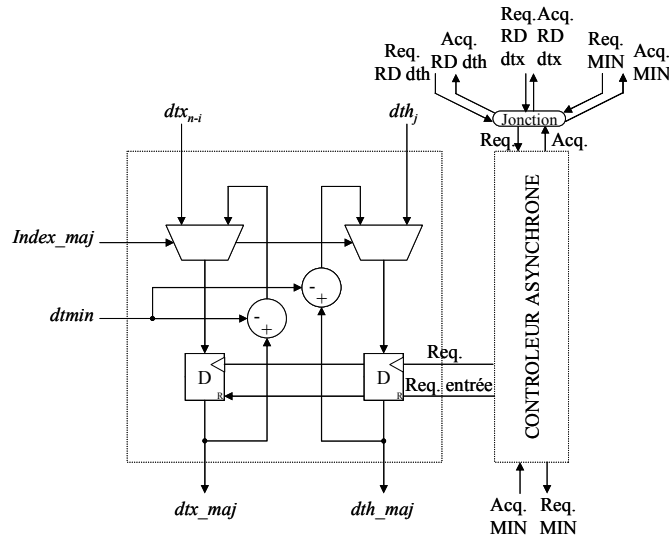
Figure 82 : Architecture du bloc MAJ : mise à jour des intervalles de temps
