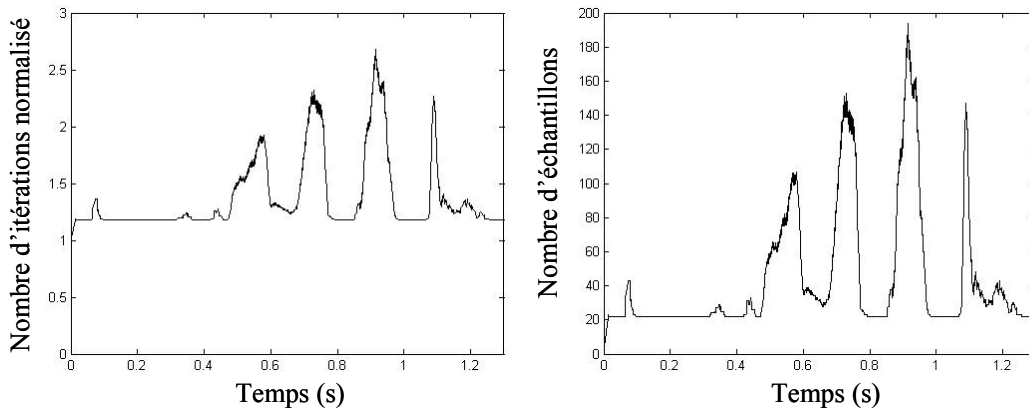
Figure 110 : Evolutions temporelles du nombre d'itérations et d'échantillons d'entrée utilisés dans le produit de convolution asynchrone.
