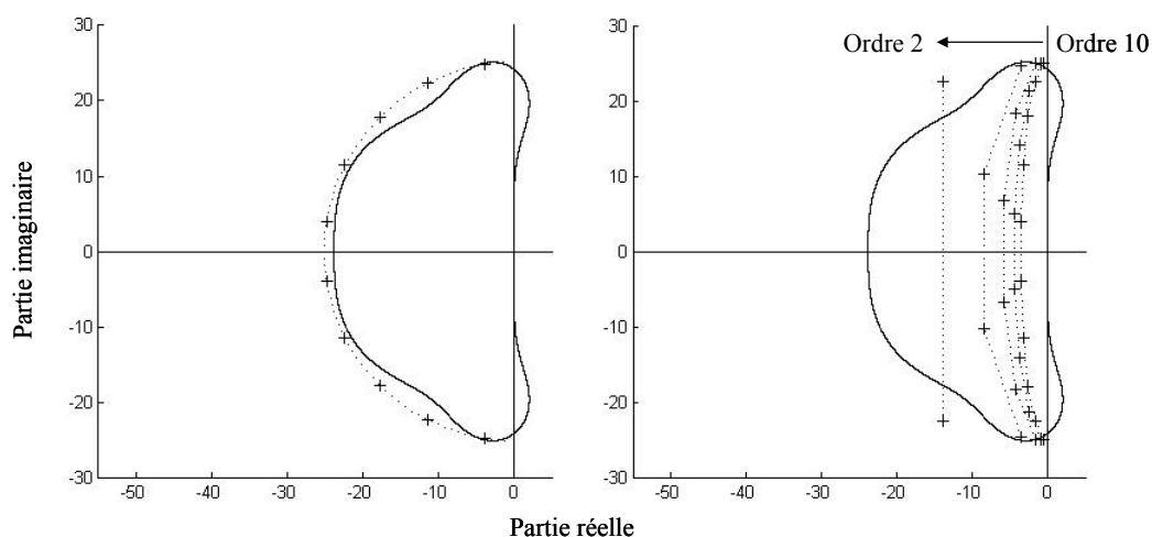
Figure 98 : Représentation dans le plan complexe analogique des pôles des filtres de Butterworth d'ordre 10 (à gauche) et de Chebyshev pour les ordres 2 à 10 (à droite)
