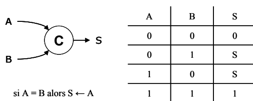
Figure 8 : Symbole et table de vérité d'une porte de Müller à 2 entrées
