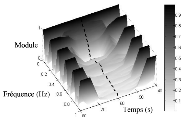
Figure 42 : Transition entre le peigne de Dirac en fréquence et le schéma d'échantillonnage d'une impulsion
