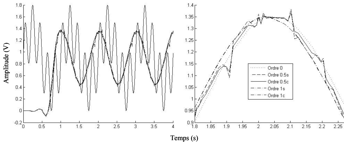
Figure 74 : Filtrage RIF passe-bas à 33 coefficients de fréquence de coupure f_c = 3\text{Hz} et échantillonnés à F_e = 20\text{Hz} selon les cinq interpolations (plan large et zoom)
