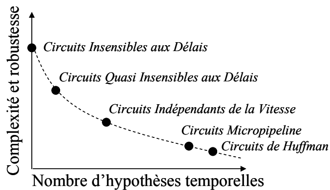
Figure 9 : Catégories de circuits asynchrones
