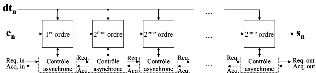
Figure 99 : Structure cascadée d'un filtre RII utilisant la méthode bilinéaire
