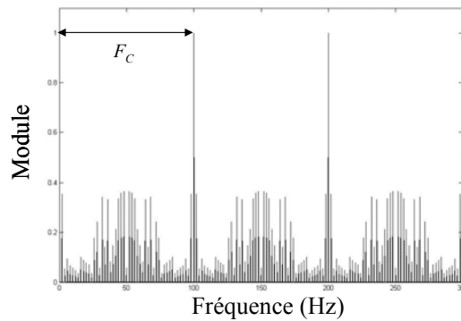
Figure 26 : Plan large du schéma d'échantillonnage d'un signal sinusoïdal
