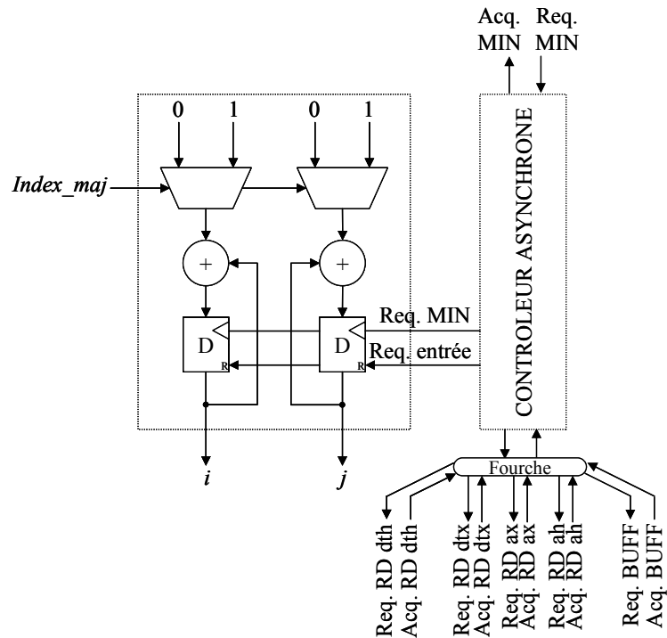
Figure 83 : Architecture du bloc ADD : mise à jour des adresses des registres
