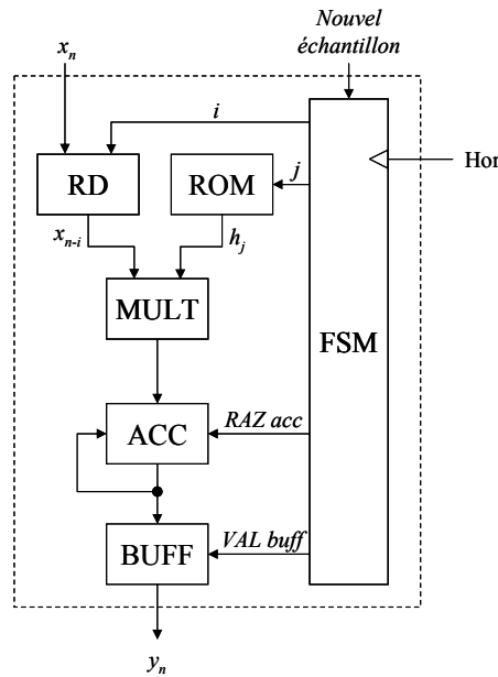
Figure 79 : Structure itérative d'un filtre RIF dans le cas uniforme
