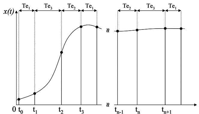
Figure 1 : Echantillonnage non uniforme à P fréquence ( P = 3 )
