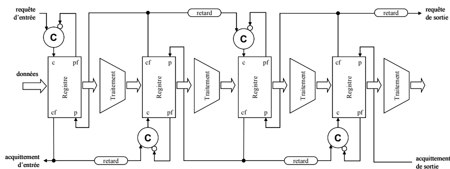
Figure 11 : Circuit Micropipeline avec traitement
