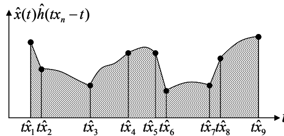
Figure 58 : Calcul complet de l'intégrale par multiplication des fonctions interpolées
