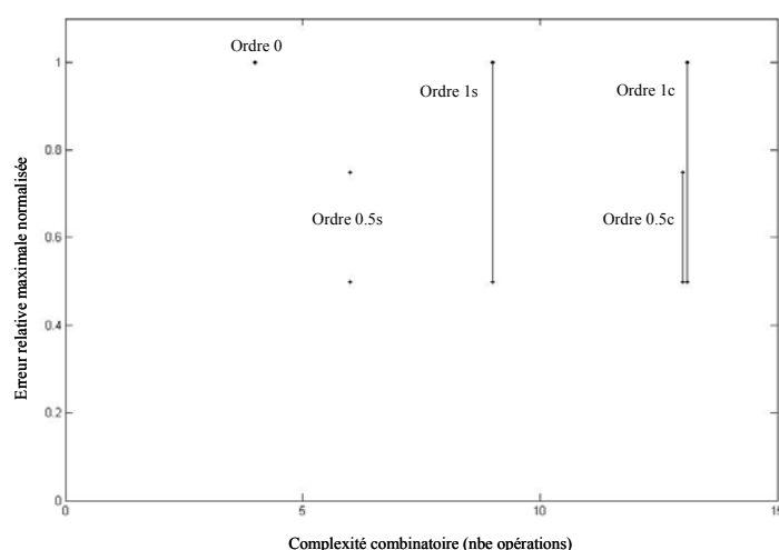
Figure 73 : Représentation de l'erreur relative maximale normalisée en fonction de la complexité combinatoire pour chaque méthode
