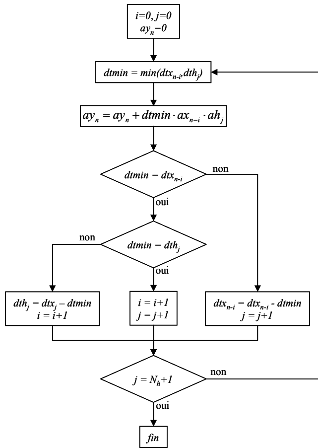
Figure 60 : Organigramme du produit de convolution asynchrone d'ordre 0
