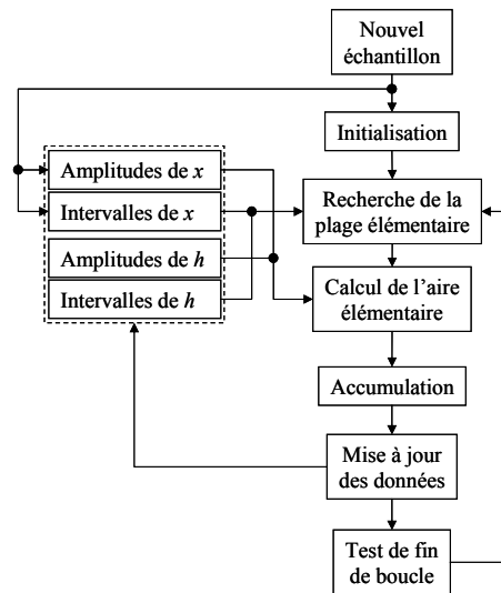
Figure 59 : Organigramme générique de l'algorithme itératif
