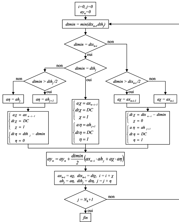
Figure 63 : Organigramme du produit de convolution asynchrone d'ordre 0.5s
