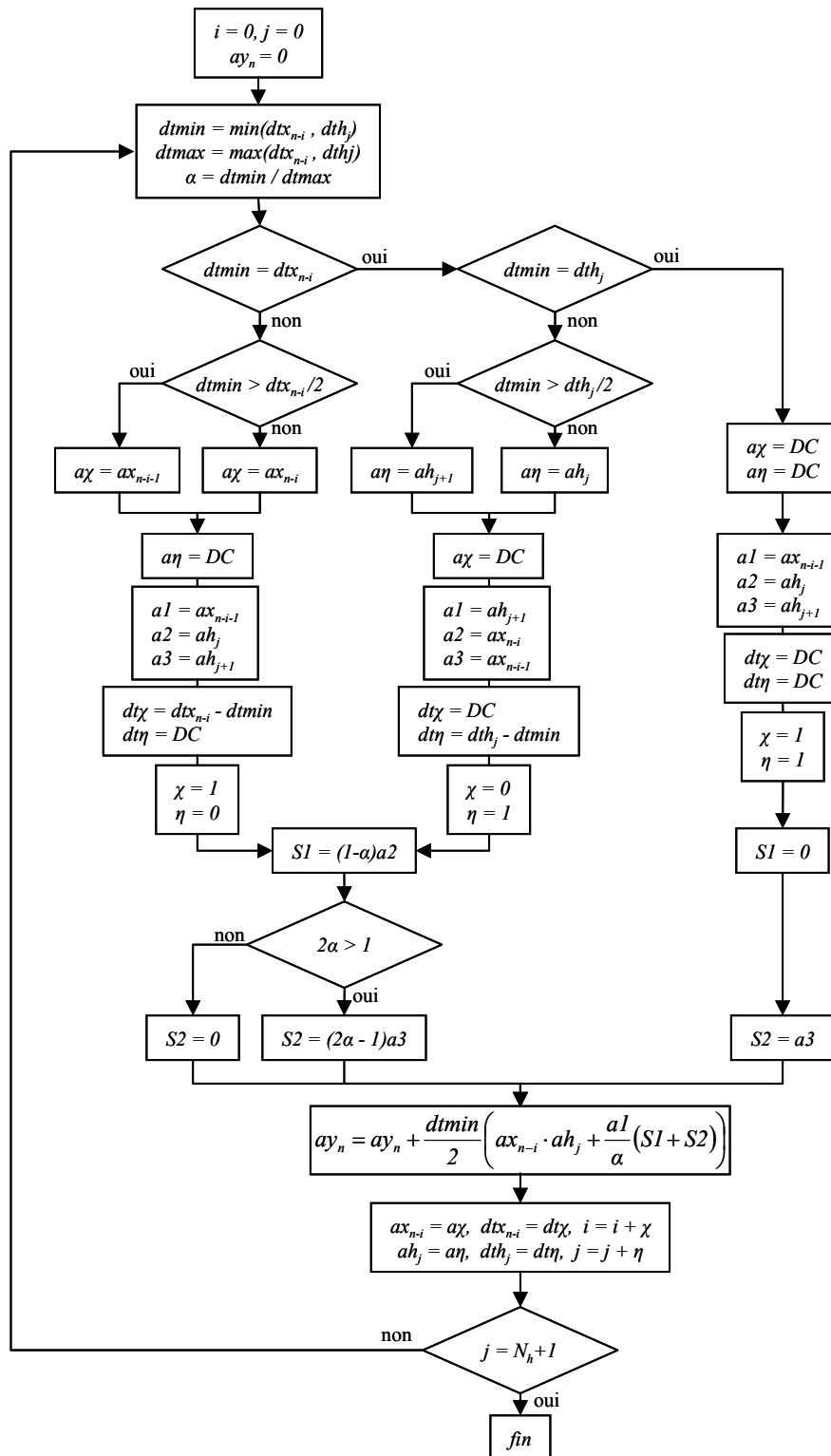
Figure 65 : Organigramme du produit de convolution asynchrone d'ordre 0.5c
