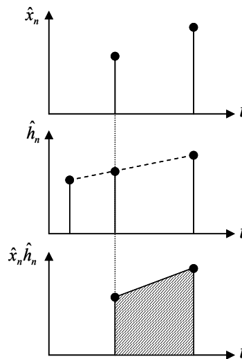
Figure 68 : Produit de convolution asynchrone d'ordre 1s
