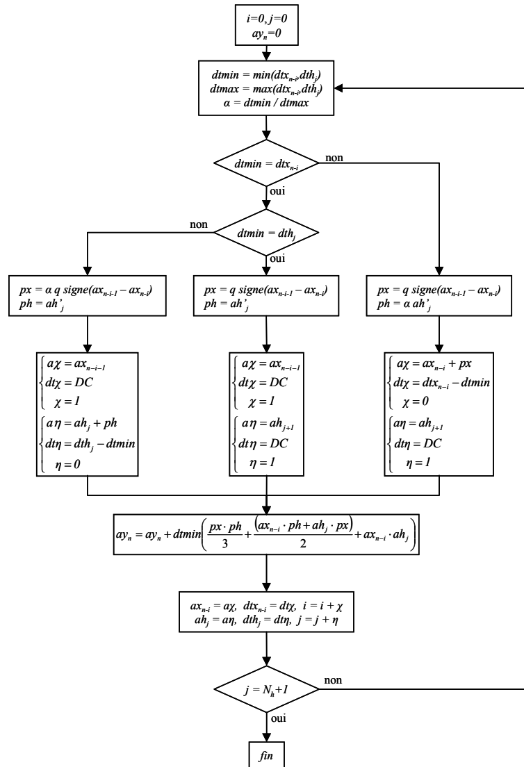
Figure 71 : Organigramme du produit de convolution asynchrone d'ordre 1c
