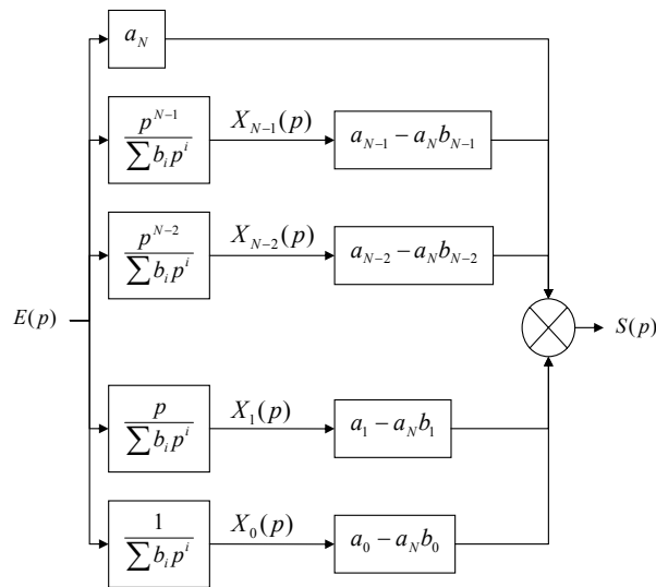
Figure 84 : Représentation dans l'espace d'état d'un filtre analogique
