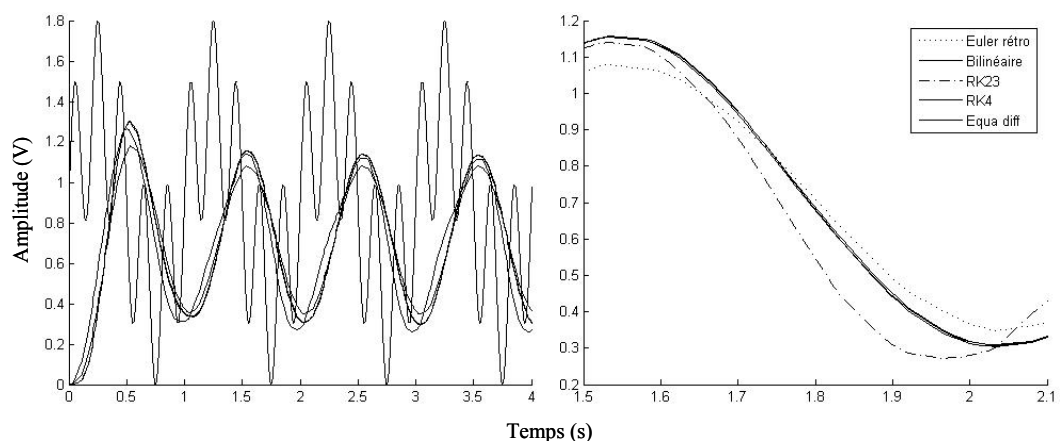
Figure 95 : Filtre de Chebyshev d'ordre 4 (plan large et zoom)
