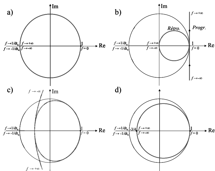
Figure 91 : Projection de l'axe imaginaire du plan complexe analogique par les transformations des méthodes bilinéaire (a), d'Euler rétrograde et progressive (b), Runge-Kutta d'ordre 4 (c) et RK23 (d)
