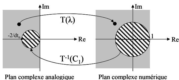
Figure 86 : Transformation du demi-plan gauche pour la méthode d'Euler progressive
