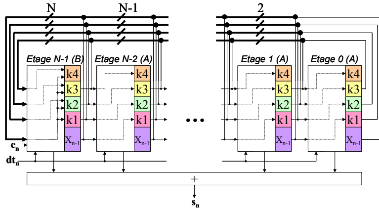
Figure 101 : Structure cascaded d'un filtre RII utilisant le schéma de Runge-Kutta d'ordre 4
