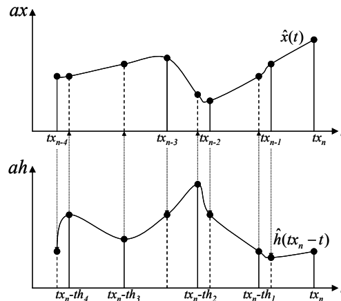
Figure 56 : Echantillonnage des points manquants par interpolation
