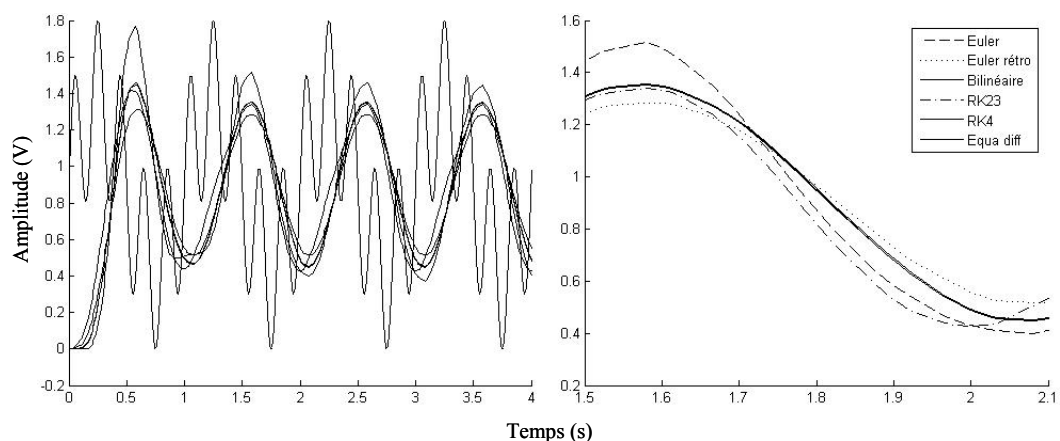
Figure 94 : Filtre de Butterworth d'ordre 6 (plan large et zoom)
