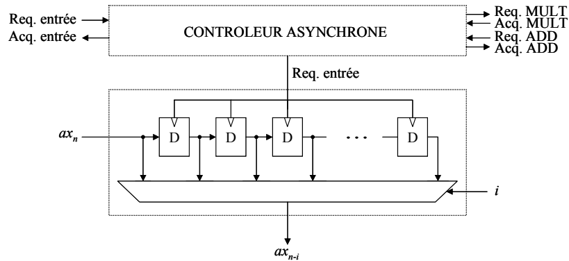
Figure 81 : Architecture du bloc RD ax : registre à décalage des amplitudes du signal d'entrée
