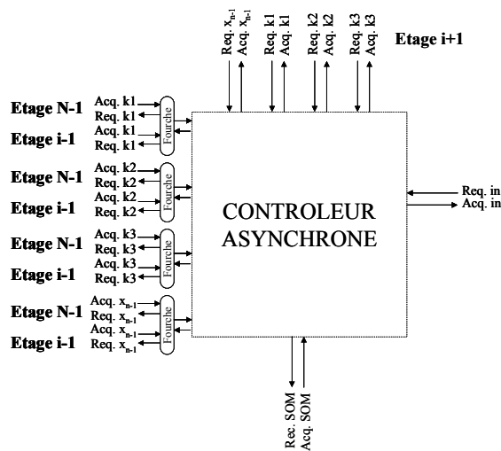
Figure 103 : Contrôleur asynchrone de la structure A utilisé par le schéma de Runge-Kutta d'ordre 4
