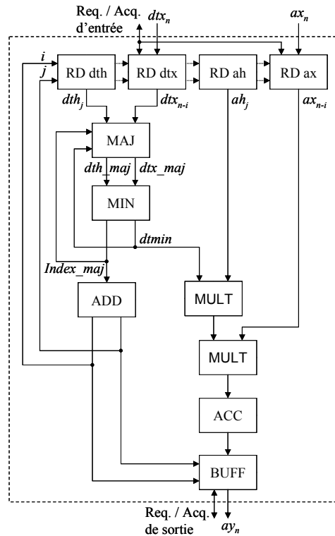
Figure 80 : Structure itérative d'un filtre RIF dans le cas non uniforme
