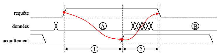
Figure 6 : Protocole à deux phases
