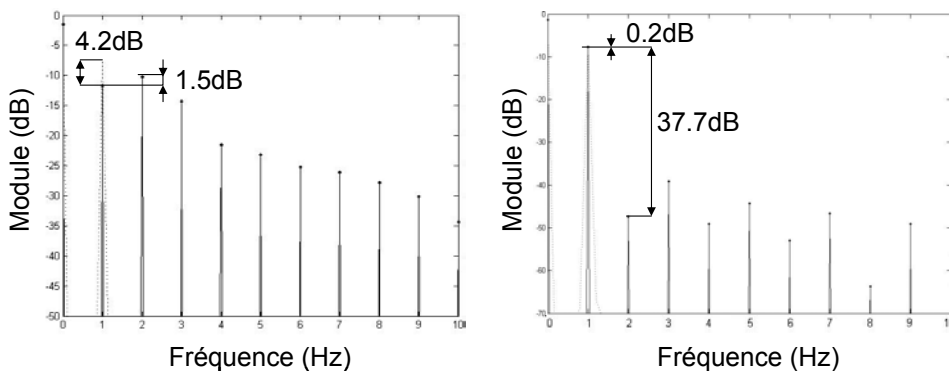
Figure 49 : Comparaison entre les spectres obtenus par GDFT (à gauche) et par TF du signal reconstruit à l'ordre 0 (à droite)
