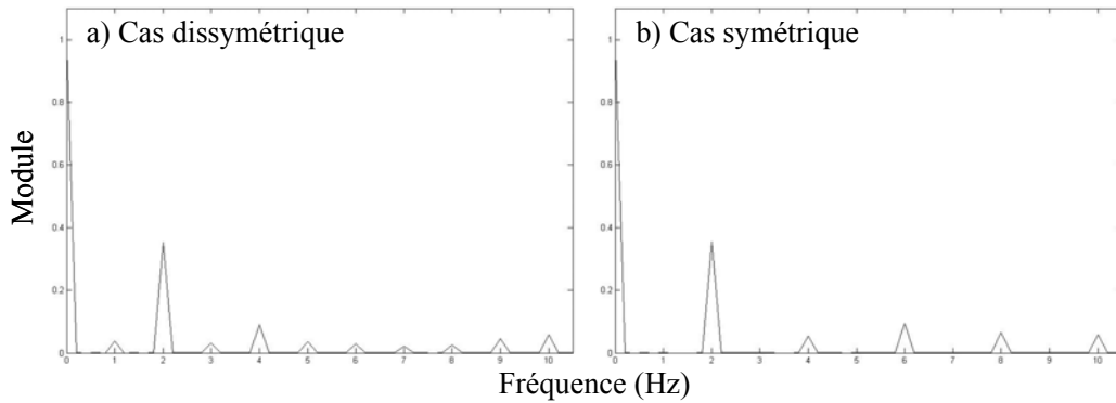
Figure 25 : Schémas d'échantillonnage de signaux sinusoïdaux
