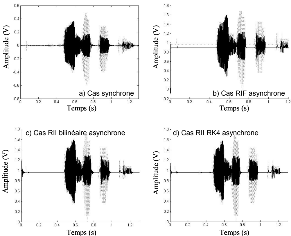
Figure 108 : Filtrage numérique d'un signal de parole échantillonné non uniformément par traversée de niveaux
