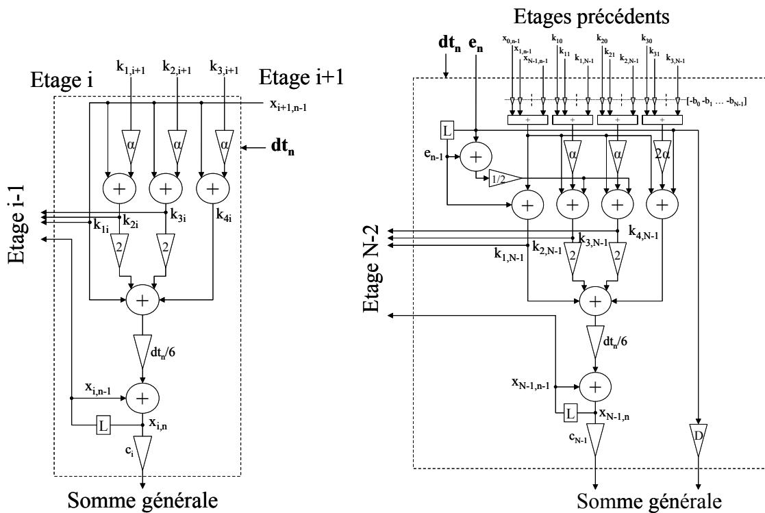
Figure 102 : Structures A et B utilisées par le schéma de Runge-Kutta d'ordre 4
