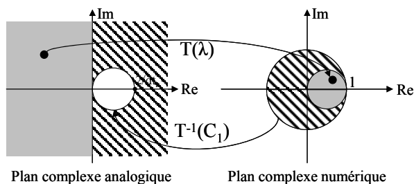
Figure 85 : Transformation du demi-plan gauche avec la méthode d'Euler rétrograde
