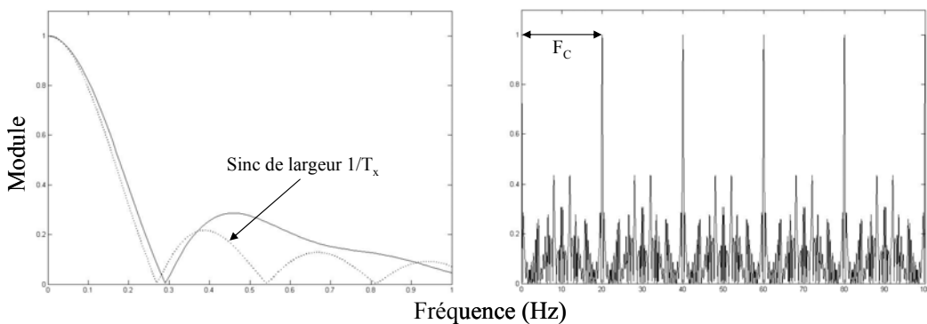
Figure 34 : Schéma d'échantillonnage normalisé d'un signal impulsionnel
