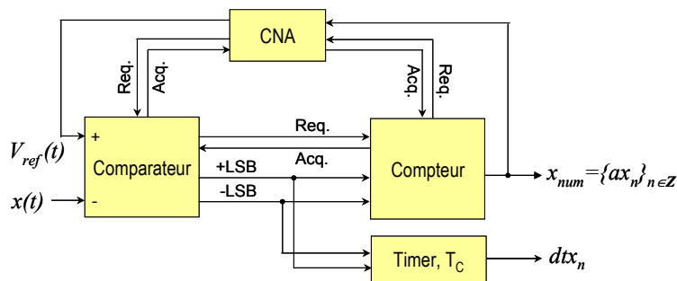
Figure 13 : Boucle de conversion asynchrone
