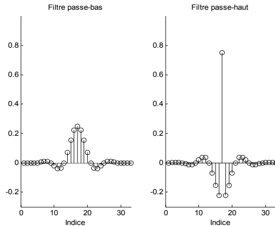
Figure 77 : Réponses impulsionnelles des filtres passe-bas et passe-haut
