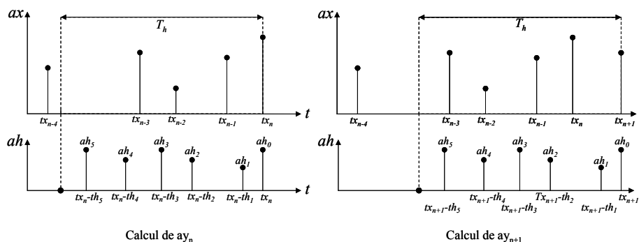
Figure 55 : Synchronisation des signaux à l'initialisation d'un calcul
