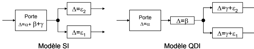
Figure 12 : Equivalence entre les circuits SI et QDI
