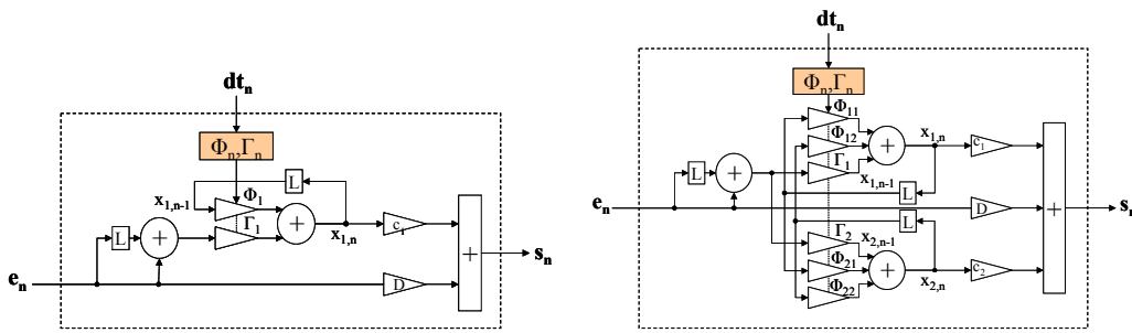
Figure 100 : Structures du 1 er ordre et du 2 ème ordre utilisant la méthode bilinéaire
