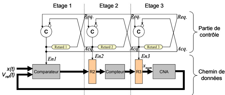
Figure 15 : Schéma fonctionnel asynchrone du CANA
