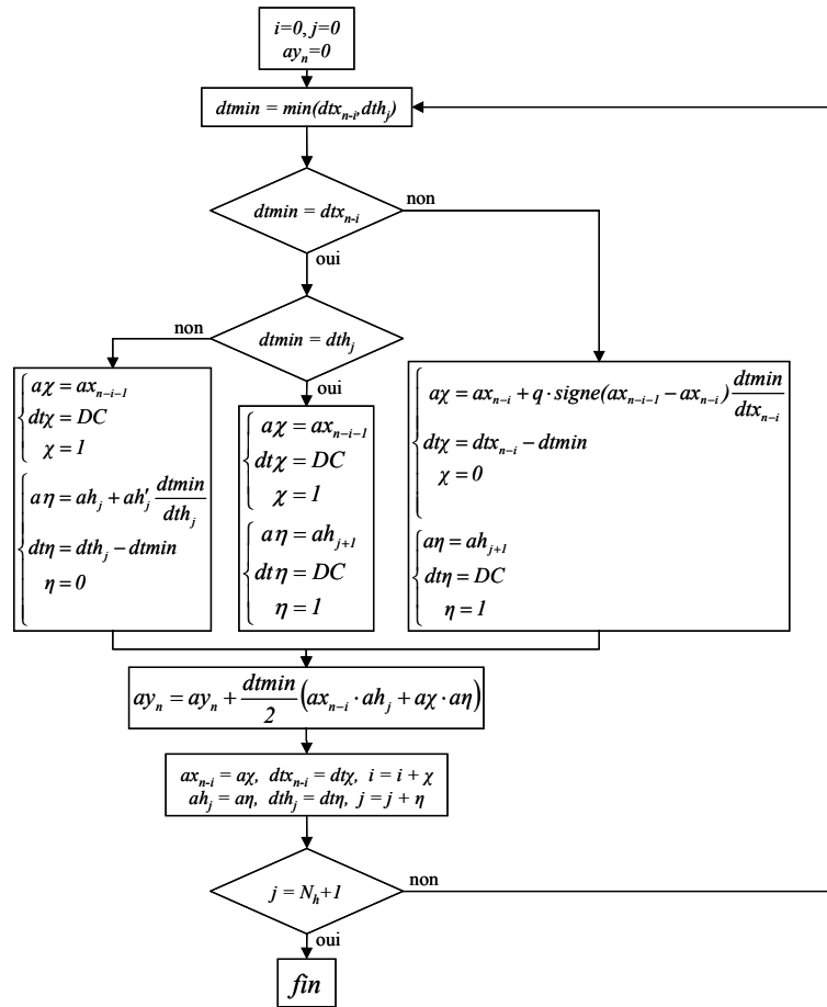
Figure 69 : Organigramme du produit de convolution asynchrone d'ordre 1s
