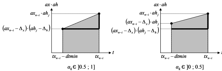
Figure 66 : Etude du pire cas de l'ordre 0.5s
