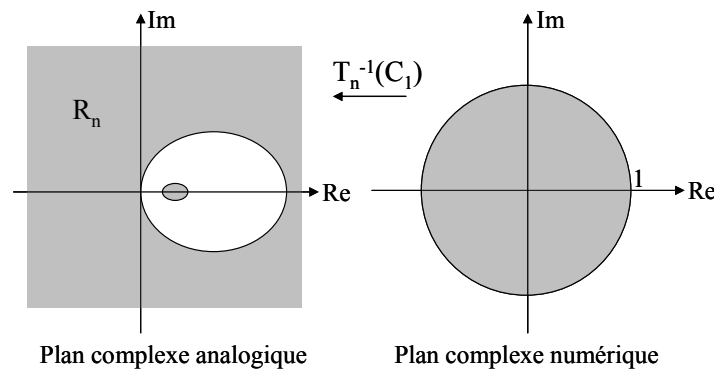
Figure 90 : Transformation inverse du cercle unité pour la méthode de Runge-Kutta d'ordre 3 à 2 étages
