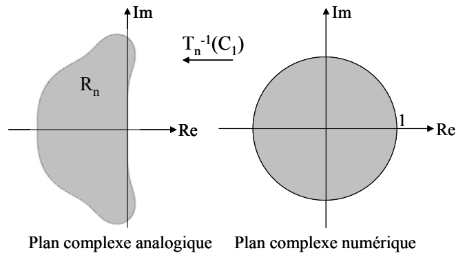
Figure 89 : Transformation inverse du cercle unité pour la méthode Runge-Kutta d'ordre 4
