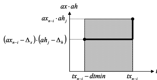
Figure 61 : Etude du pire cas de l'ordre 0
