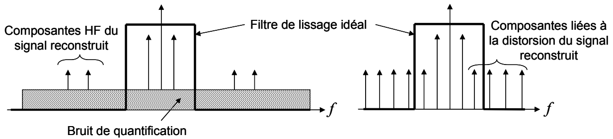
Figure 52 : Effet du lissage d'un signal reconstruit par bloqueur d'ordre 0 dans le cas régulier (à gauche) et dans le cas non uniforme par traversée de niveaux (à droite)
