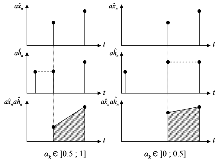
Figure 62 : Produit de convolution asynchrone d'ordre 0.5s
