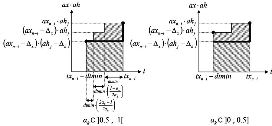
Figure 67 : Etude du pire cas de l'ordre 0.5c
