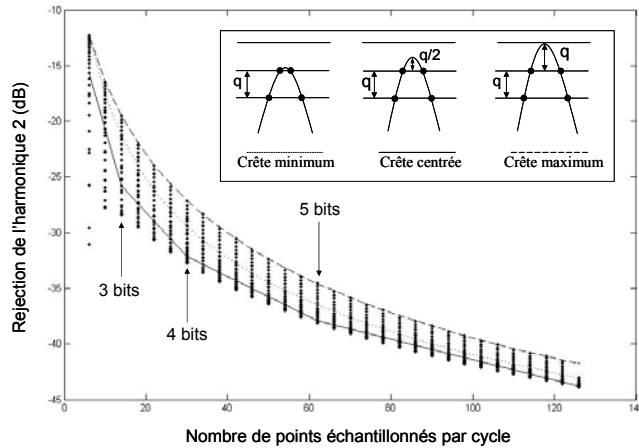
Figure 51 : Taux de rejection de l'harmonique 2 en fonction du nombre de points échantillonnés par cycle d'un signal sinusoïdal
