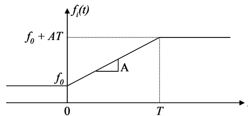
Figure 43 : Fréquence instantanée d'une modulation linéaire de fréquence
