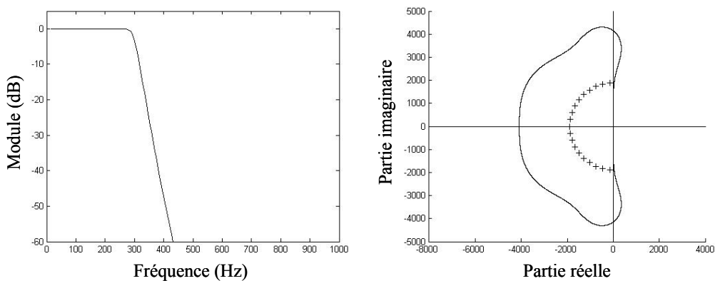
Figure 107 : Réponse en fréquence (à gauche) et pôles (à droite) du filtre RII
