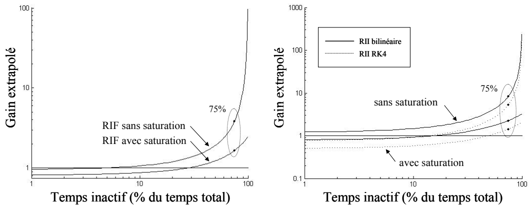
Figure 113 : Gains extrapolés en fonction de l'activité du signal de parole présenté dans notre exemple pour les différents filtres
