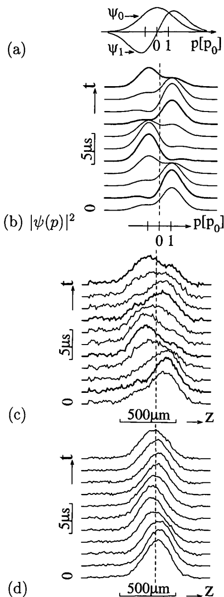
FIG. 5.3 – Evolution de la distribution en impulsion (c) d’une superposition des niveaux vibrationnels |n = 0\rangle et |n = 1\rangle avec des poids égaux et (d) d’un état cohérent à très faible nombre vibrationnel moyen ( \langle n \rangle = 0.08 ). Les courbes sont les coupes verticales d’images prises après 8 ms de temps de vol. Le temps t d’évolution dans le piège (qui est la durée séparant la fin de l’impulsion Raman et la coupure du piège), nul pour la première coupe, est augmenté de 2\mu\text{s} d’une coupe à l’autre. La figure (b) donne l’évolution de la distribution en vitesse d’une superposition de |n = 0\rangle et |n = 1\rangle avec des poids égaux.
