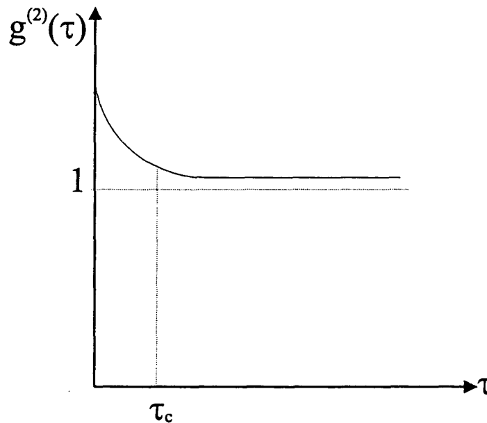
Fig. 15: Temps de cohérence
