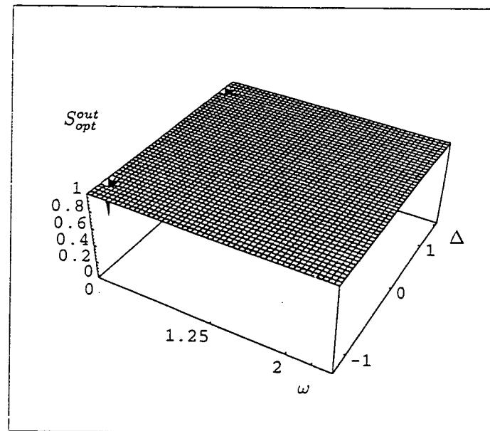
Fig. 42: Spectre de bruit S_{opt}^{out} en fonction du désaccord \Delta et de la fréquence \omega pour g=1 , \gamma = \kappa = \frac{1}{40} , \varepsilon = 100 et \alpha = 10^{-9} (couplage fort)
