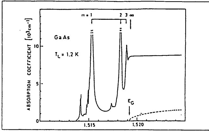
Fig. 6: Spectre d'absorption
