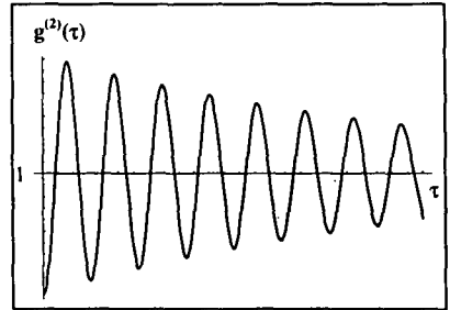
Figure 3: Variations temporelles de la fonction d'autocorrélation g^{(2)}(\tau) à désaccord \phi=0 entre laser et cavité.
