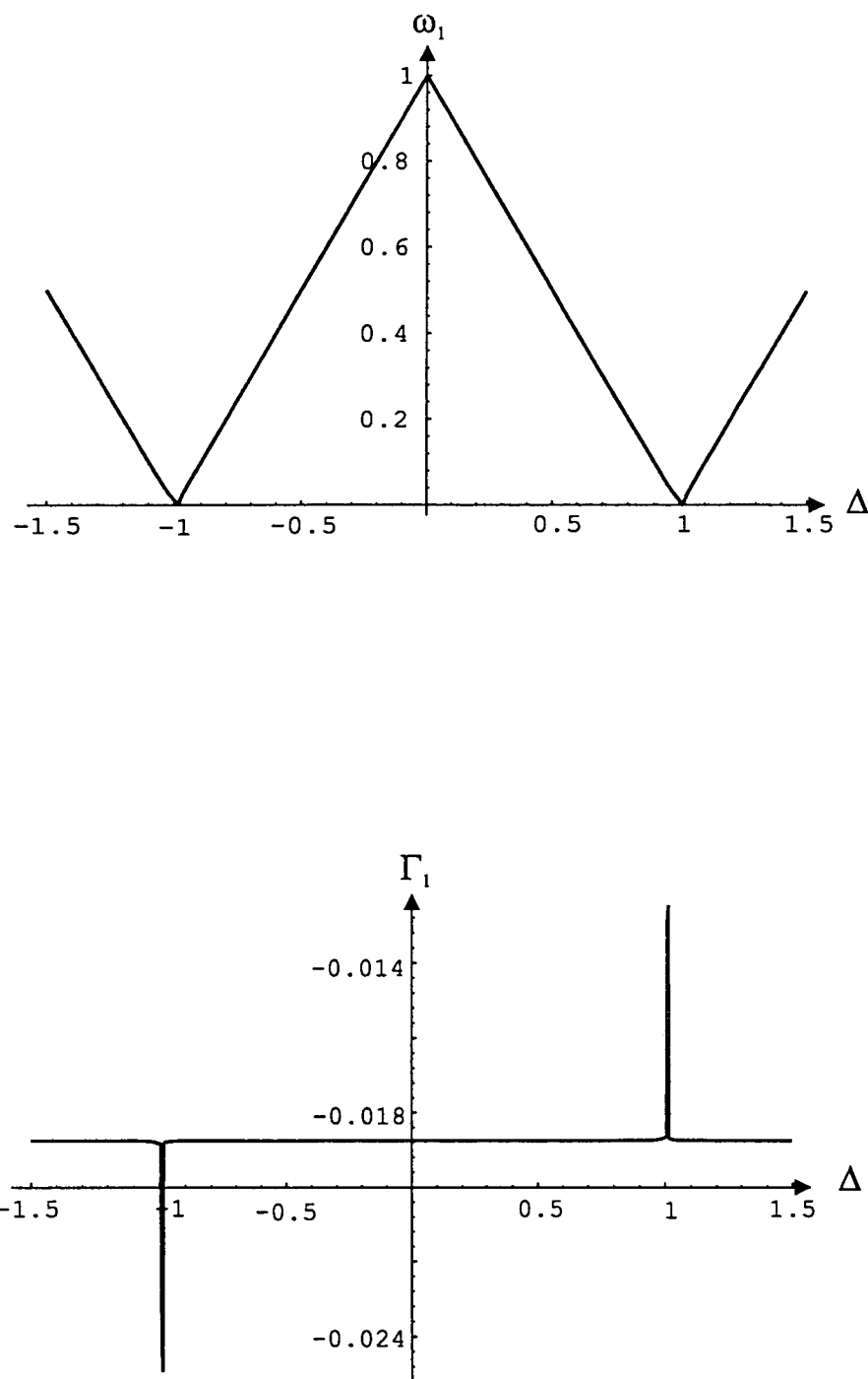
Fig. 66: Fréquence \omega_1 et dissipation \Gamma_1 en fonction de désaccord \Delta avec g=1, \gamma = \kappa = 0.025, \varepsilon = 100 et \alpha = 10^{-9}
