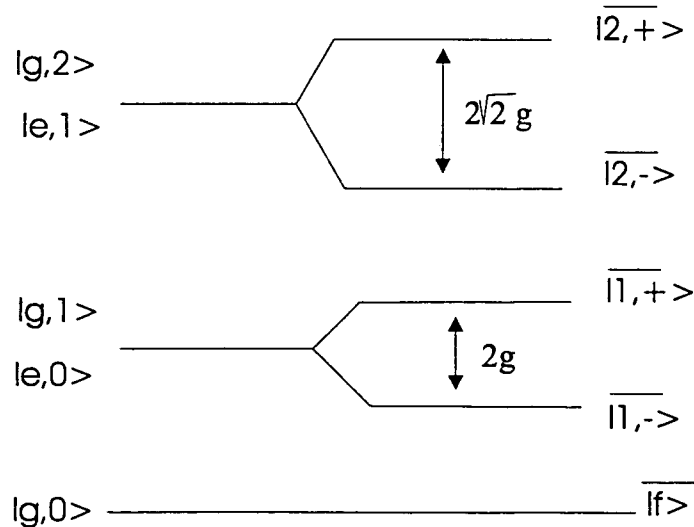
Fig. 3: Les niveaux d'énergies pour les états non couplés et couplés à résonance.
