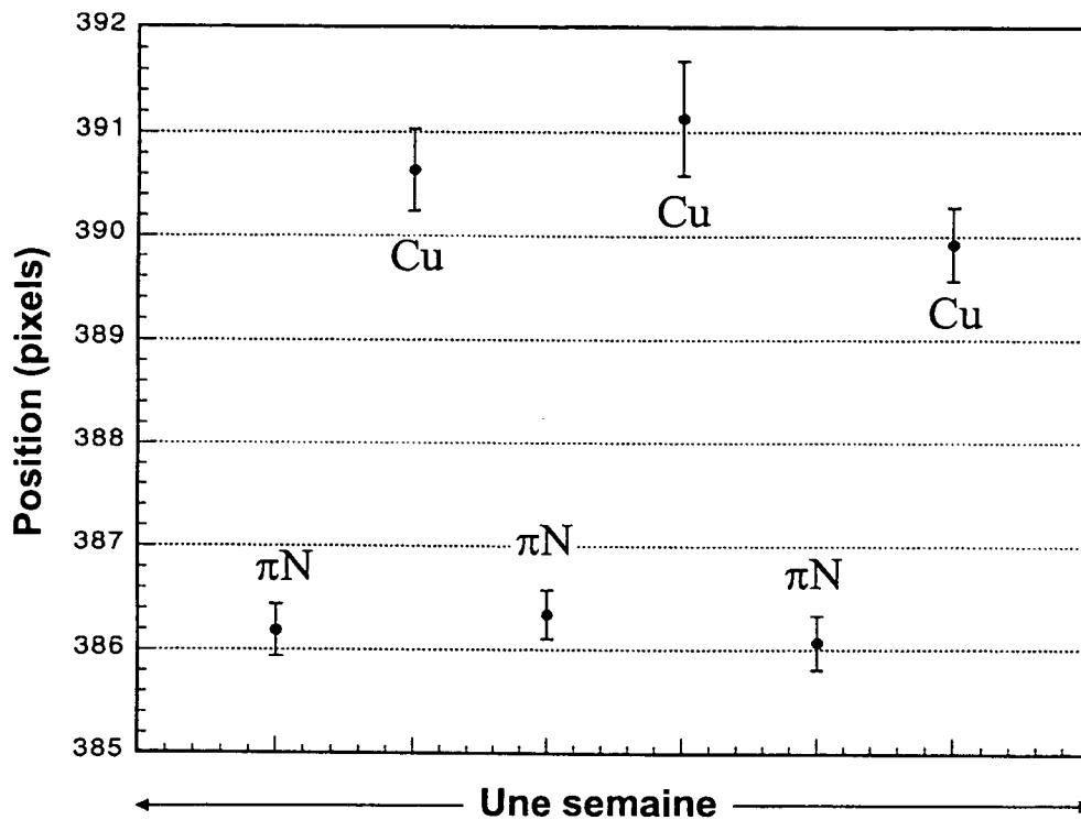
Figure 4-8: Stabilité du spectromètre au cours du temps. Les positions du Cu mettent en évidence une fluctuation moyenne du système de \pm 0.75 pixels au cours d'une semaine. Les positions de l'azote pionique montrent, quant à elles, une faible variation car elles sont moyennées sur un temps de mesure très long.
