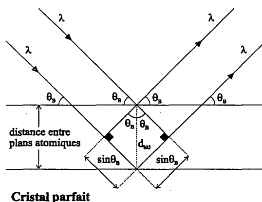
Figure 2-6: Réflexion de Bragg d'un faisceau de rayons-X sur un cristal parfait. Les plans atomiques agissent comme des miroirs, l'angle d'incidence est donc égal à l'angle de réflexion. Une interférence additive apparaît lorsque la différence de marche 2d_{hkl} \sin \theta_B est un multiple entier de la longueur d'onde \lambda .
