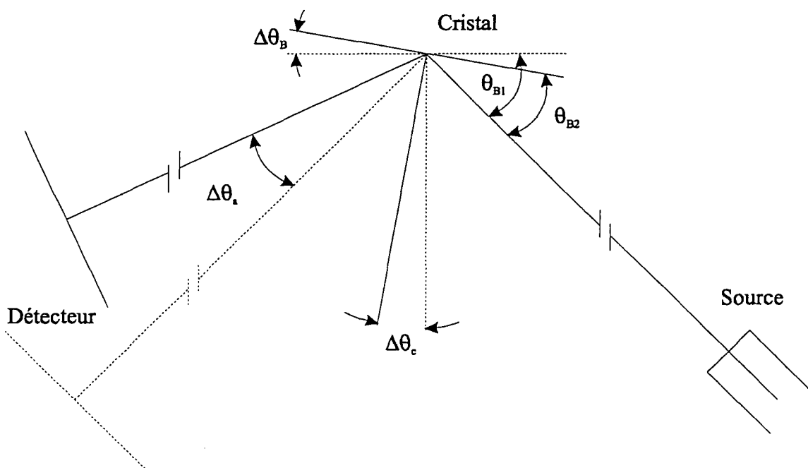
Figure 2-14: Sélection d'un angle du cristal. Si on tourne le cristal de \Delta\theta_B , le bras du spectromètre doit être tourné de 2\Delta\theta_B .
