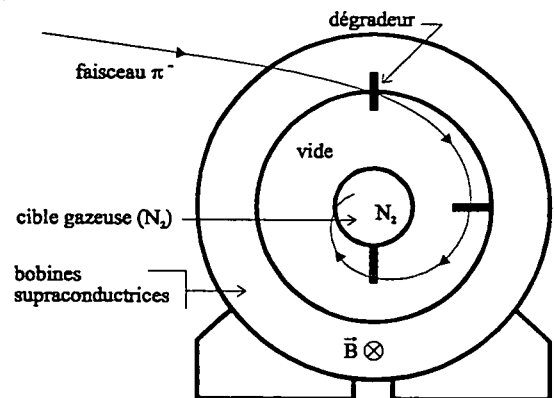
Figure 2-4: Suite aux collisions qu'elles subissent dans le gaz, et sous l'action du champ magnétique, les particules décrivent une spirale qui les amène au centre de la cible gazeuse où elles sont stoppées.
