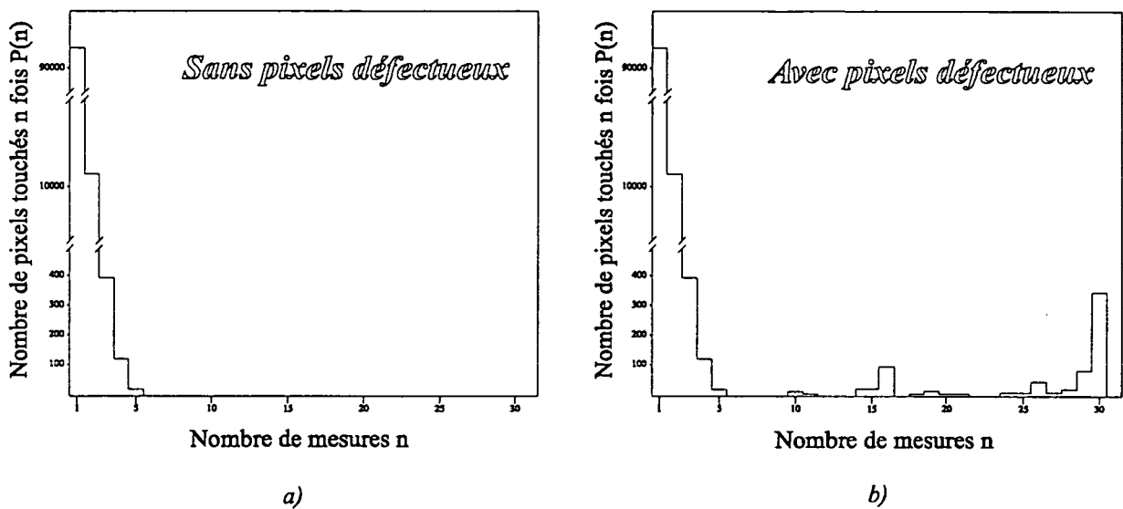
Figure 3-13: a) Histogramme d'un CCD sans pixels défectueux. Le nombre de pixels touchés n fois décroît au fur et à mesure que n croît, et s'annule à partir d'une certaine valeur de n . b) Histogramme d'un CCD ayant des pixels défectueux. On remarque la présence de pixels qui restent activés un grand nombre de fois. Ces pixels sont défectueux car ils ne peuvent pas être dus à des rayons-X.
