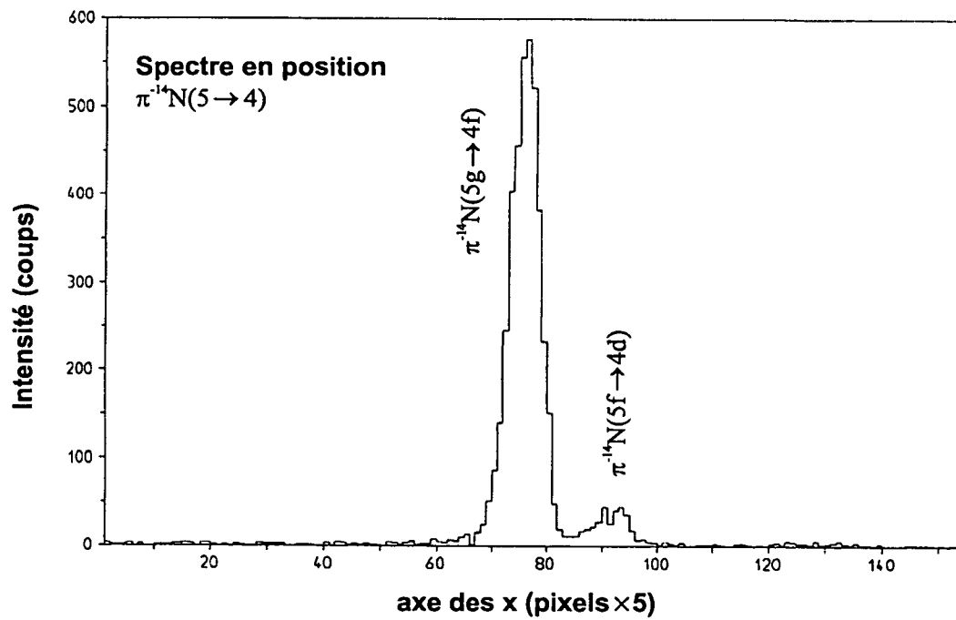
Figure 3-8: Spectre en position de l'azote pionique obtenu par projection du spectre de dispersion sur l'axe horizontal du CCD (après rejet du bruit de fond). Ce spectre nous permet de déterminer la position de la raie sur le détecteur, et de remonter à l'énergie de la transition d'après la géométrie du spectromètre.
