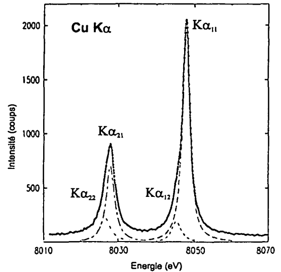
Figure 4-3: La raie K\alpha du cuivre montrant les transitions satellites comme étudiées par le modèle de Deutsch et al. [54].
