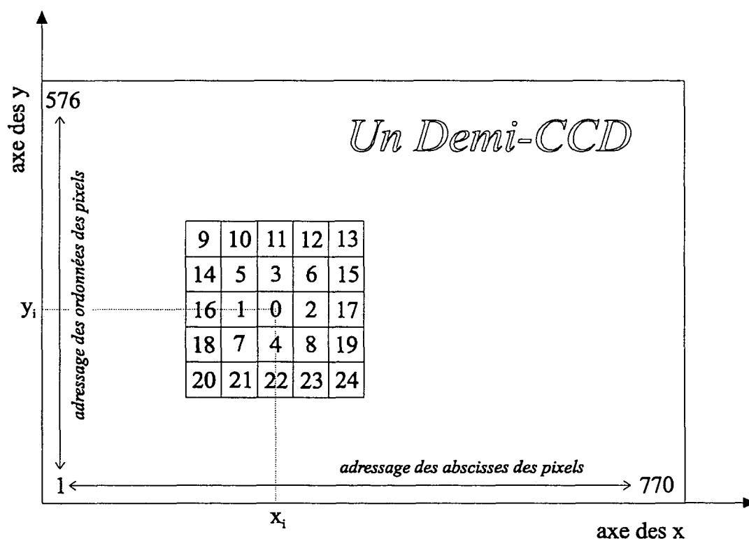
Figure 3-5: Numérotation et positionnement des pixels environnants. Les 24 pixels entourant le pixel central noté 0, sont répartis selon 2 cadres, interne (pixels 1 à 8) et externe (pixel 9 à 24). Chaque pixel est repéré par son abscisse et son ordonnée; les 2 axes horizontal et vertical du CCD sont pris pour les axes x et y respectivement.
