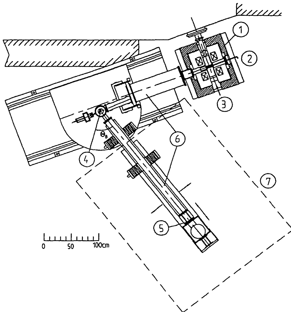
Figure 4-4: Installation de la trappe cyclotron et du spectromètre de Bragg dans la zone \pi\text{E5} au PSI. 1: Trappe cyclotron. 2: Chambre cible. 3: Tube à rayons-X. 4: Cristal courbe. 5: Détecteur CCD. 6: Tubes à vide. 7: Contour de l'enceinte de blindage.
