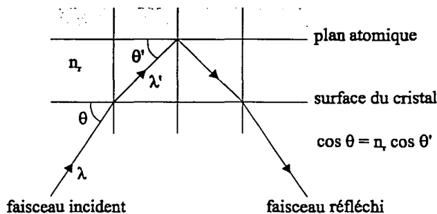
Figure 3-18: Effet de l'indice de réfraction. Le faisceau incident est dévié de la normale à l'entrée du cristal sous l'influence de l'indice de réfraction relatif entre le milieu extérieur et le cristal. Comme conséquence, l'angle de Bragg se trouve modifié à l'intérieur du cristal.
