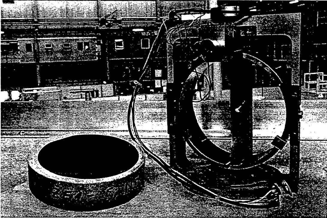
Figure 2-9: Un cristal courbe de silicium avec son support.
