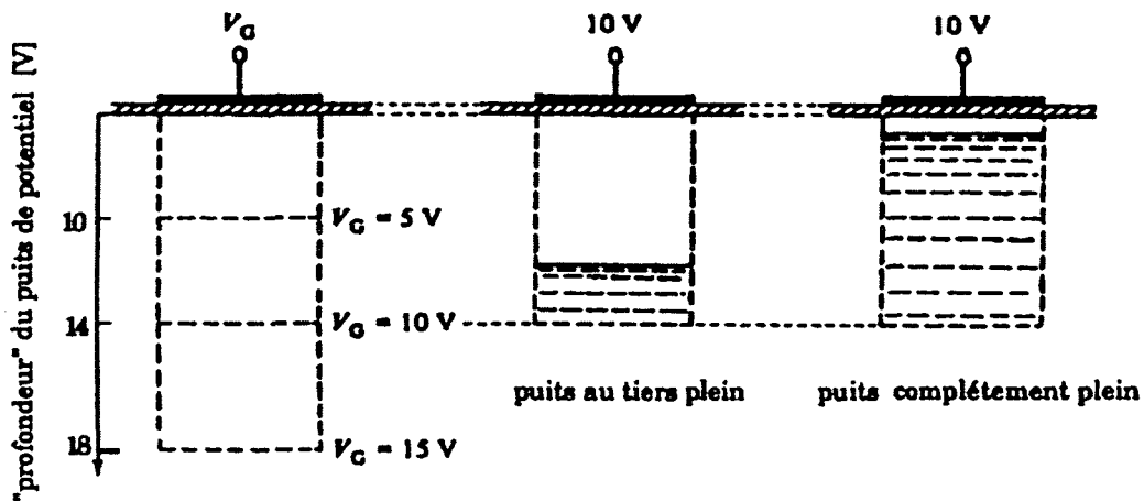
Figure 2-18: Le modèle hydraulique du puits de potentiel. La profondeur du puits est définie par V_G . Le stockage d'une charge est assimilable au remplissage du puits par un liquide.
