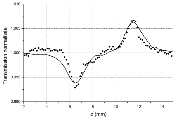
Homosil (épaisseur = 7.4 mm )
