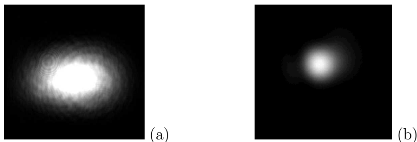
FIG. 4.2 – Faisceau issu du système MIRA900 + PULSE SWITCH. Intensité du faisceau au niveau du coupleur de sortie (a) et champ lointain (après filtrage) dans le plan focal d'une lentille de focale 100 mm (b).
