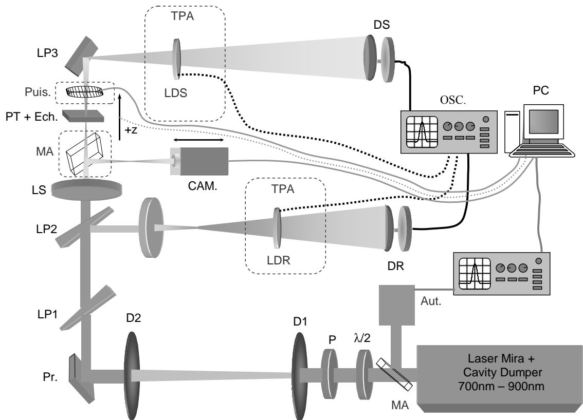
FIG. 4.27 – Montage expérimental dans le cas du système MIRA + PULSE SWITCH. Les éléments des montages sont : FIR : filtre coupe visible, \lambda/2 : lame demi-onde à 1064 nm, P : polariseur, 2\omega : cristal de KTP et filtre coupe IR (pour les mesures à 532), L1, L2, D1, D2 : lentilles et diaphragmes pour filtrage spatial, Pr. : prisme, LP1, LP2, LP3 : lames prismatiques, Pyro. : pyromètre, Puis. : mesureur de puissance, LR, LS : lentilles ( f' = 100 mm) sur support X-Y à vis micrométriques, Aut. : autocorrélateur, MA : miroir amovible pour l'étude du faisceau où du profil temporel, CAM. : camera CCD et objectif sur platine de translation, PT : platine de translation motorisée commandée par PC, Ech. : échantillon mobile, DR, DS : photodiodes de la voie de référence et de la voie signal placées après un trou et un diffuseur, LDR, LDS : photodiodes larges de la voie de référence et de la voie signal pour la mesure d'absorption à deux photons, PDR : photodiode rapide pour la mesure du profil temporel, OSC. : oscilloscope, PC : ordinateur
