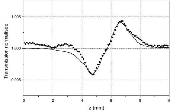
Herasil (épaisseur = 3 mm )
