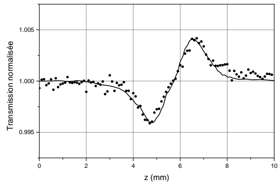
Suprasil (épaisseur = 4 mm )
