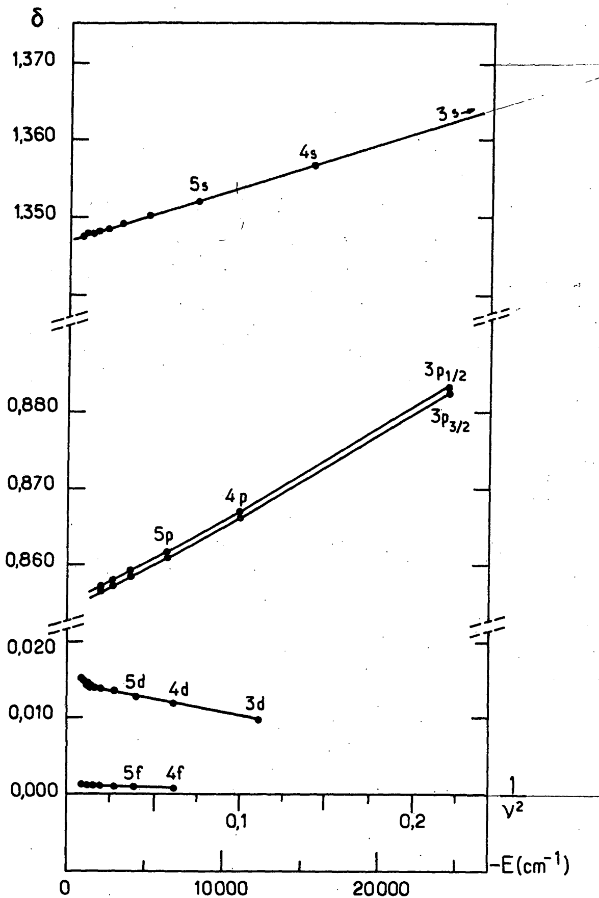
Fig.13 - Variation des défauts quantiques dans le sodium ( 36 )
