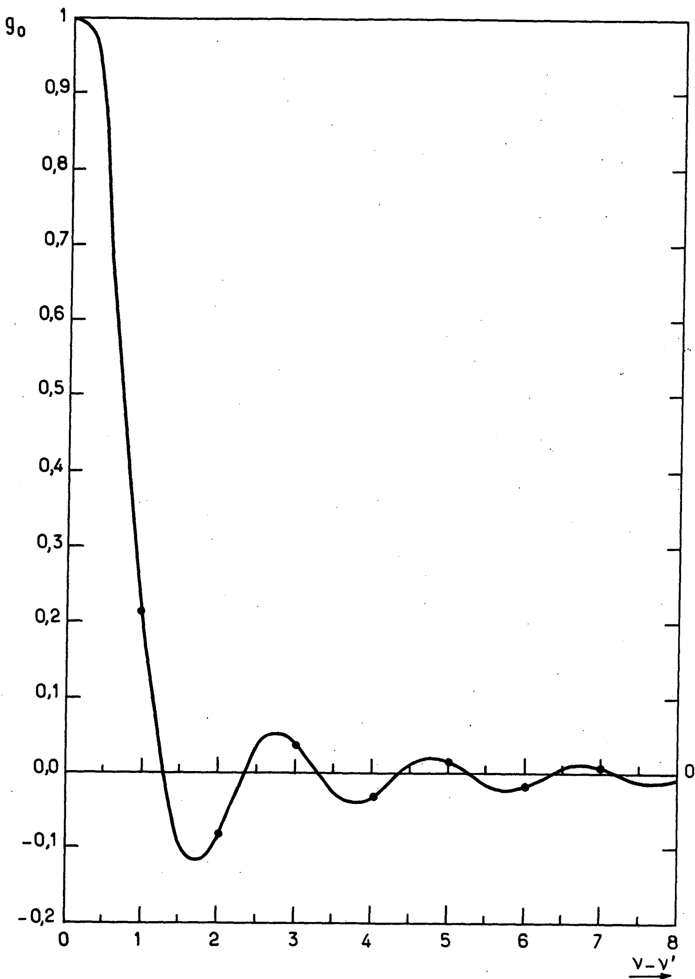
Fig.15. fonction g_0(v-v') (réf. (50))
