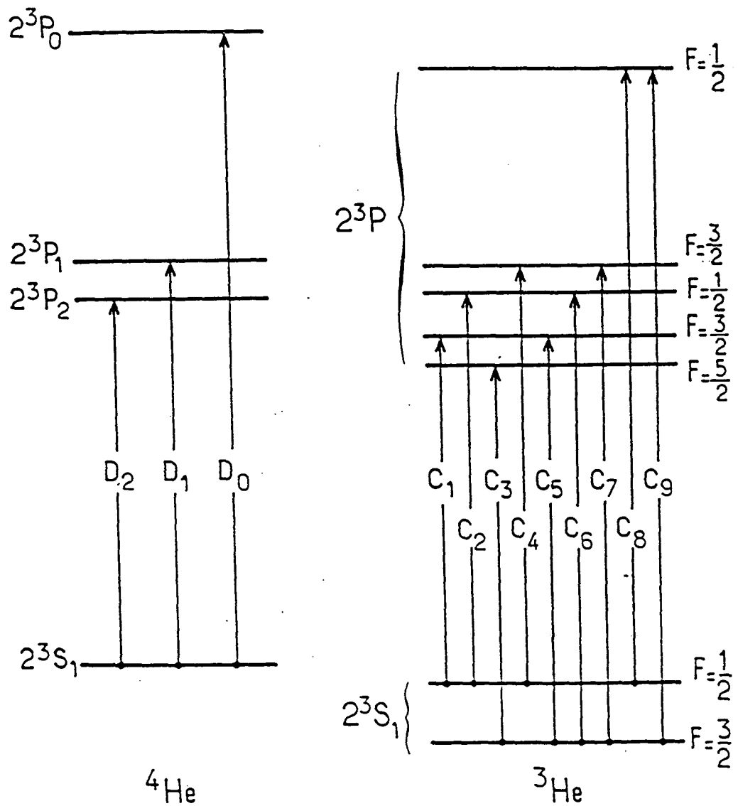
Figure P-2 Niveaux 2^3S et 2^3P de l'hélium : structure fine et transition D_0, D_1, D_2 pour l'hélium-4. Structure hyperfine et transition C_1 à C_9 pour l'hélium-3.
