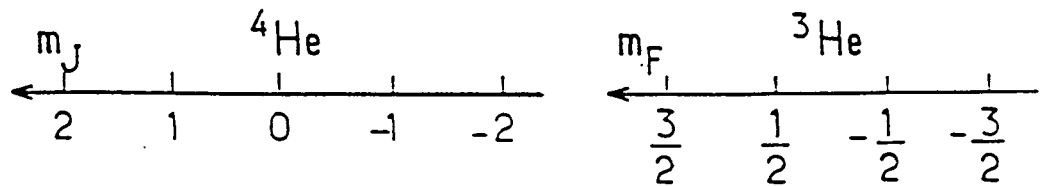
Figure II-2 Structure et noms des sous-niveaux 2^3S et 2^3P de l'hélium-4 (à gauche) et de l'hélium-3 (à droite).
