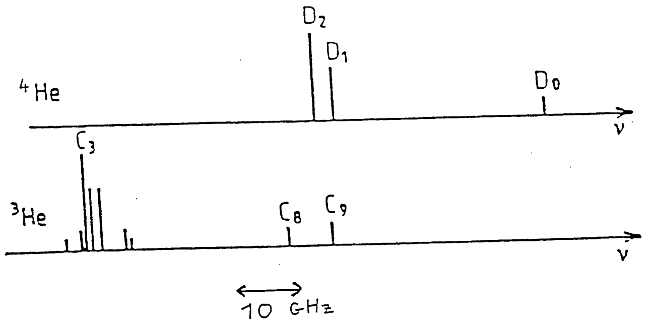
Figure P-3 Position relative des raies de l'hélium-4 (en haut) et de l'hélium-3 (en bas).
