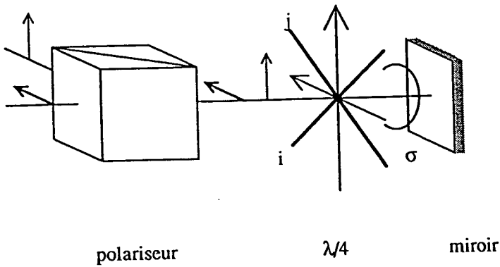
Figures 7 et 8 : Détermination des axes neutres d'une lame \lambda/4 .
