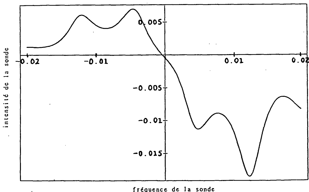
Figure 22 : Courbe théorique sur la transition F = 4/F' = 5 , calculée pour une seule paire de faisceaux pièges et une sonde faisant un angle de 25^\circ avec elle. L'intensité correspond à une pulsation de Rabi par onde \Omega^2/\Gamma^2 = 3/2 et le désaccord est \delta = -20\Gamma . Il apparaît deux composantes dont le rapport des distances au centre est 2,7.
