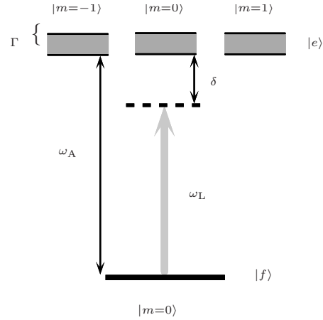
FIG. A.1 – La transition utilisée.
