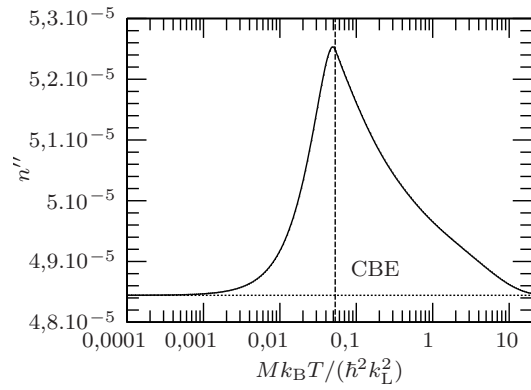
(b) Partie imaginaire, \delta = 10\Gamma .
