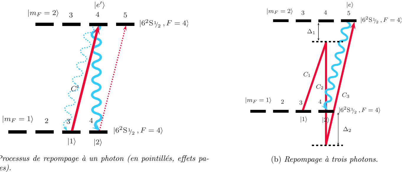
FIG. 3.23 – Deux méthodes de repompage pour le refroidissement Raman dans un piège magnétostatique.
