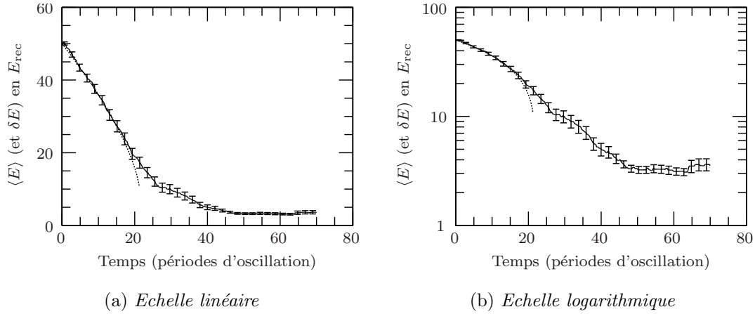
FIG. 2.15 – Evolution de l'énergie moyenne des atomes en fonction du temps. En pointillés, le premier modèle présenté au paragraphe 2.4.a (éq. (2.65)). En trait plein, simulation de Monte-Carlo 1D, avec 100 atomes (les barres verticales matérialisent 2\delta E , où \delta E est l'écart-type). Les paramètres sont \bar{\Omega}/2 = 0,03k v_{\text{rec}} , \bar{\Gamma}/2 = 0,1k v_{\text{rec}} , v_{\text{rés}} = 3v_{\text{rec}} , \eta = 1 , \xi = 0,75 , \omega_x = 133 \text{ rad/s} .
