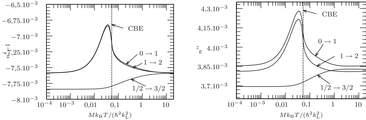
(a) Partie réelle
