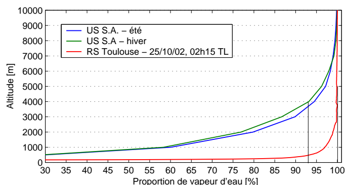
FIG. 3.7 – Distribution cumulative relative de la vapeur d'eau dans la troposphère obtenue à partir des profils de concentration d'azote et de vapeur d'eau issus de l'US Standard Atmosphere (US s.a.) [USSA, 1976], pour l'été (trait bleu) et l'hiver (trait vert), pour une latitude moyenne ( 45^\circ ). A titre de comparaison, un profil calculé à partir d'un radiosondage lâché de Toulouse (25/10/02, 02h15 TL) est tracé (trait rouge).
