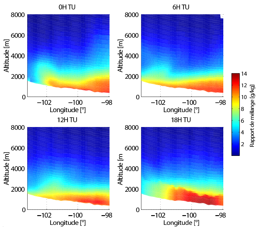
FIG. 6.7 – Rapport de mélange simulé par MM5 le 29 mai 2002 le long d'une coupe verticale est-ouest passant par Homestead pour 4 échéances successives : 0H, 6H, 12H et 18H TU.
