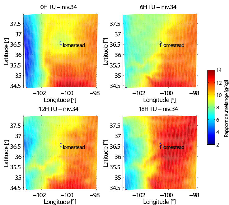
FIG. 6.6 – Rapport de mélange simulé par MM5 le 29 mai 2002 au niveau 34 (~ 500m), pour 4 échéances successives : 0H, 6H, 12H et 18H TU.
