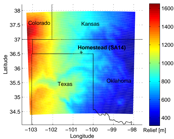
FIG. 6.5 – Relief du domaine de la simulation MM5 pour le cas du 29 mai 2002. La station GPS à Homestead (SA14) est aussi représentée.
