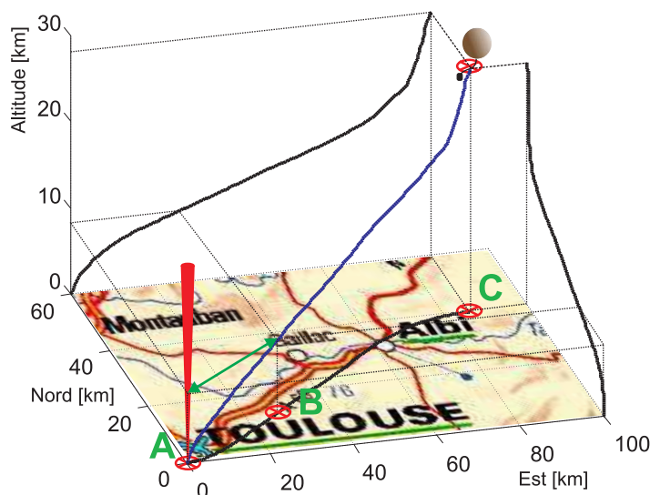
FIG. 5.14 – Trajectoire 3D du radiosondage lâché le 28 octobre 2002 à 00h07 TL de Toulouse (point A ). La comparaison lidar/radiosondage s’effectue jusqu’à \sim 7 km d’altitude (cf. figure 5.11). A cette altitude, le radiosondage se trouve à \sim 30 km à l’est et \sim 10 km au nord (point B ) du volume sondé par le lidar Raman IGN/SA. A son altitude maximale (point C ), le ballon est à \sim 85 km à l’est et \sim 40 km au nord de son point de départ. Cette figure illustre l’intérêt relatif qu’il faut donner aux comparaisons lidar/radiosondage et à la qualité de l’étalonnage ainsi réalisé.
