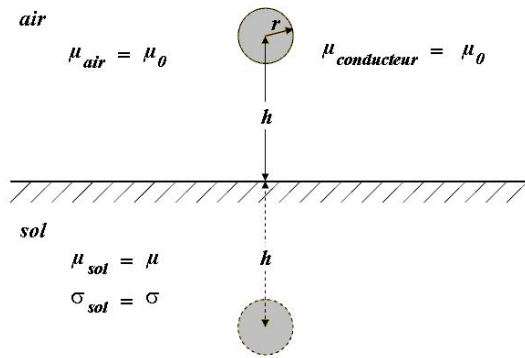
Figure 2-13 : Conducteur cylindrique au dessus d'un sol réel
