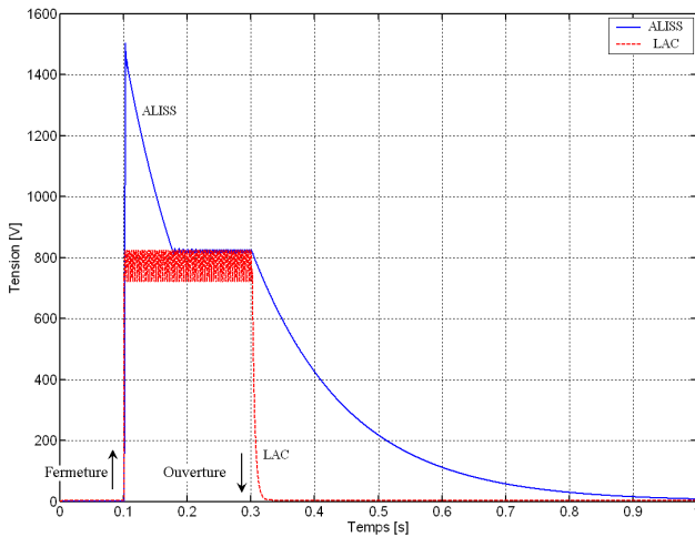
Figure 4-24 : Tension en sortie du disjoncteur de sous-station
