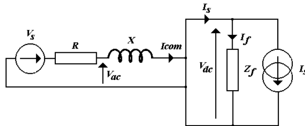
Figure 5-4 : Schéma équivalent, phase (2), régime d'empiètement
