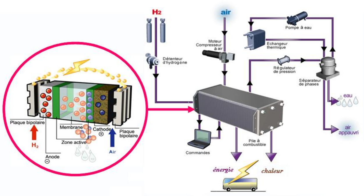
Figure 1-17 : Composants d'un système Pile à Combustible
