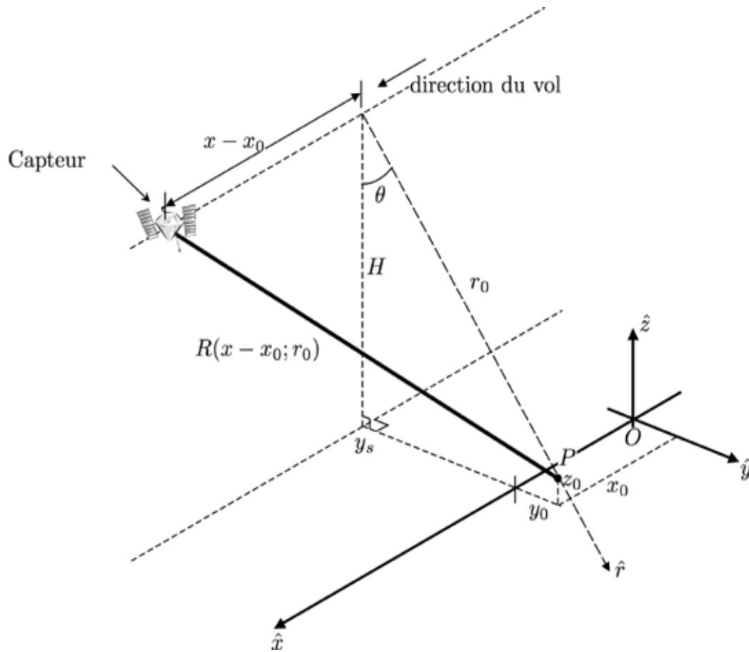
FIG. 1.2 – Géométrie d'une mesure SAR.
