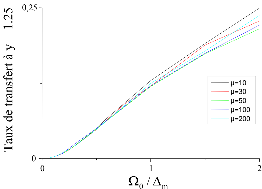
Figure 5.7 : Variation du taux de transfert vers l'état excité en fonction de \Omega_0 / \Delta_m pour un désaccord normalisé y = 1,25 . Les calculs ont été réalisés avec une impulsion CHS symétrique de durée 6\beta^{-1} . La durée de vie de cohérence a été prise égale à T_2 = 8\beta^{-1} .
