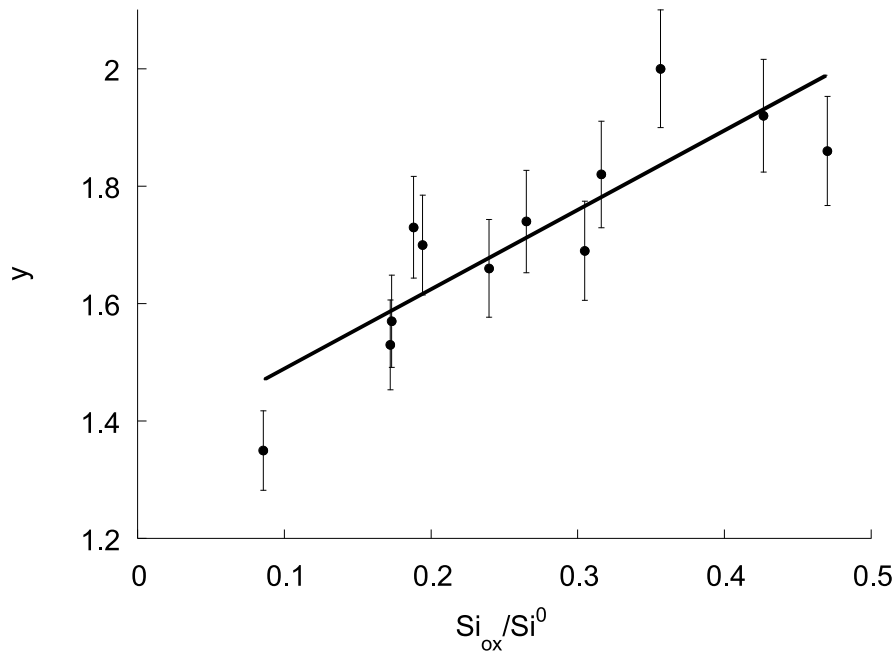
FIG. 4.3 – Evolution de la stœchiométrie de l'oxyde \text{SiO}_y en fonction de la quantité relative de silicium oxydé pour l'ensemble des dépôts réalisés.
